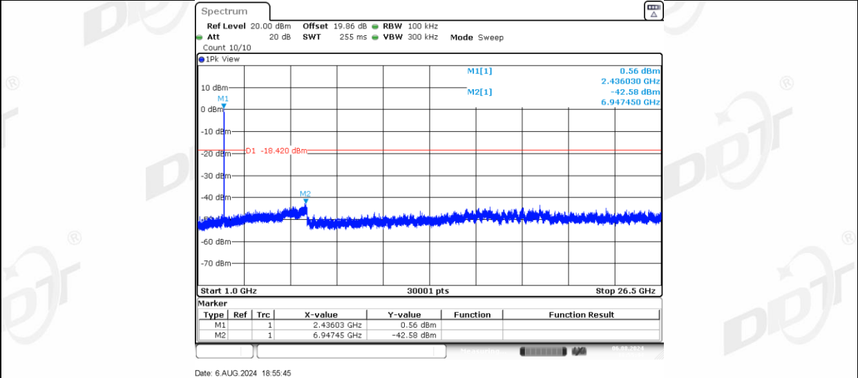
11N20MIMO_Ant-3_2437_0~Reference
