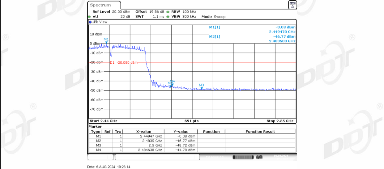
11N40MIMO_Ant-3_High_2452
