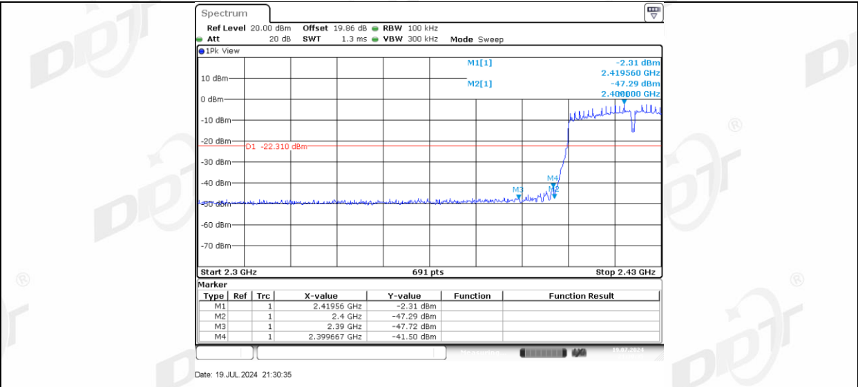
11N40MIMO_Ant-3_Low_2422
