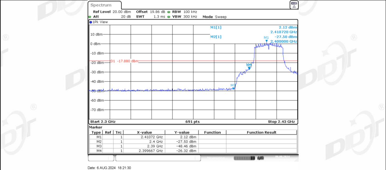
11N20MIMO_Ant-3_Low_2412
