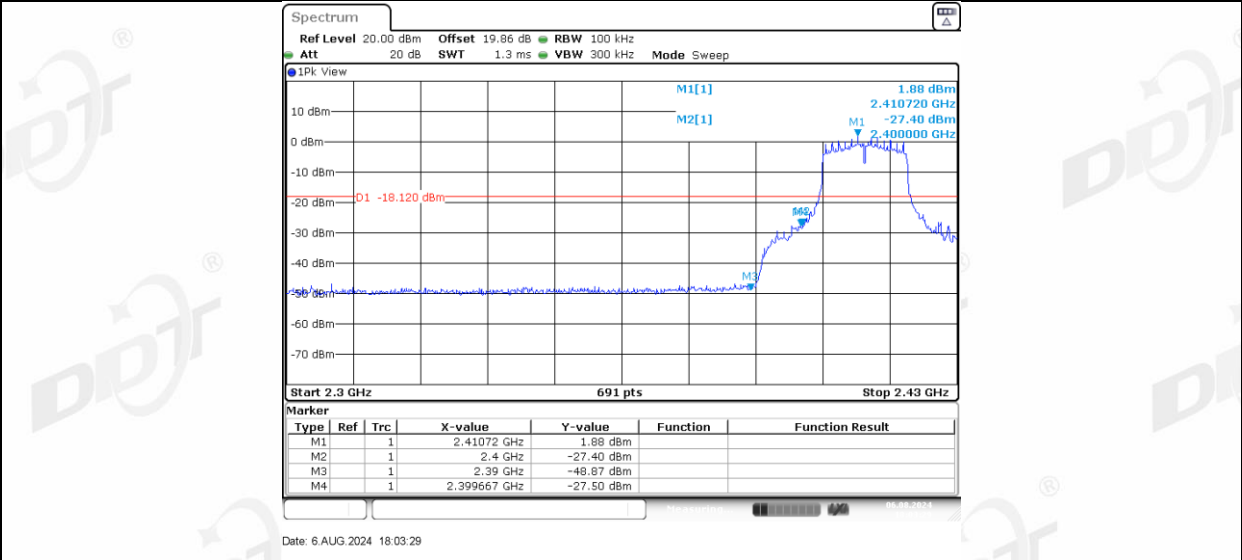
11G-CDD_Ant-3_Low_2412
