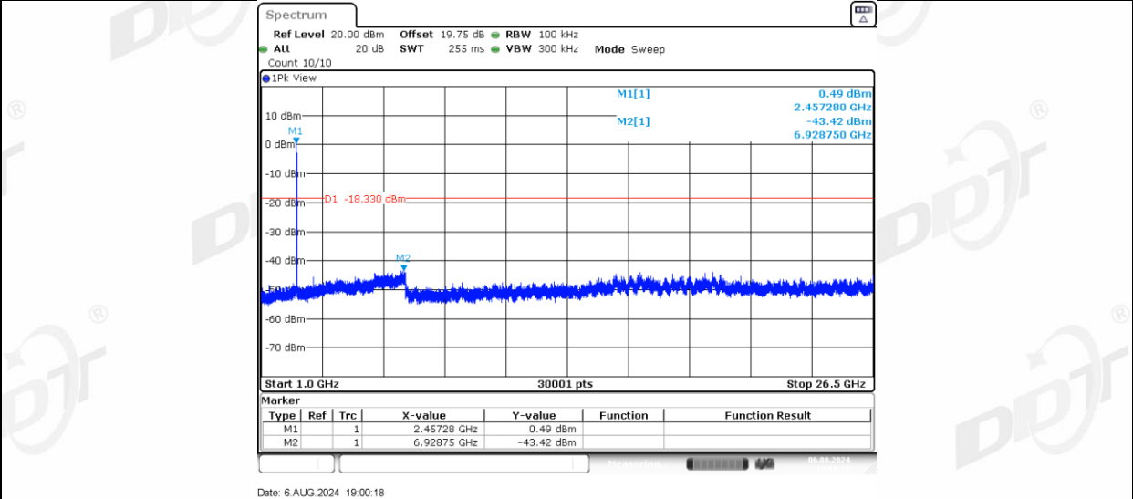
11N20MIMO_Ant-3_2462_0~Reference
