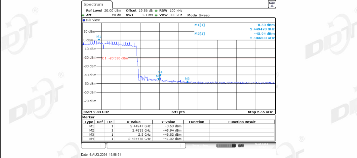
11AX40MIMO_Ant-3_High_2452
