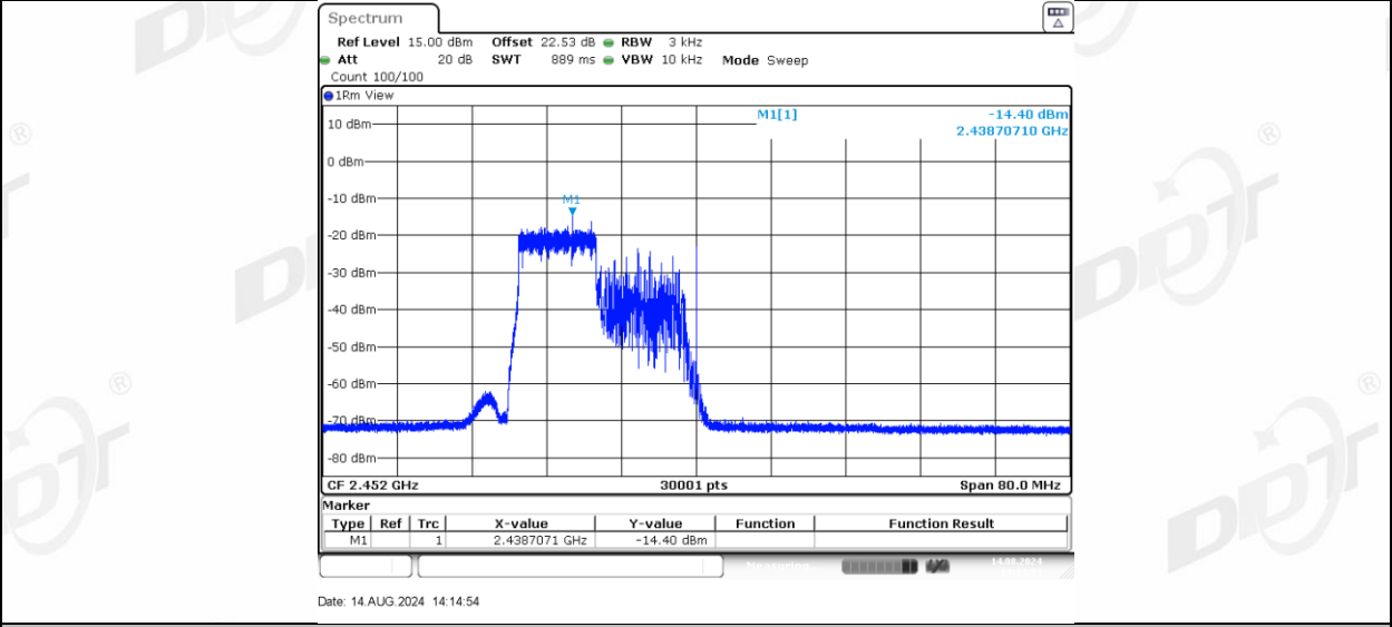
11AX40MIMO_Ant-3_2452_106Tone_RU56
