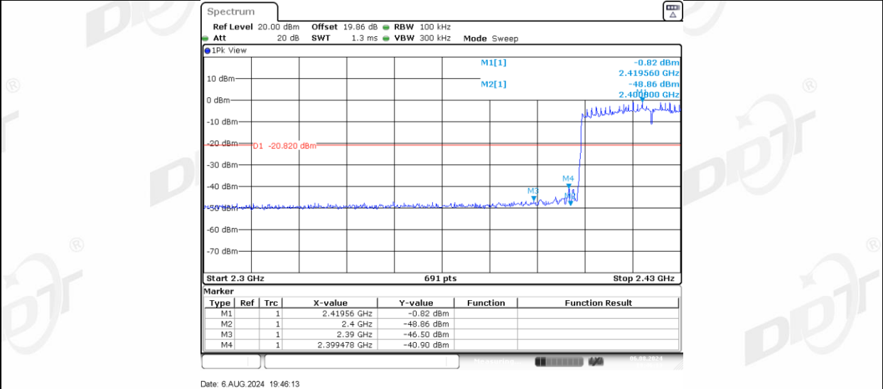
11AX40MIMO_Ant-3_Low_2422
