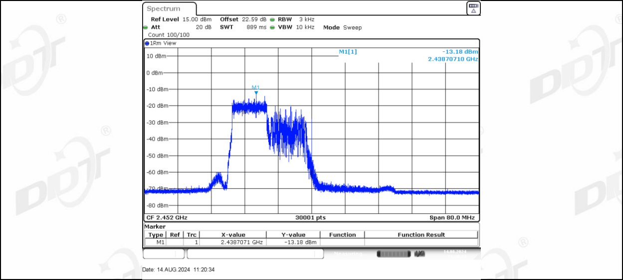
11AX40MIMO_Ant-1_2452_106Tone_RU56
