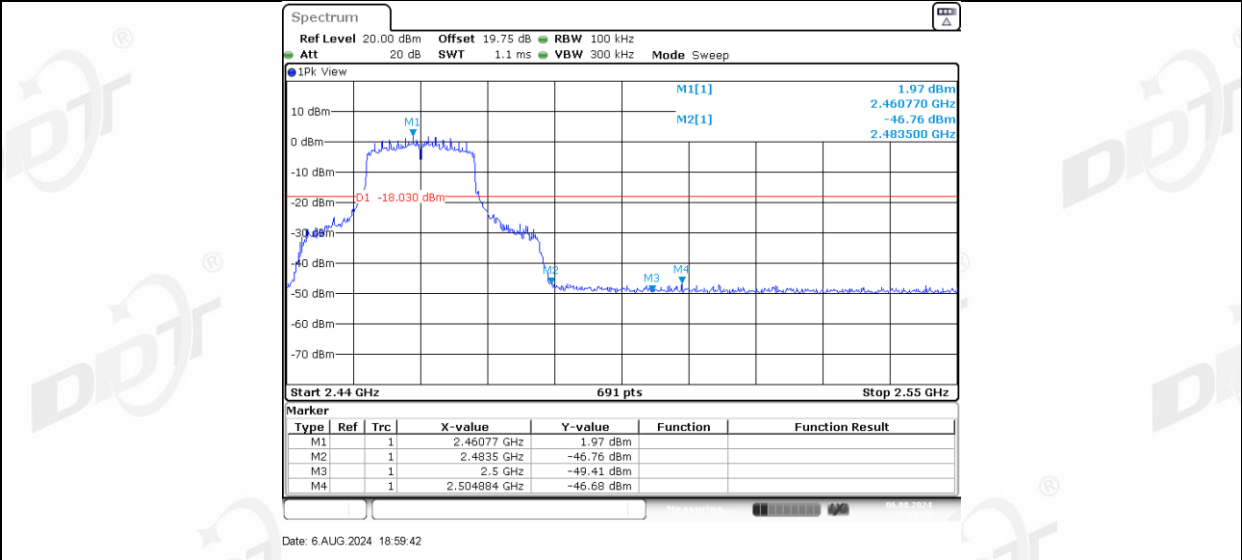
11N20MIMO_Ant-3_High_2462
