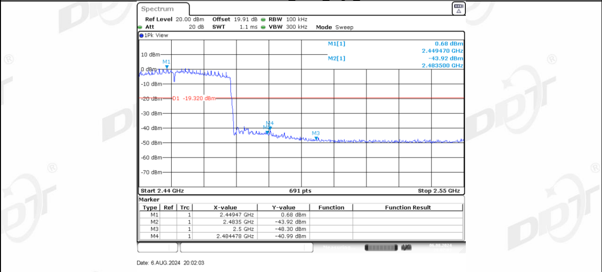
11AX40MIMO_Ant-3_High_2452
