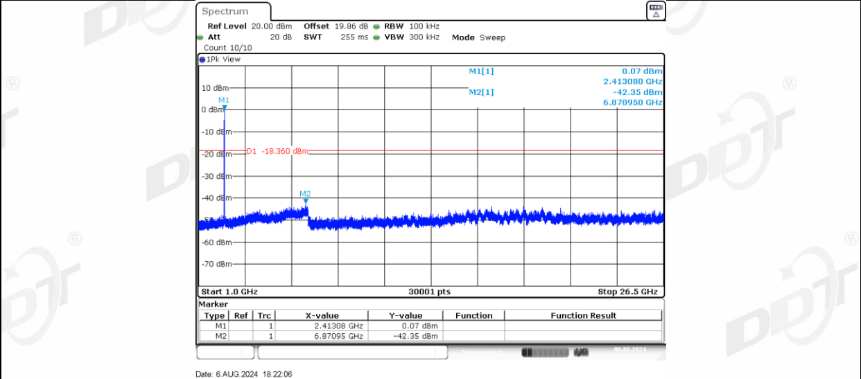
11N20MIMO_Ant-3_2412_0~Reference
