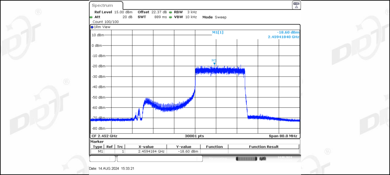
11AX40MIMO_Ant-3_2452_106Tone_RU53
