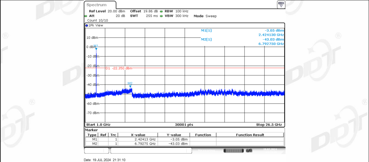
11N40MIMO_Ant-3_2422_0~Reference
