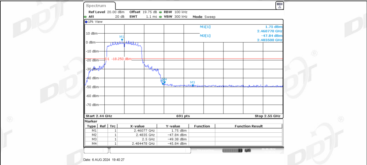
11AX20MIMO_Ant-3_High_2462
