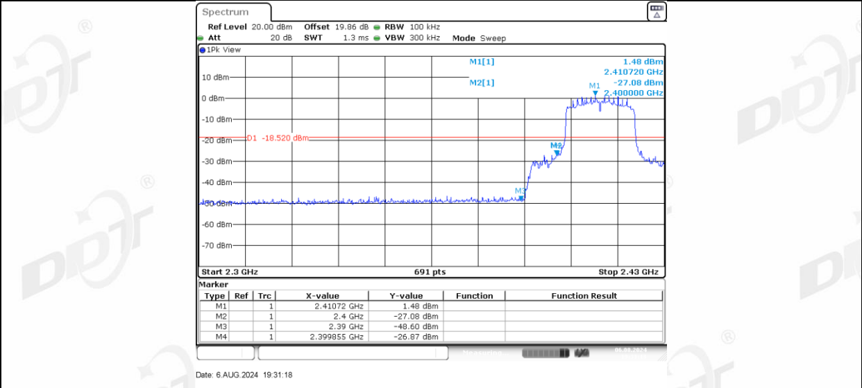
11AX20MIMO Ant-3_Low_2412
