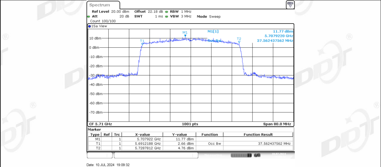
11AX40MIMO_Ant-3_5710
