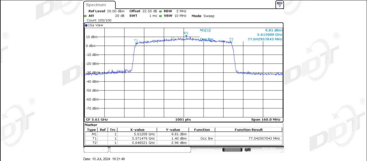
11AX80MIMO_Ant-3_5610
