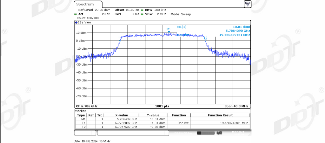
11AX20MIMO_Ant-3_5785
