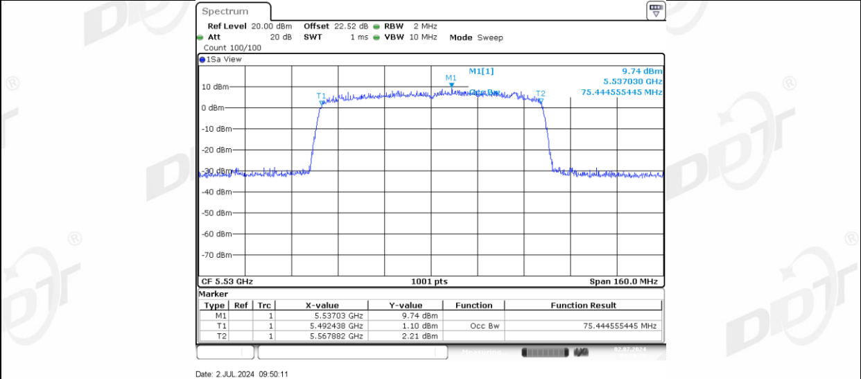
11AC80MIMO_Ant-3_5530
