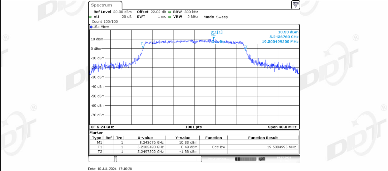
11AX20MIMO_Ant-3_5240
