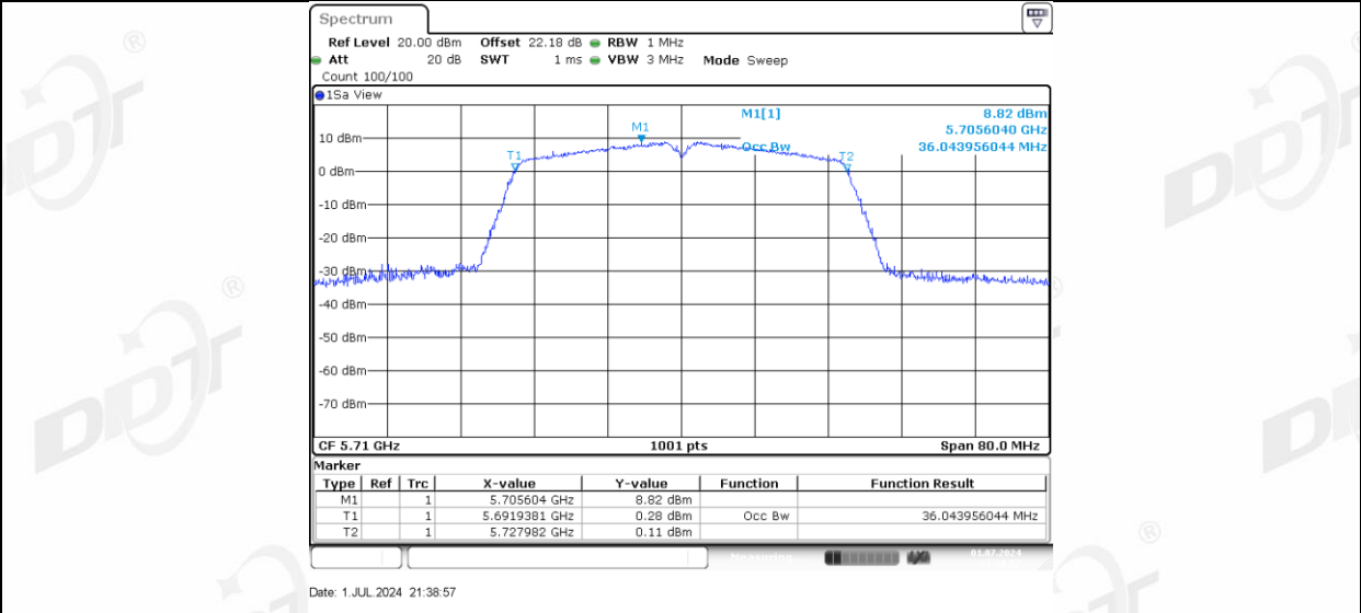
11AC40MIMO_Ant-3_5710
