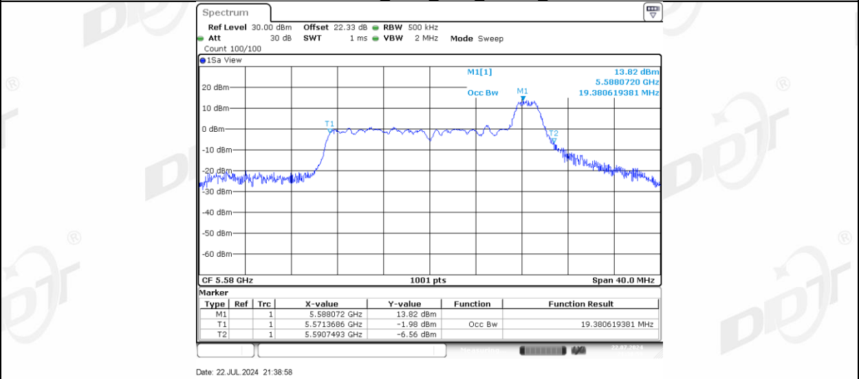
11AX20MIMO Ant-3 5580_52Tone_RU37
