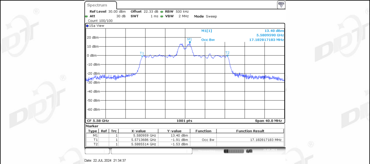
11AX20MIMO Ant-3 5580_26Tone_RU8
