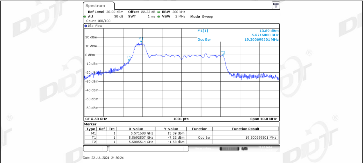
11AX20MIMO Ant-3 5580_26Tone_RU4
