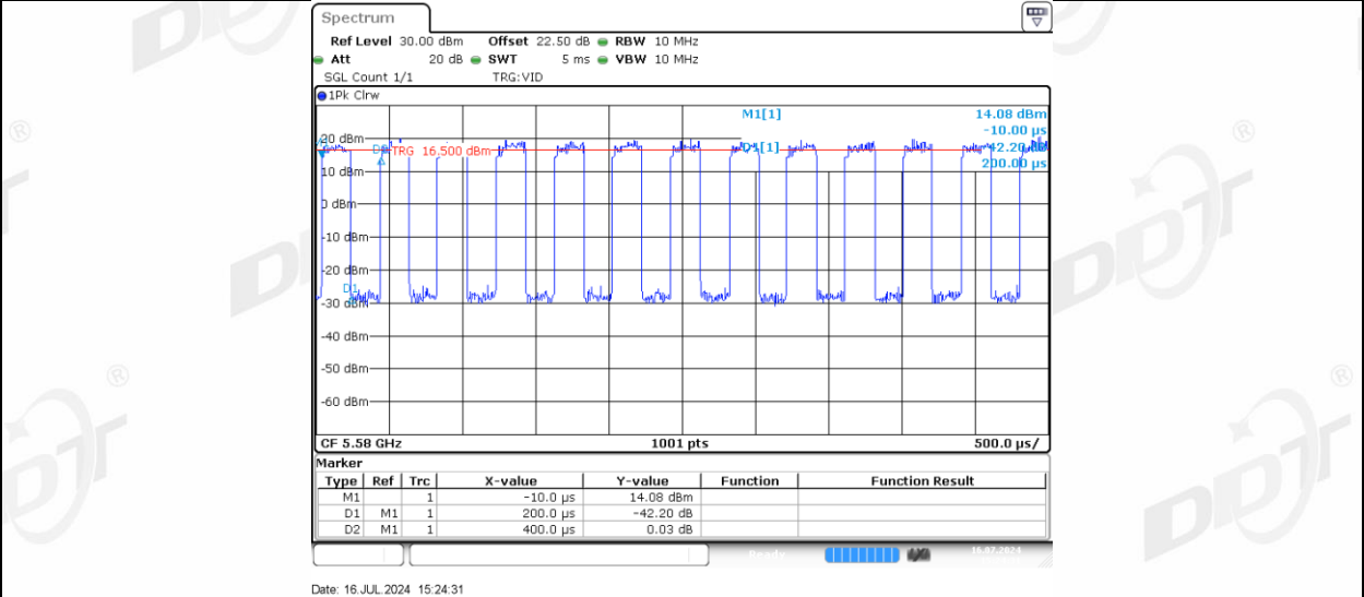
11AX20MIMO_Ant-3_5580
