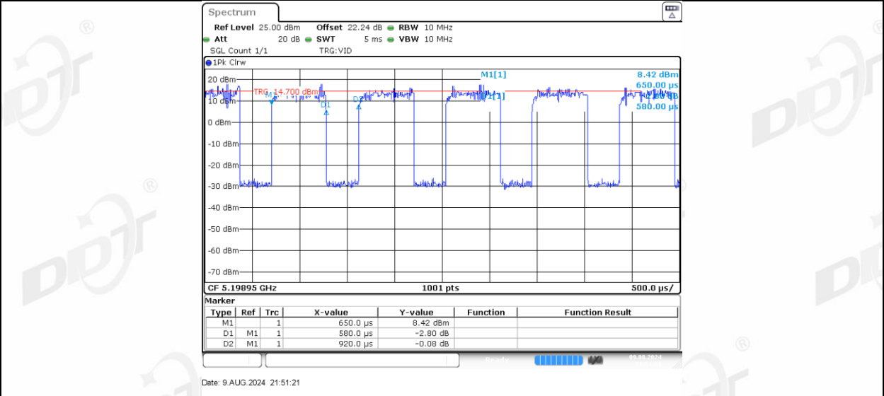
11AX20MIMO_Ant-3_5200_26Tone_RU8
