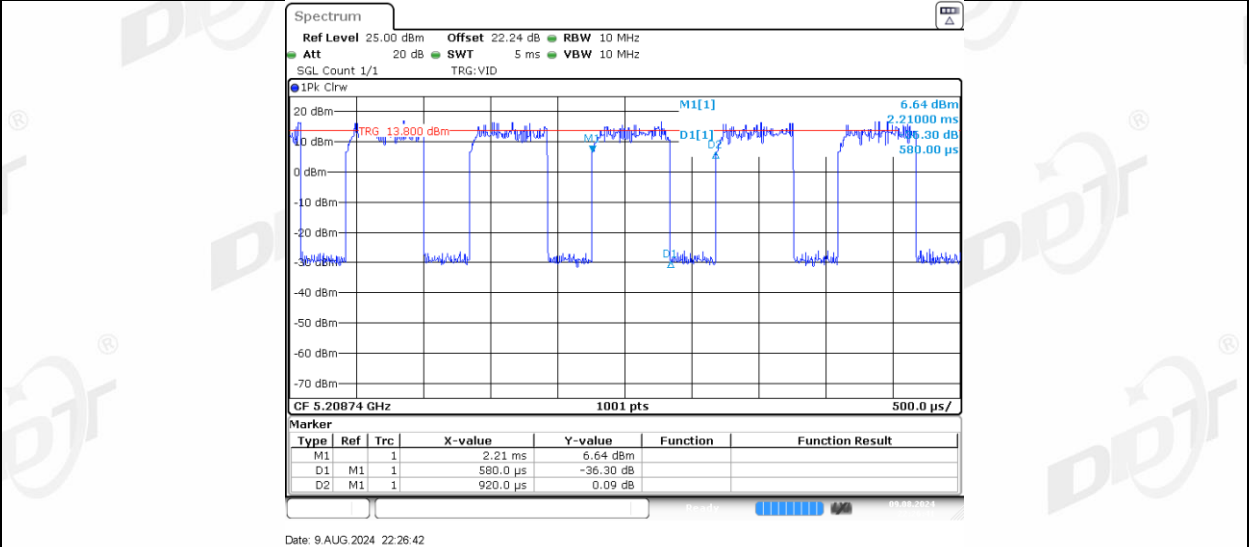
11AX20MIMO_Ant-3_5200_52Tone_RU37
