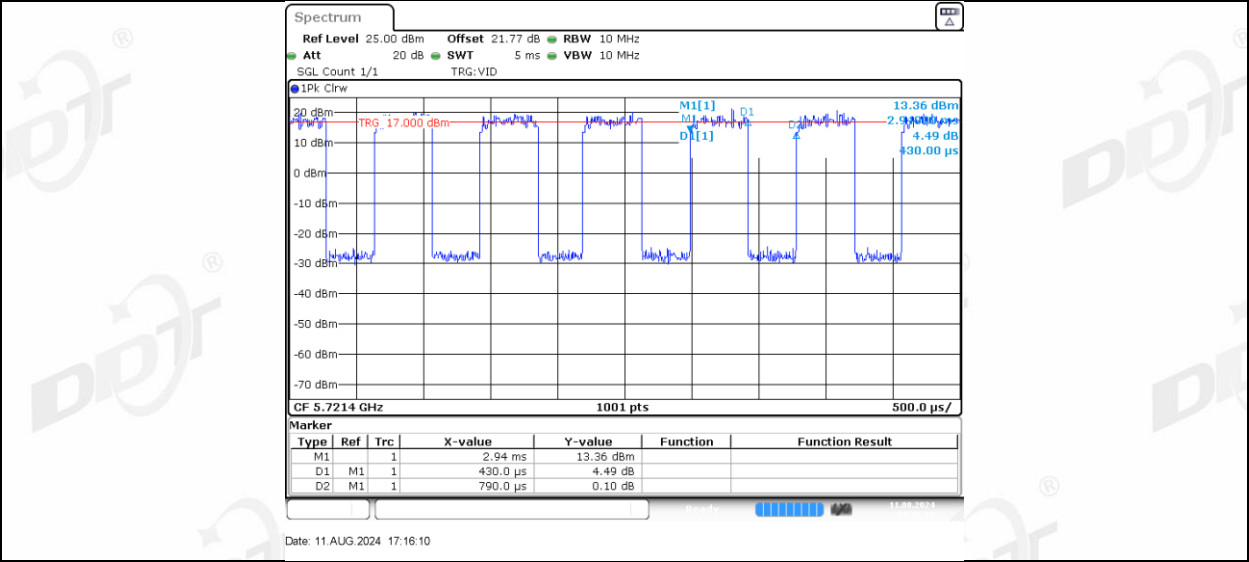
11AX20MIMO Ant-3 5720 26Tone RU0
