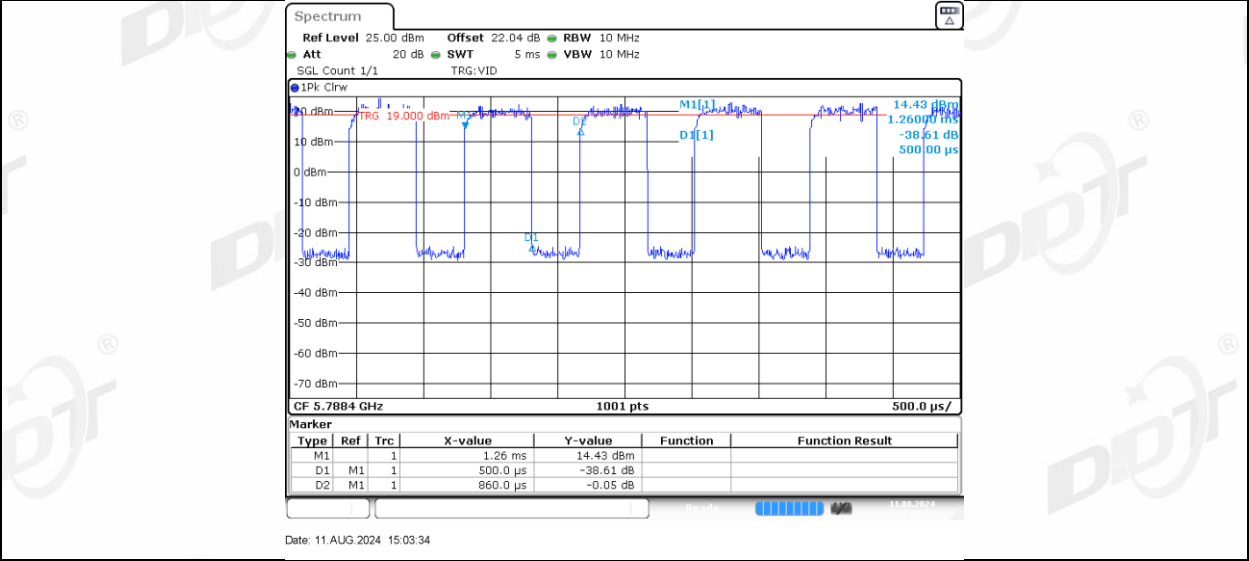
11AX20MIMO_Ant-3_5785_52Tone_RU40
