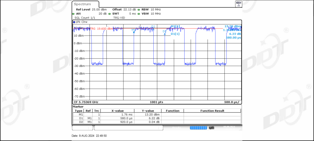
11AX20MIMO Ant-3 5745 52Tone RU37
