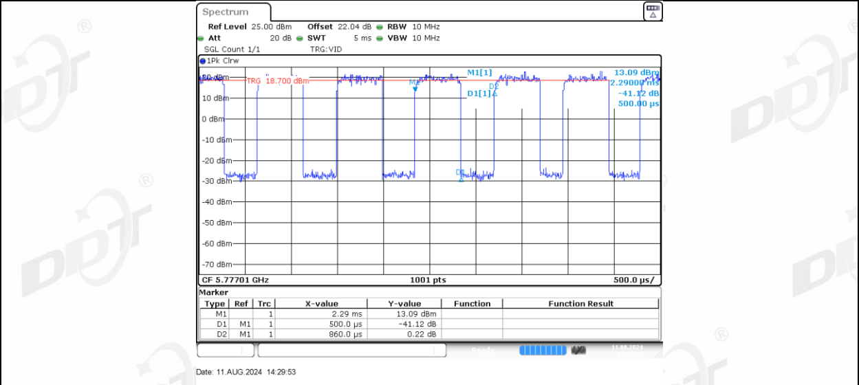
11AX20MIMO_Ant-3_5785_52Tone_RU39
