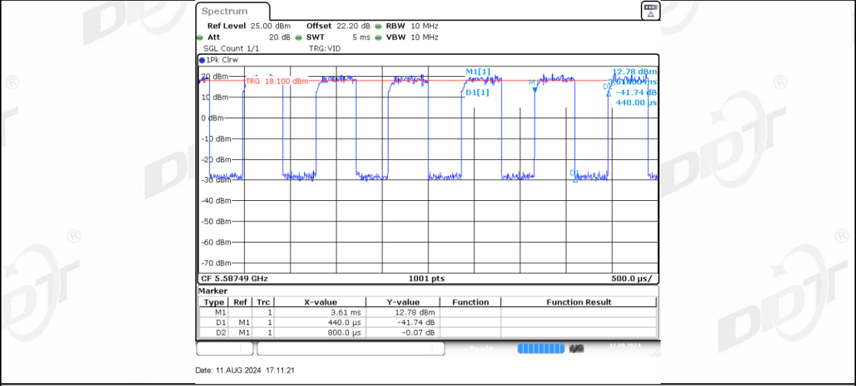
11AX20MIMO_Ant-3_5580_26Tone_RU0
