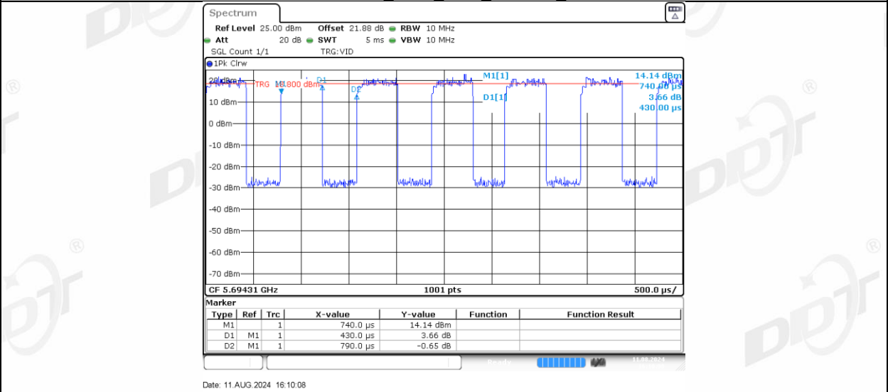
11AX20MIMO_Ant-1_5700_106Tone_RU54
