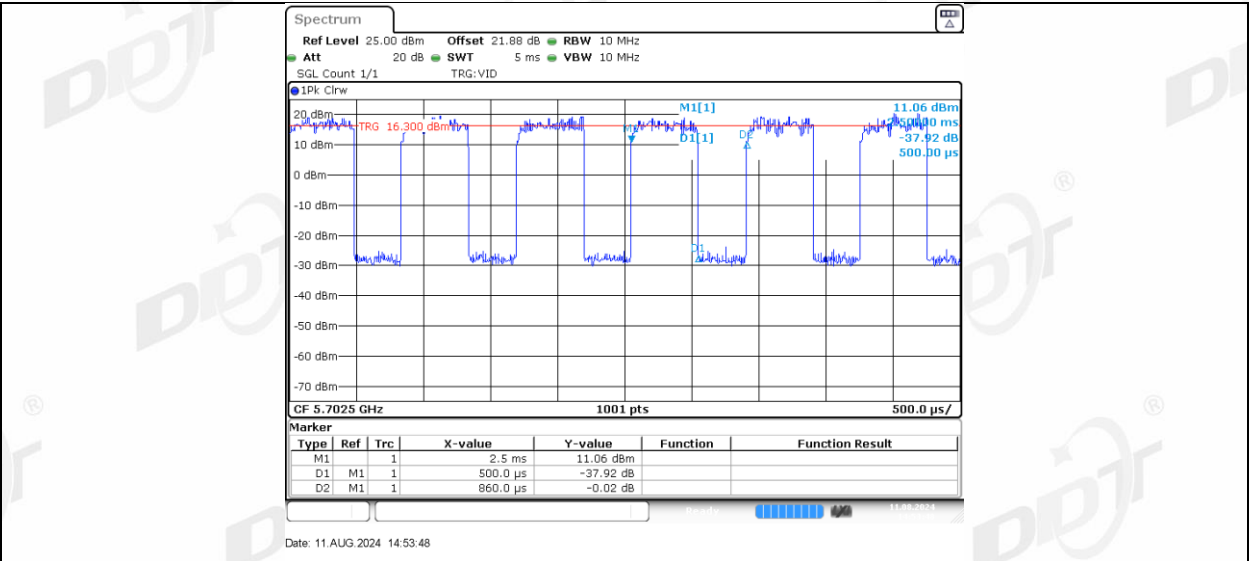
11AX20MIMO_Ant-1_5700_52Tone_RU40
