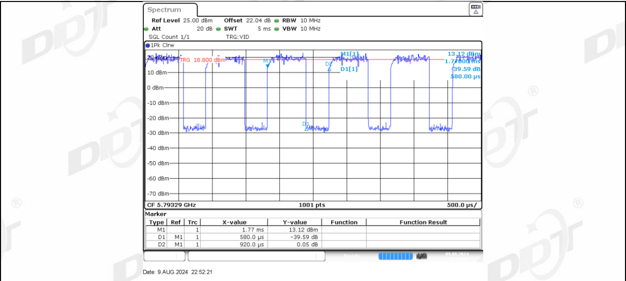
11AX20MIMO_Ant-3_5785_52Tone_RU37
