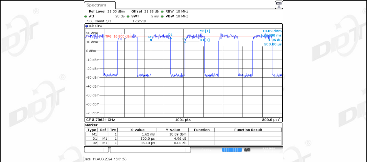
11AX20MIMO_Ant-1_5700_106Tone_RU53
