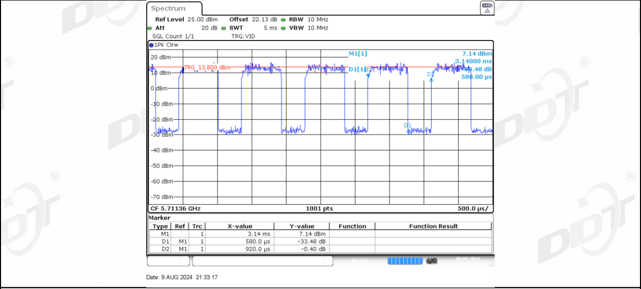
11AX20MIMO Ant-3 5720 26Tone RU4
