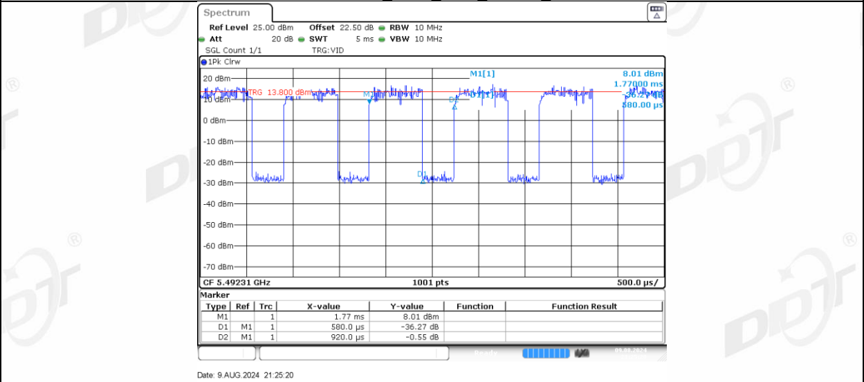
11AX20MIMO Ant-3_5500_26Tone_RU4
