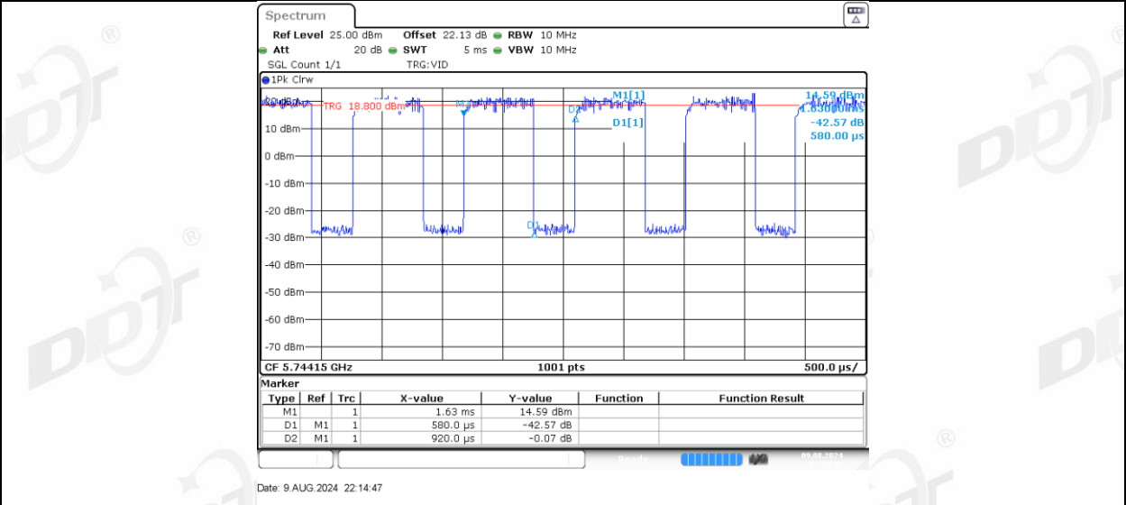
11AX20MIMO Ant-3 5745 26Tone RU8
