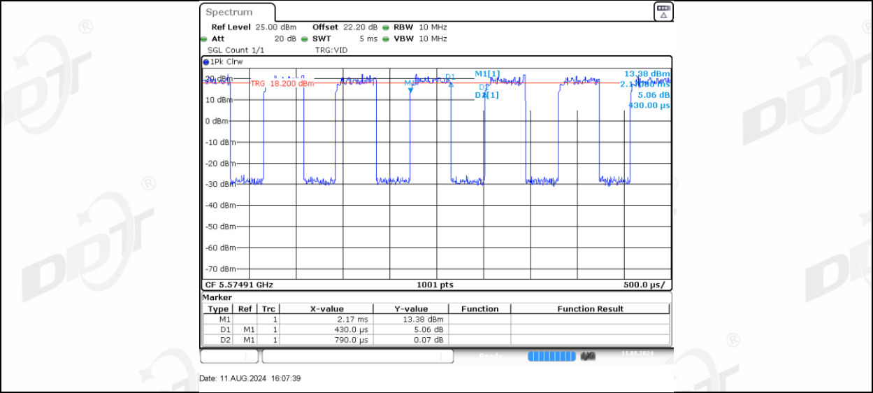
11AX20MIMO_Ant-1_5580_106Tone_RU54
