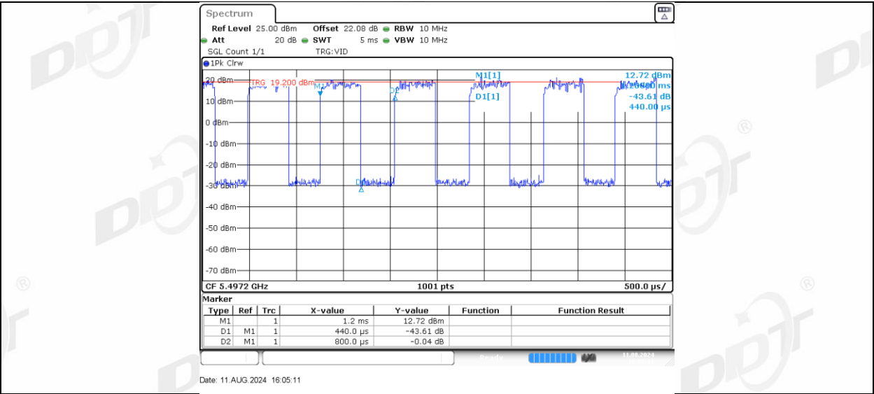
11AX20MIMO Ant-1_5500_106Tone_RU54
