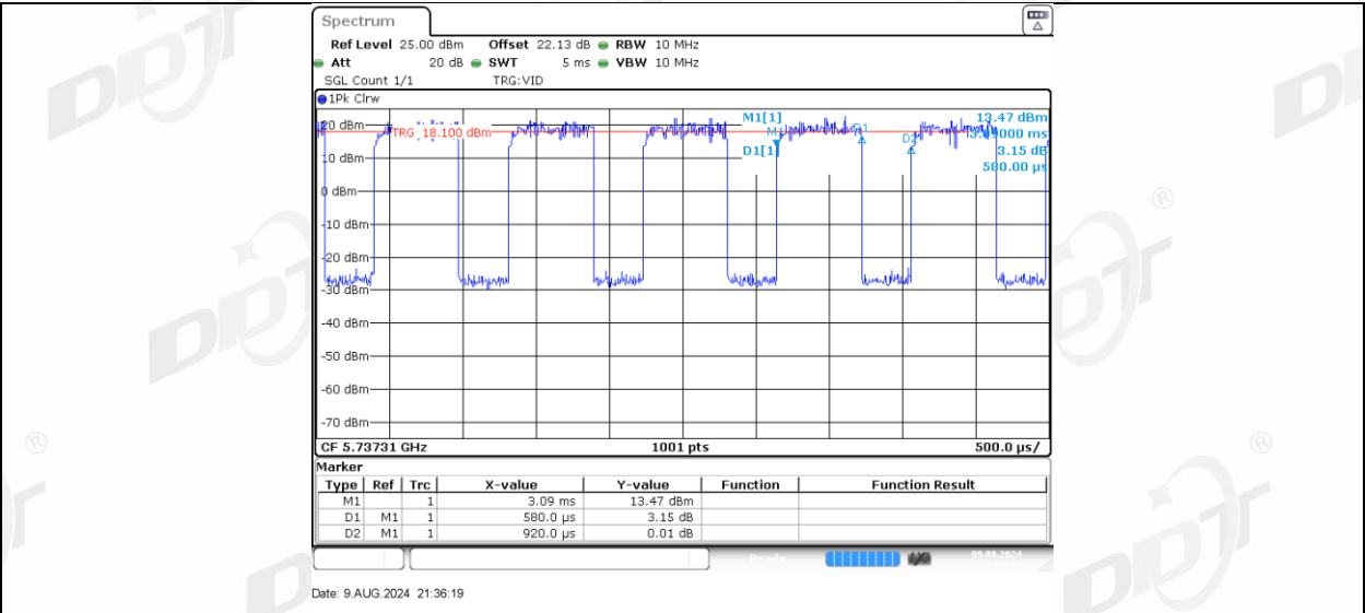
11AX20MIMO Ant-3 5745 26Tone RU4
