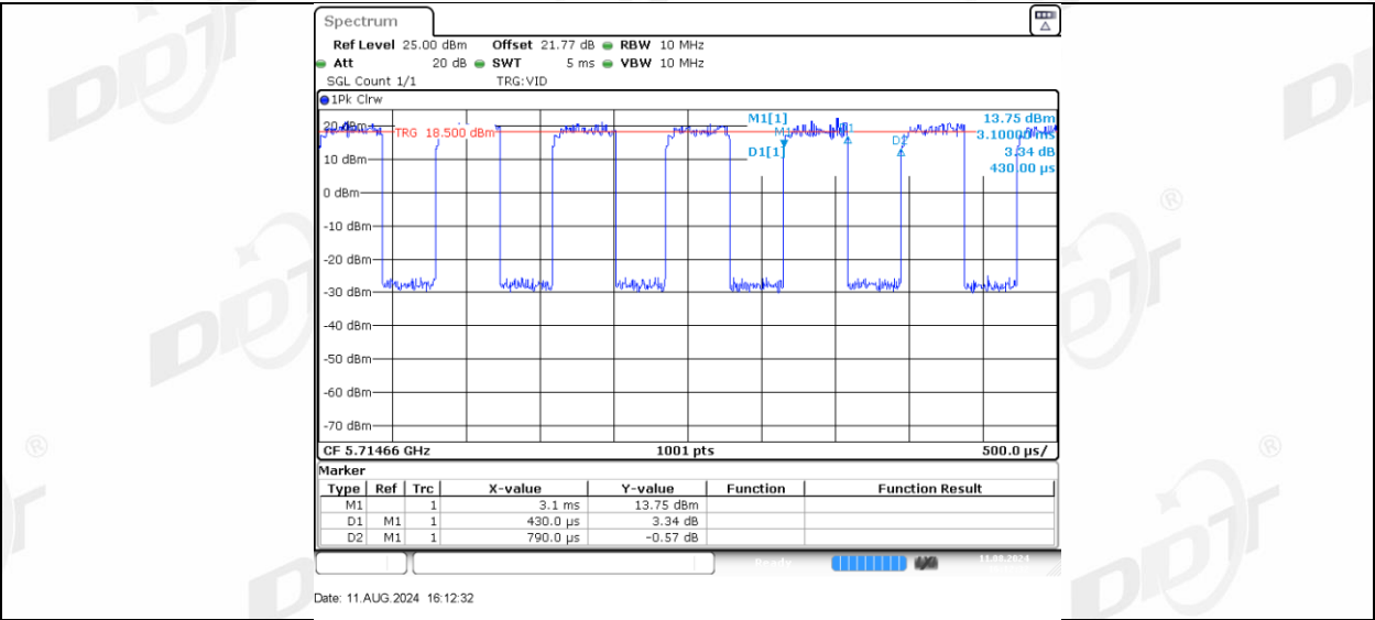
11AX20MIMO Ant-1 5720 106Tone RU54
