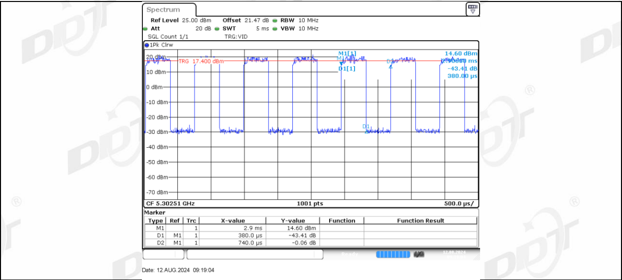
11AX40MIMO_Ant-1_5310_242Tone_RU62
