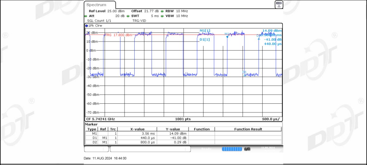
11AX40MIMO_Ant-1_5755_106Tone_RU56
