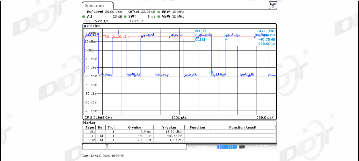
11AX40MIMO_Ant-3_5510_106Tone_RU53
