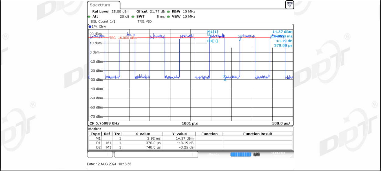
11AX40MIMO_Ant-3_5755_106Tone_RU53
