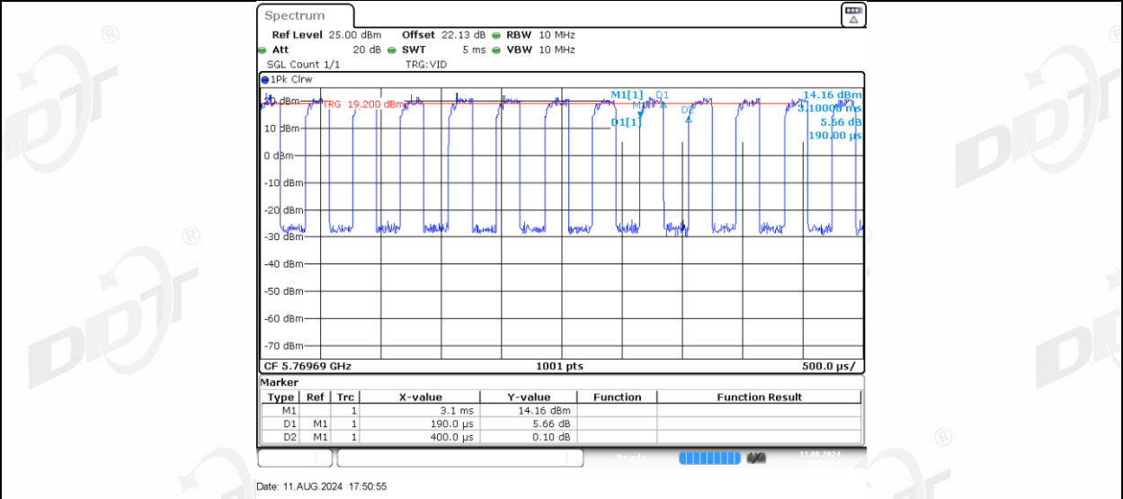
11AX40MIMO_Ant-3_5755_242Tone_RU61
