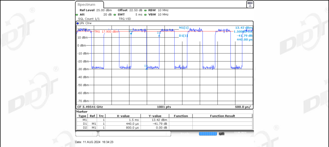
11AX40MIMO_Ant-3_5510_106Tone_RU56
