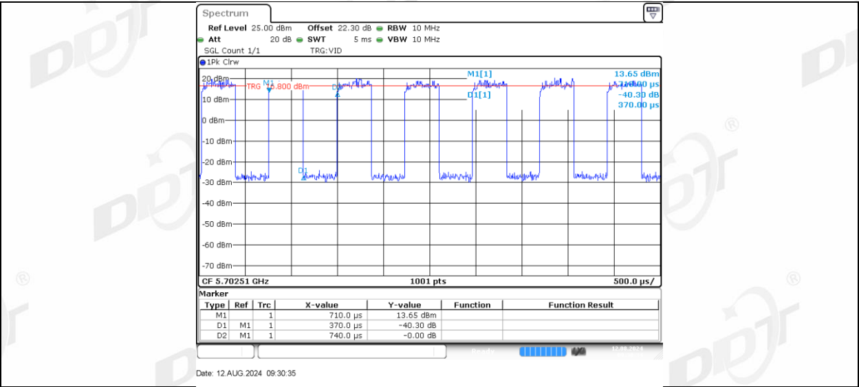
11AX40MIMO_Ant-3_5710_242Tone_RU62
