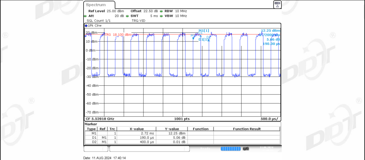
11AX40MIMO_Ant-3_5510_242Tone_RU61
