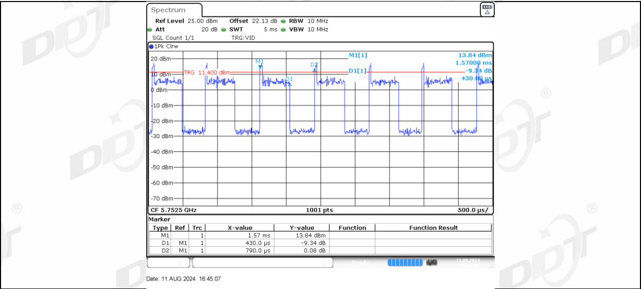
11AX40MIMO_Ant-3_5755_106Tone_RU56
