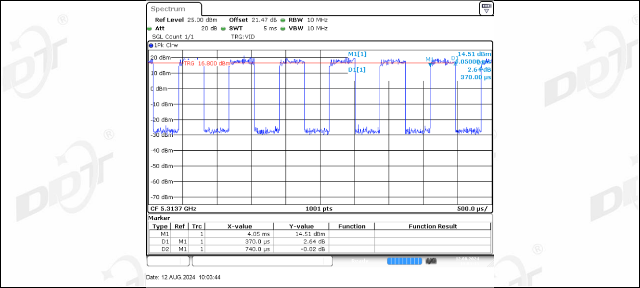
11AX40MIMO_Ant-3_5310_106Tone_RU53
