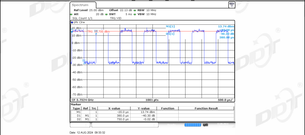
11AX40MIMO_Ant-3_5755_242Tone_RU62
