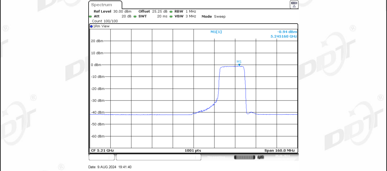
11AX80MIMO_Ant-3_5210_484Tone_RU65
