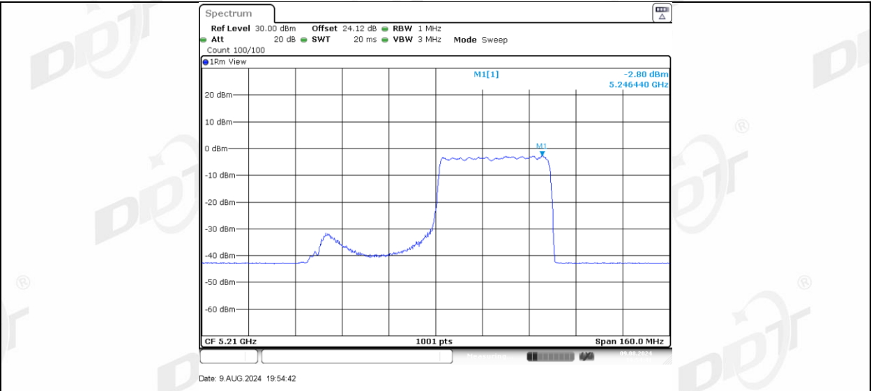
11AX80MIMO_Ant-3_ 242Tone_RU61
