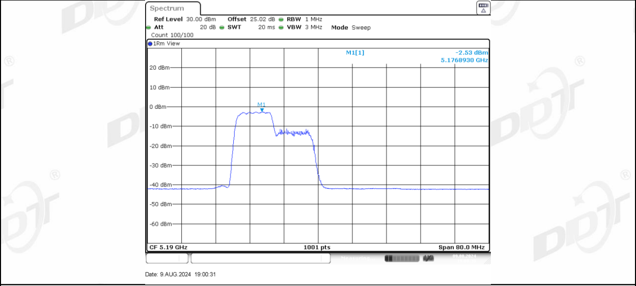
11AX40MIMO_Ant-1_5190_106Tone_RU56
