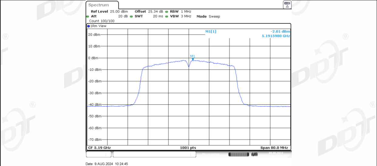
11AC40MIMO_Ant-3_5190
