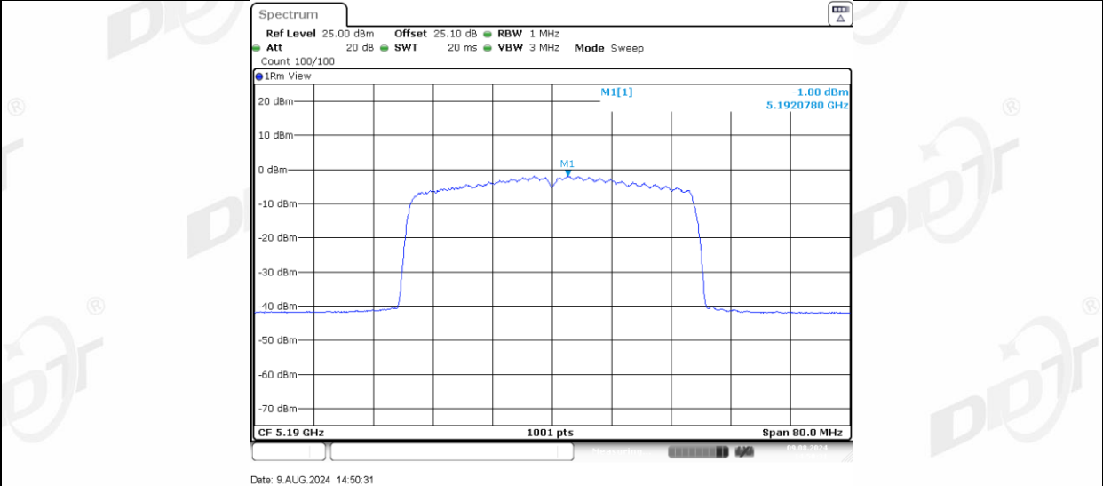
11AX40MIMO_Ant-3_5190
