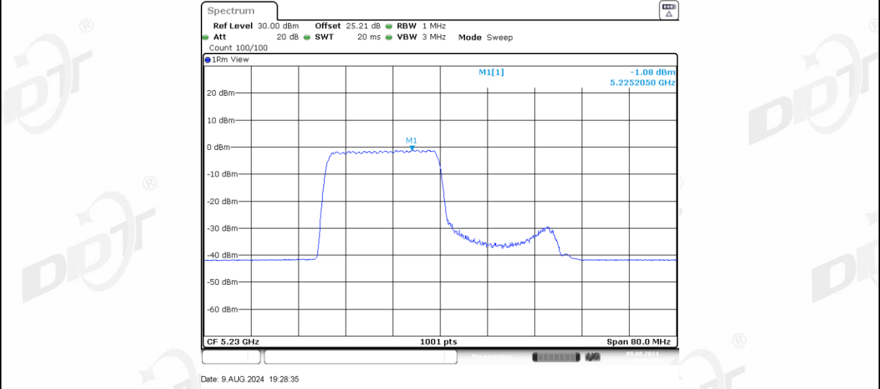
11AX40MIMO_Ant-3_5230_242Tone_RU62
