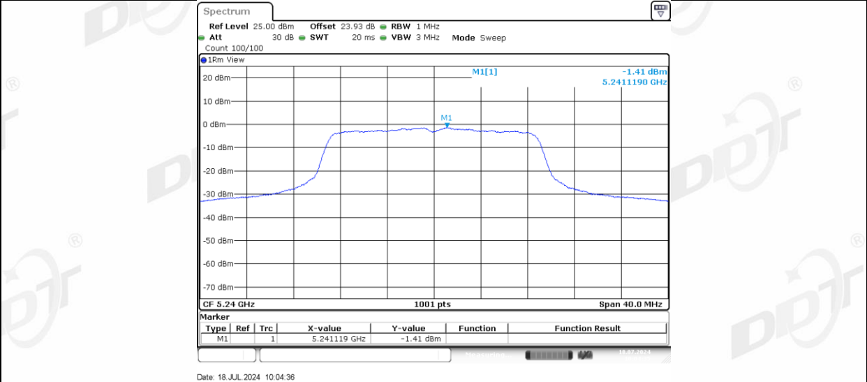
11N20MIMO_Ant-3_5240
