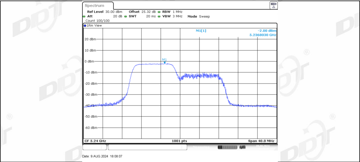
11AX20MIMO_Ant-3_5240_106Tone_RU54
