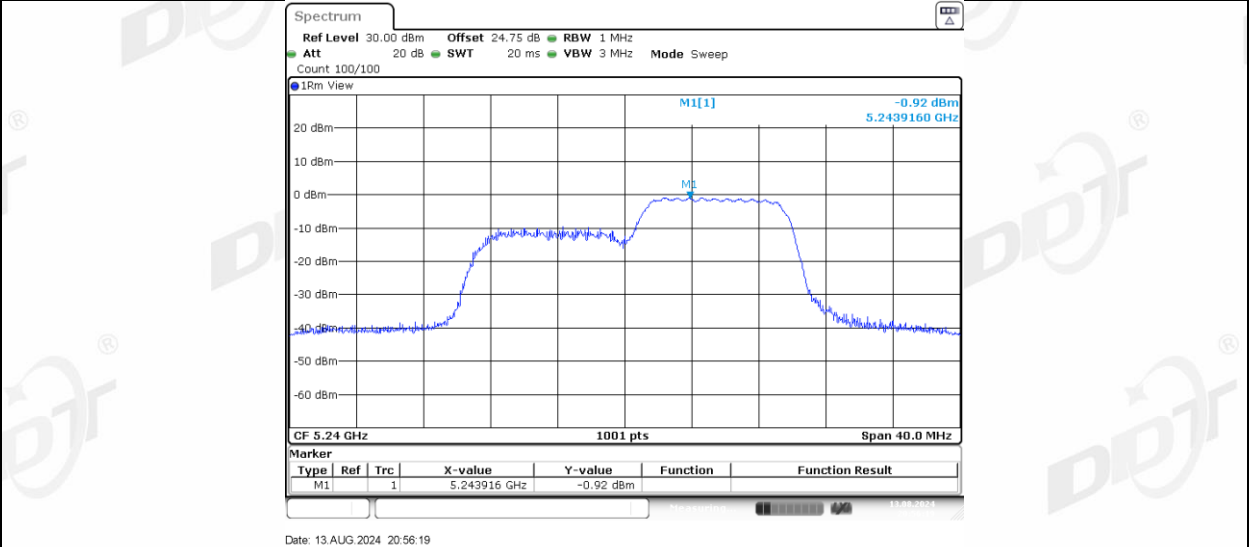
11AX20MIMO_Ant-3_5240_26Tone_RU0
