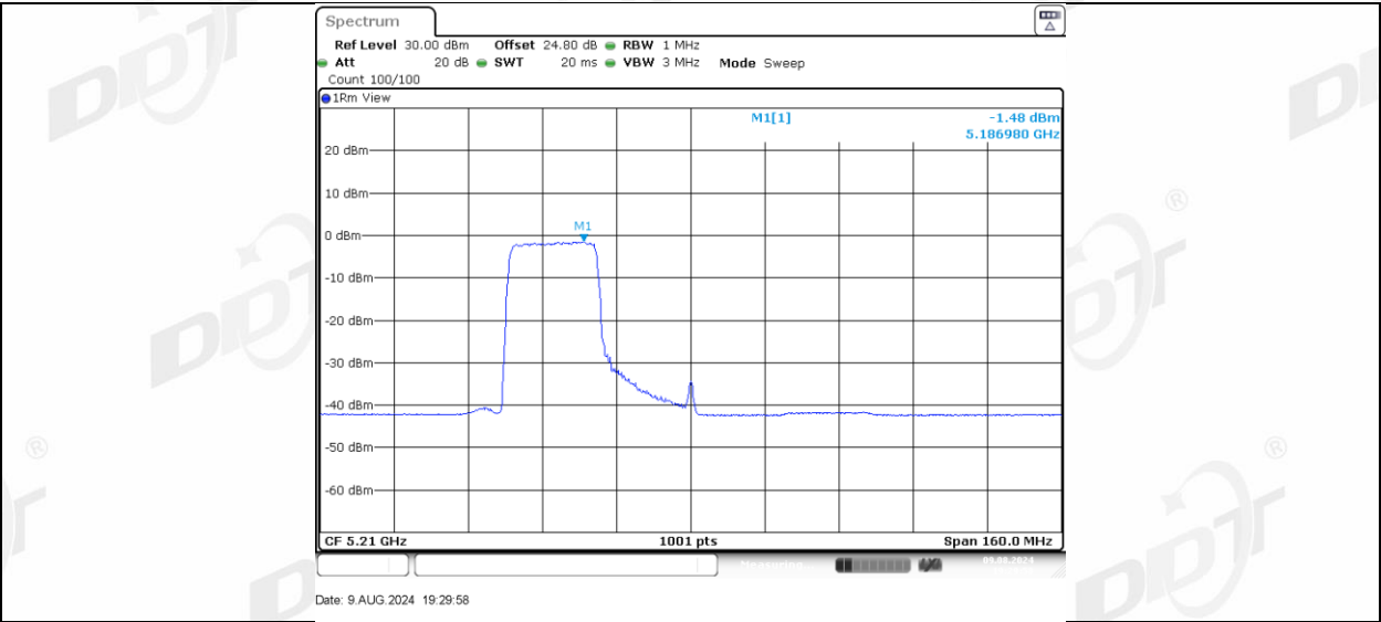
11AX80MIMO_Ant-1_5210_242Tone_RU64
