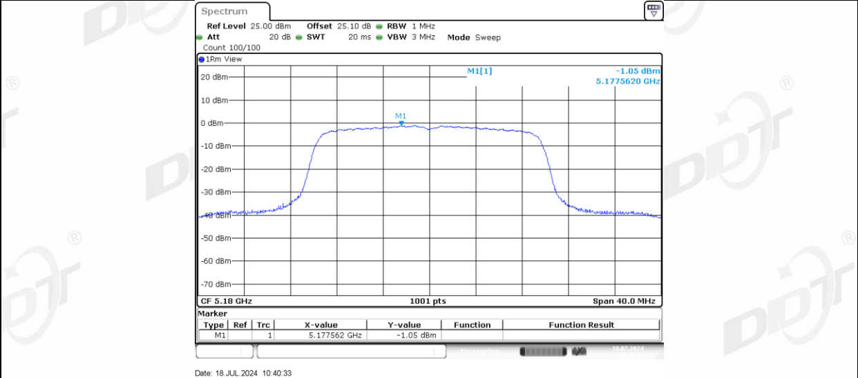
11AX20MIMO_Ant-3_5180
