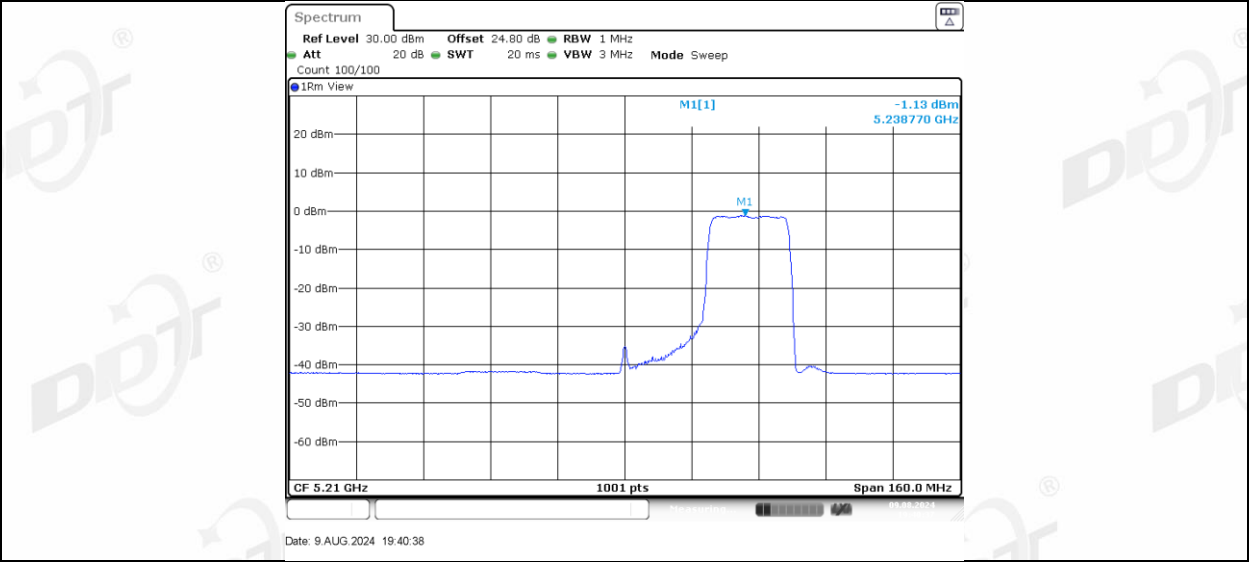
11AX80MIMO_Ant-1_5210_484Tone_RU65
