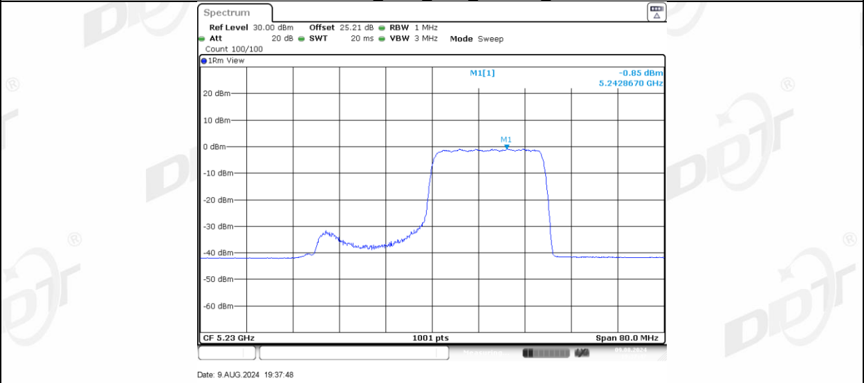
11AX80MIMO_Ant-1_5210_242Tone_RU61
