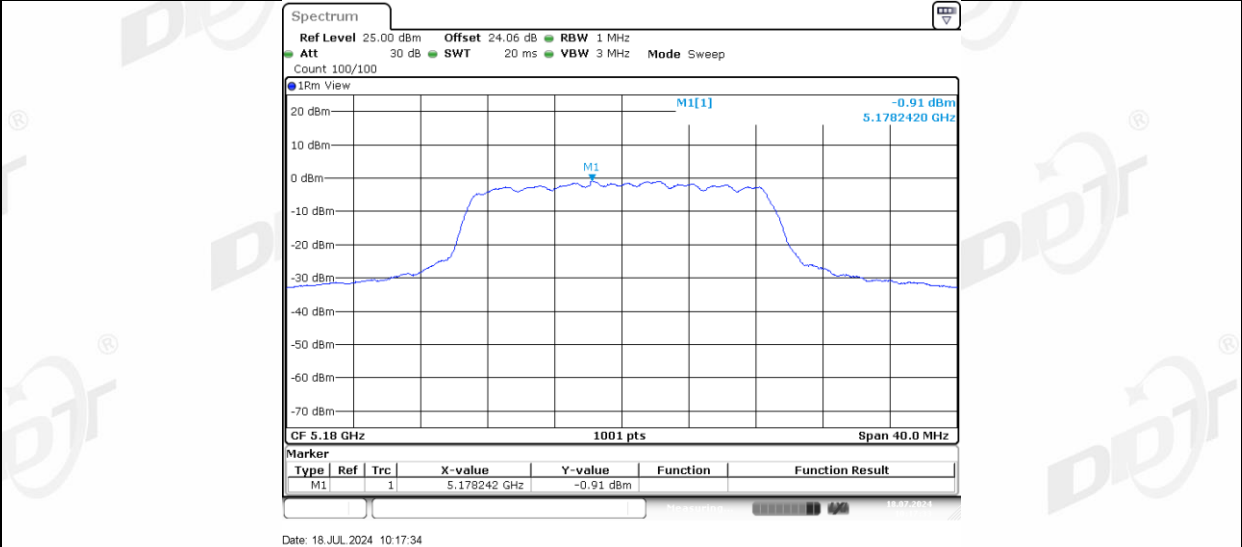
11AC20MIMO_Ant-3_5180
