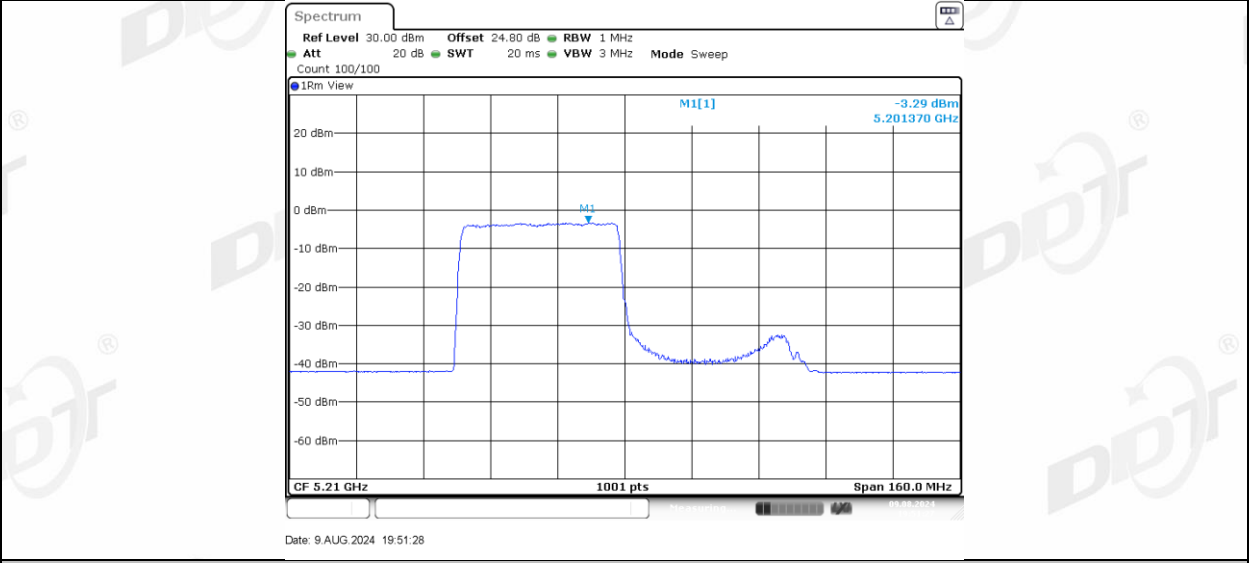
11AX80MIMO_Ant-1_5210_484Tone_RU66
