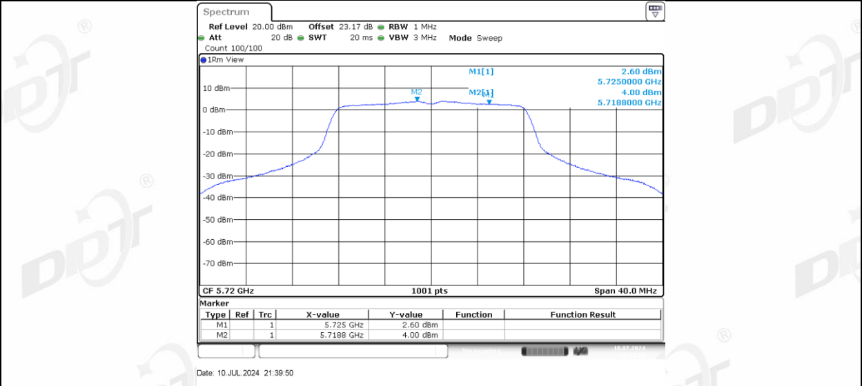
11A-CDD_Ant-1_5720_UNII-3
