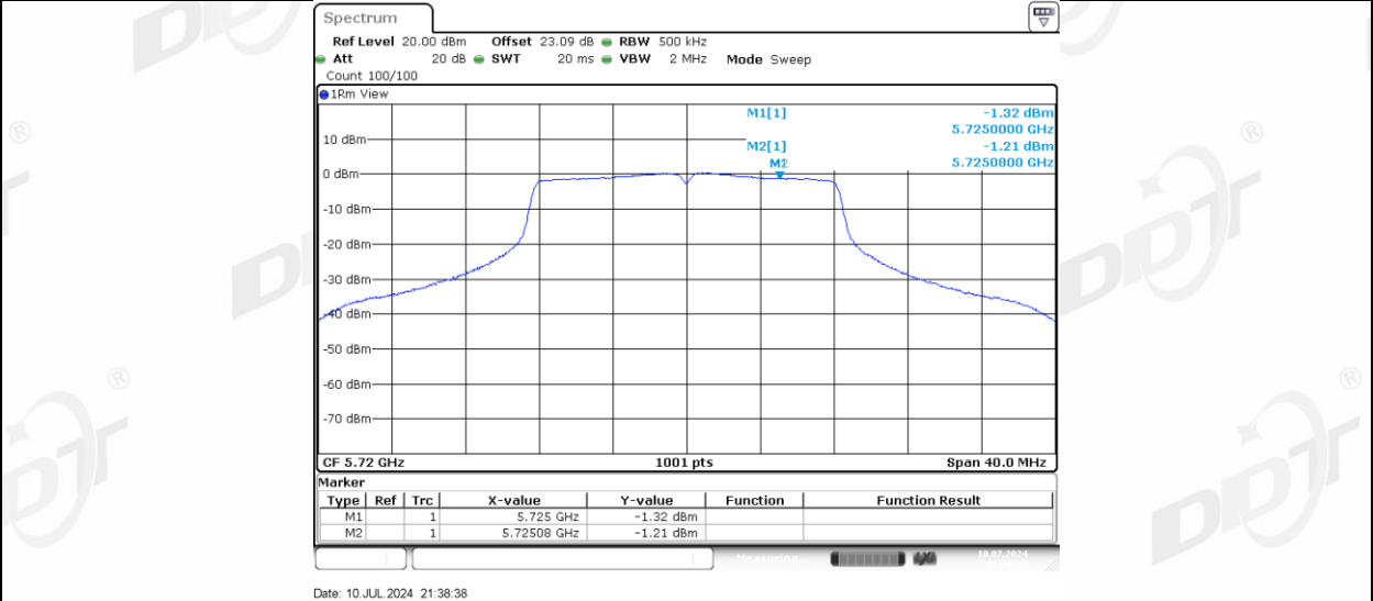
11A-CDD_Ant-3_5720_UNII-3
