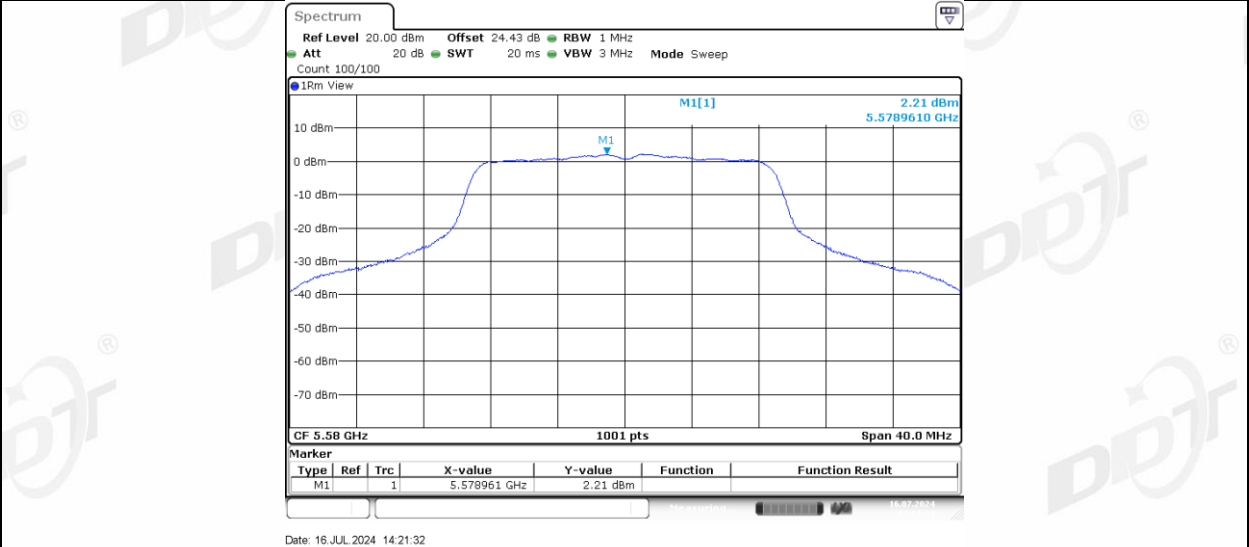
11AC20MIMO_Ant-3_5580
