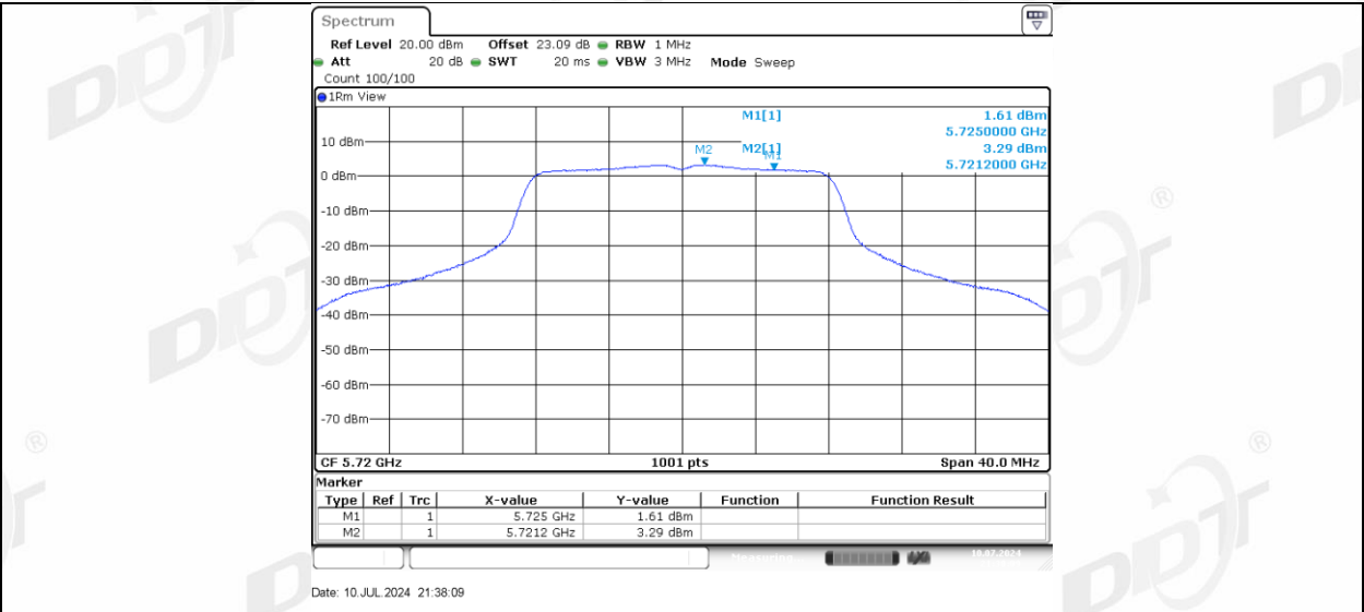
11A-CDD_Ant-3_5720_UNII-2C
