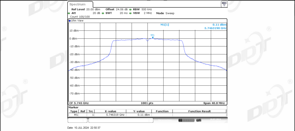
11N20MIMO_Ant-3_5745
