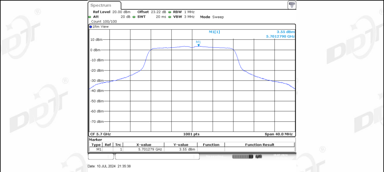
11A-CDD_Ant-3_5700
