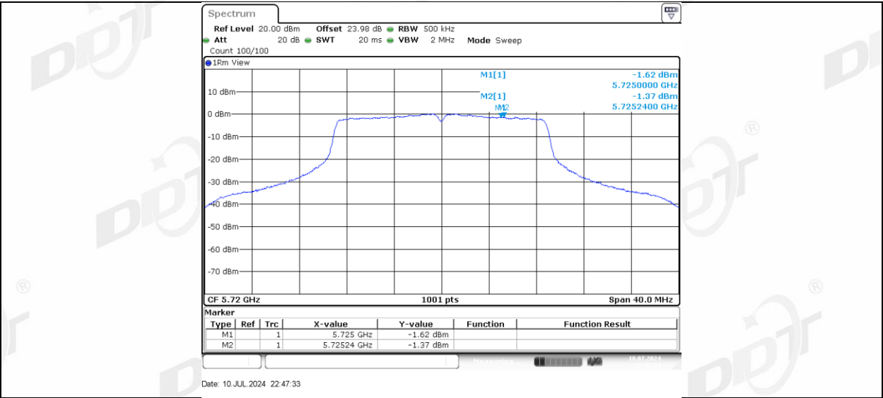
11N20MIMO_Ant-3_5720_UNII-3
