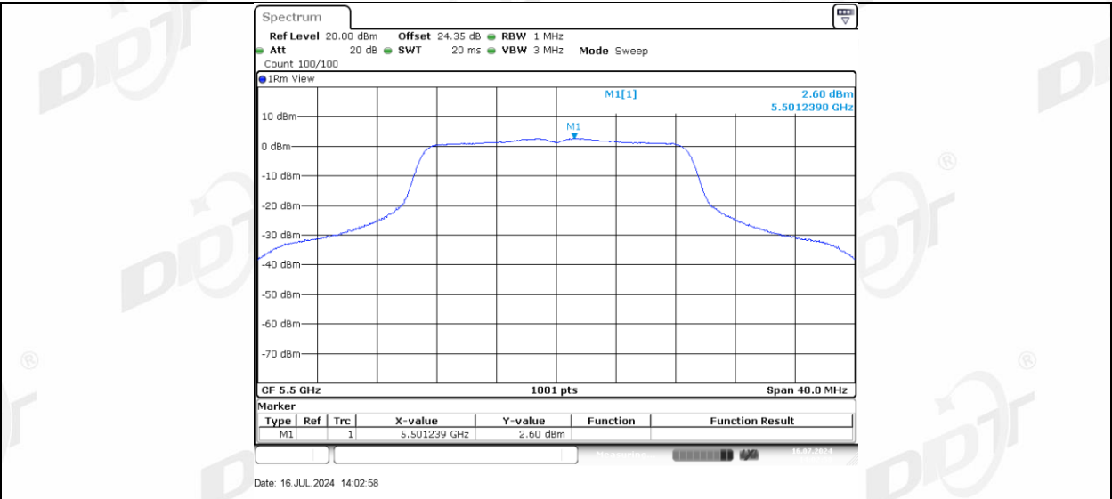
11AC20MIMO_Ant-3_5500
