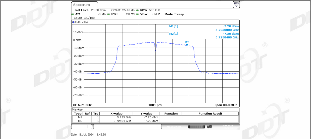
11N40MIMO_Ant-3_5710_UNII-3
