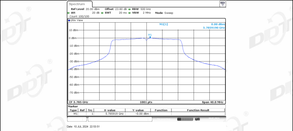
11N20MIMO_Ant-3_5785
