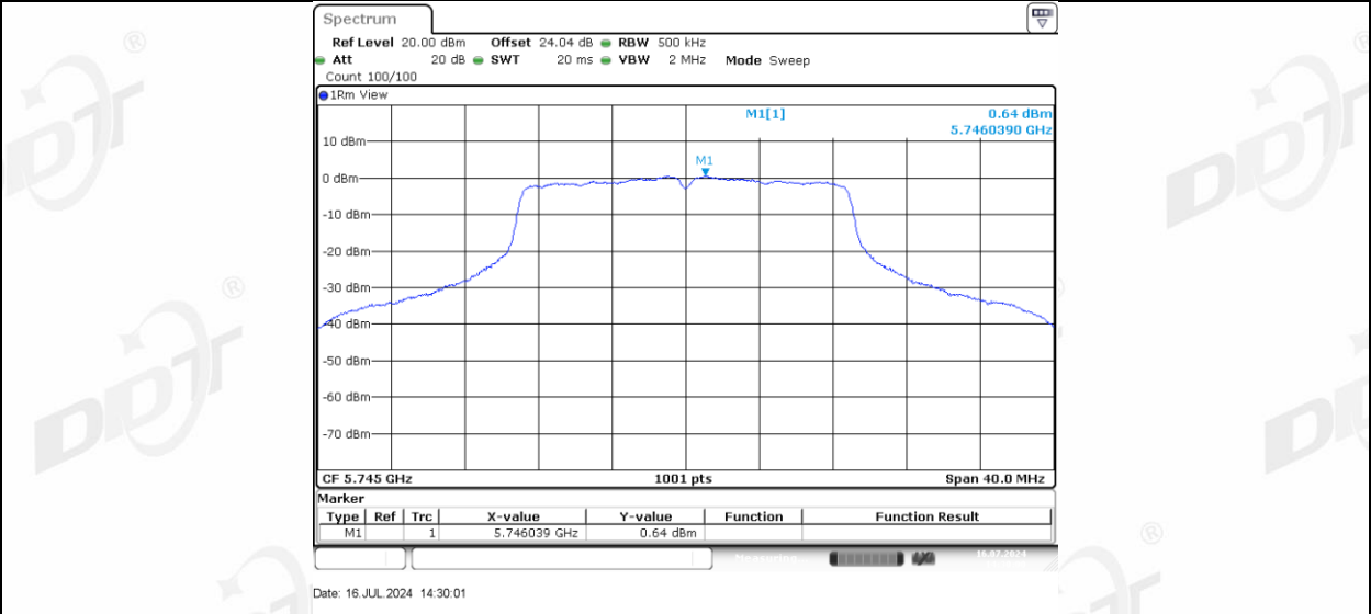
11AC20MIMO_Ant-3_5745
