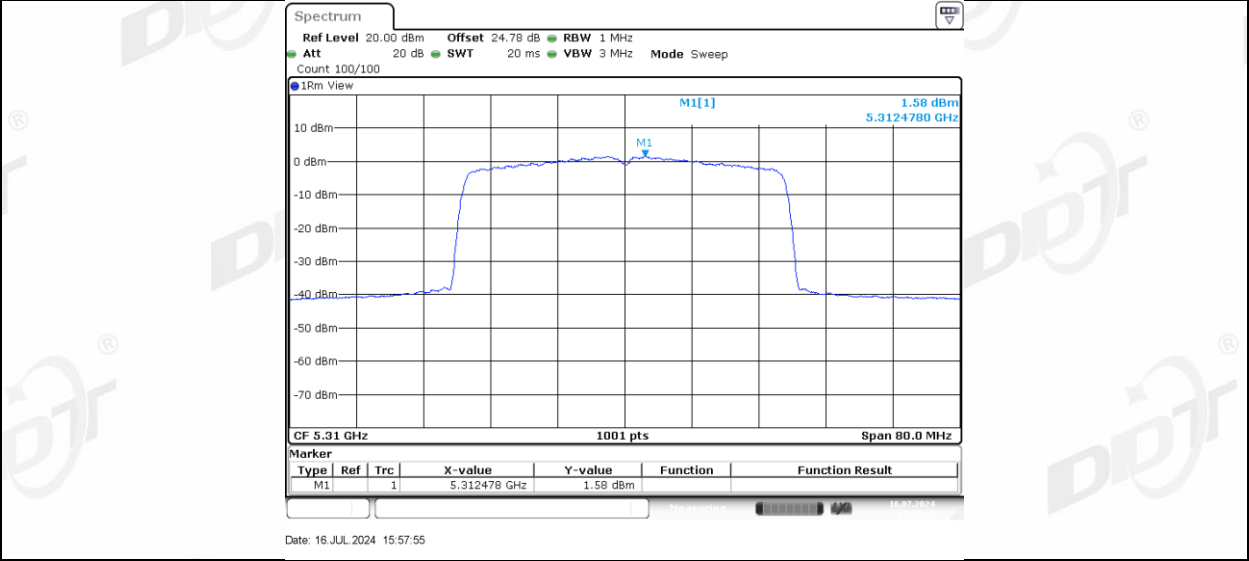
11AX40MIMO Ant-3_5310
