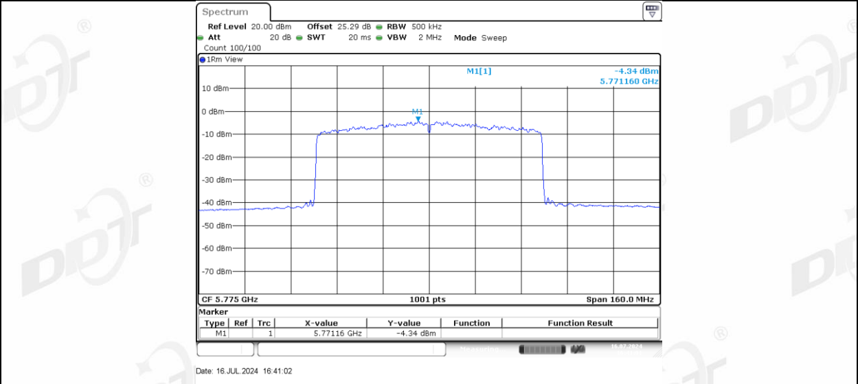
11AX80MIMO_Ant-3_5775
