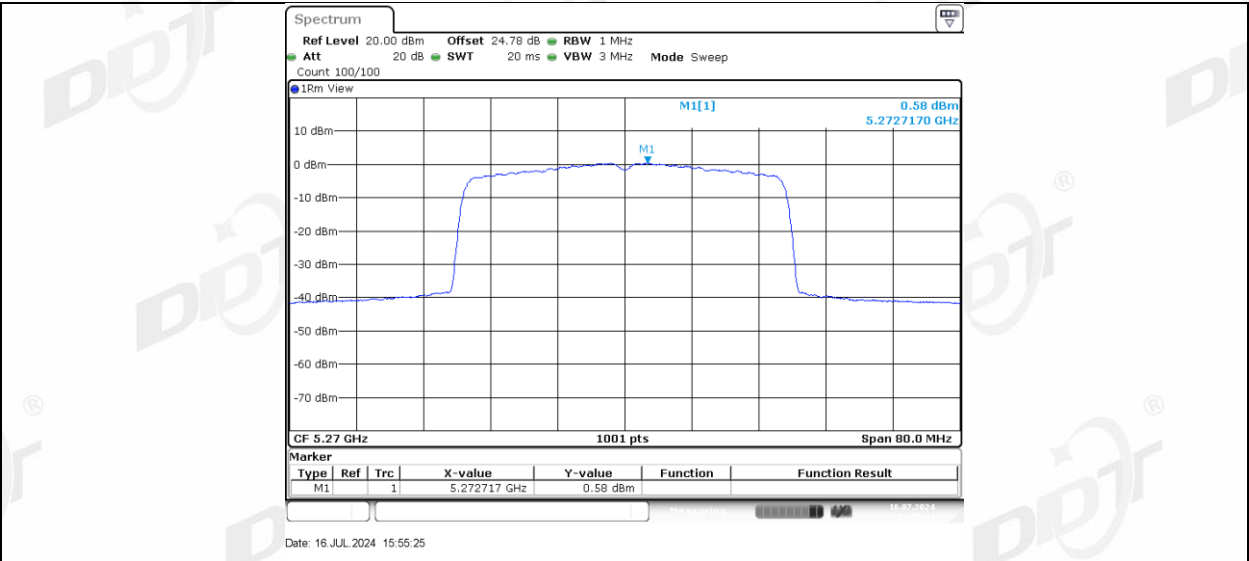
11AX40MIMO Ant-3_5270
