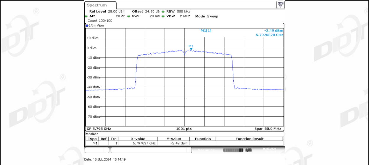
11AX40MIMO Ant-3_5795
