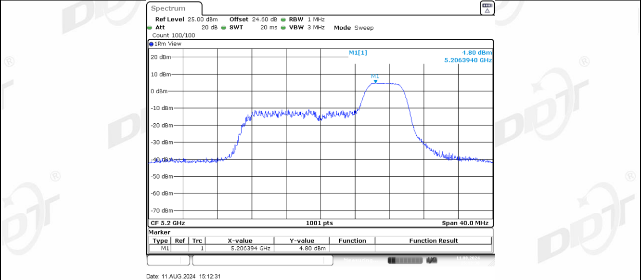
11AX20MIMO_Ant-3_5200_106Tone_RU53
