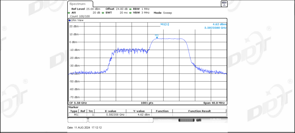
11AX20MIMO Ant-3 5580 26Tone RU0
