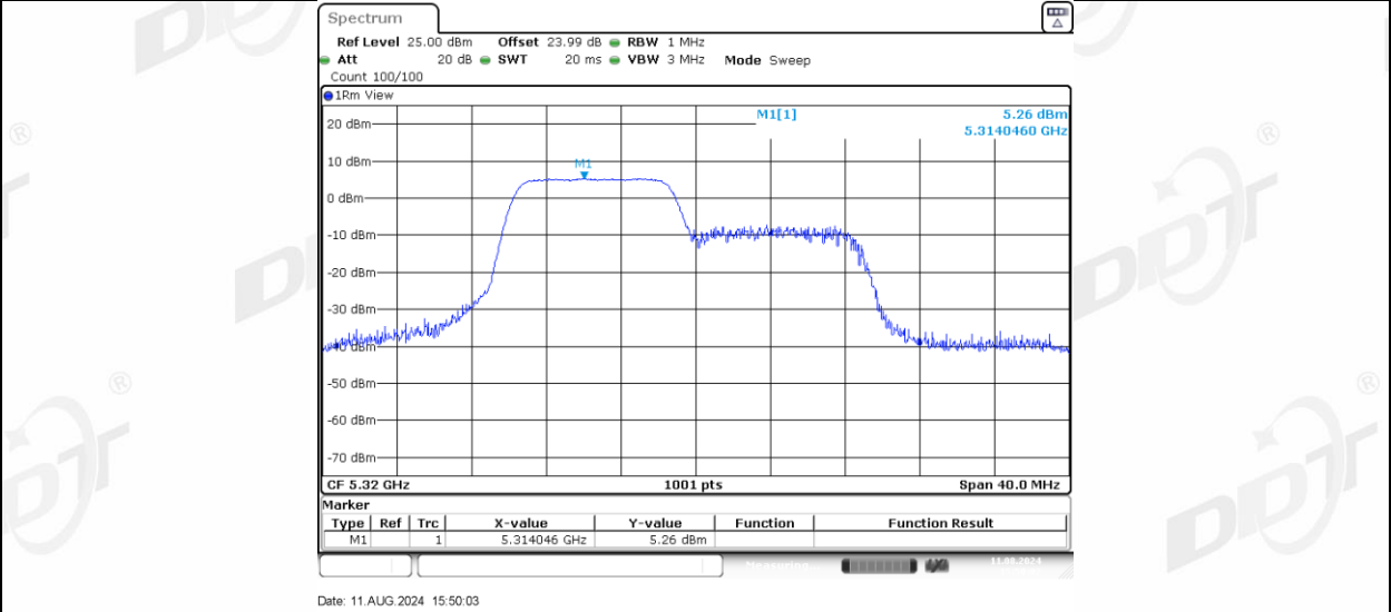
11AX20MIMO_Ant-1_5320_106Tone_RU54
