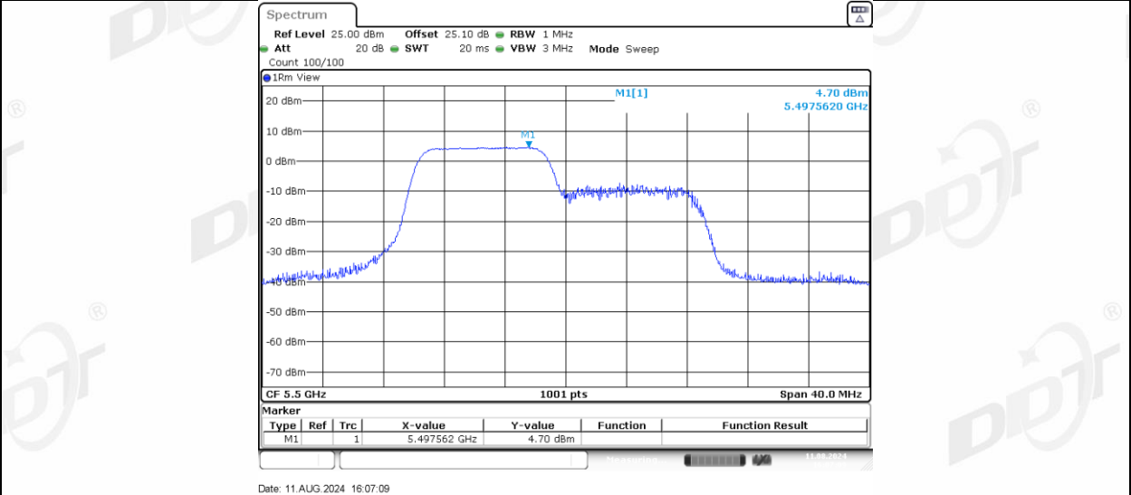
11AX20MIMO_Ant-3_5500_106Tone_RU54
