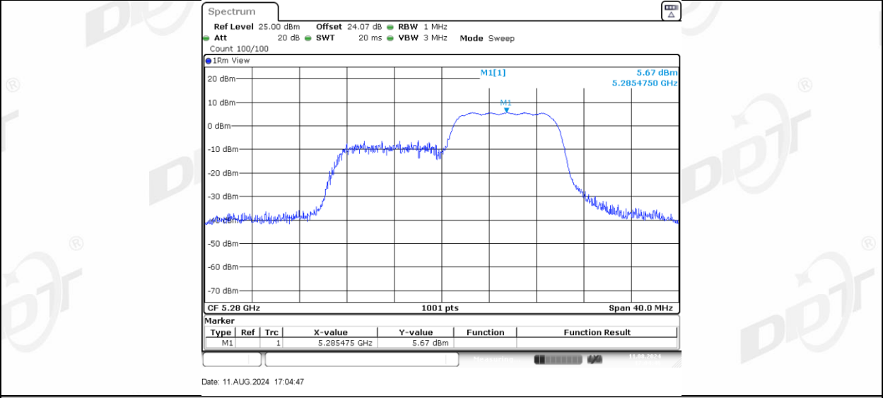
11AX20MIMO Ant-3 5280 26Tone RU0
