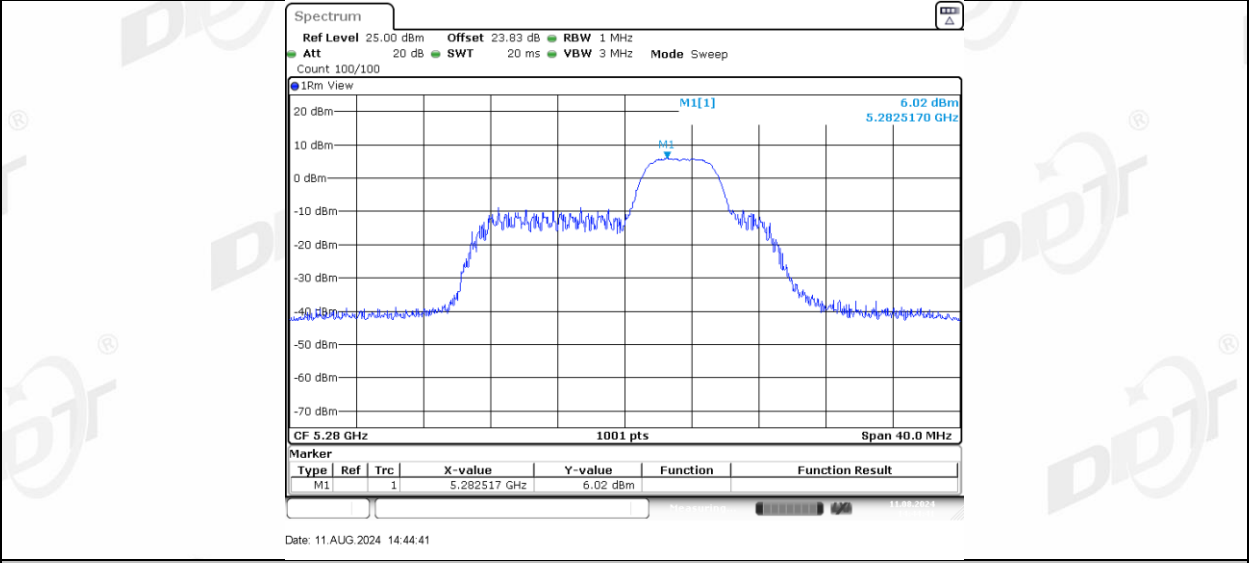
11AX20MIMO_Ant-1_5280_52Tone_RU40
