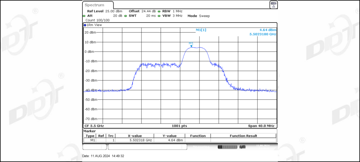
11AX20MIMO_Ant-1_5500_52Tone_RU40
