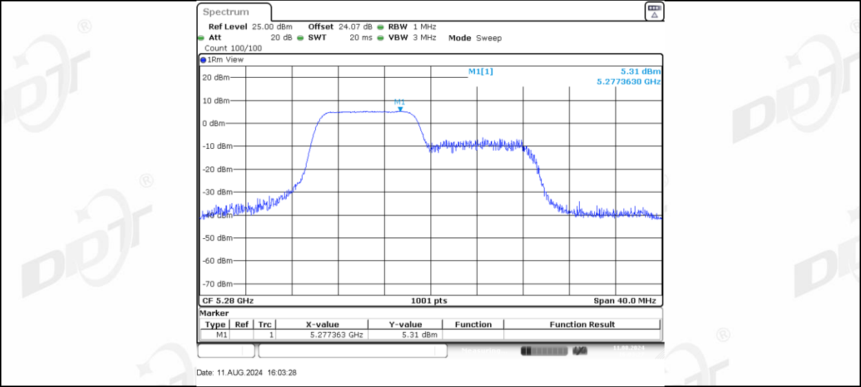
11AX20MIMO Ant-1 5280 106Tone RU54
