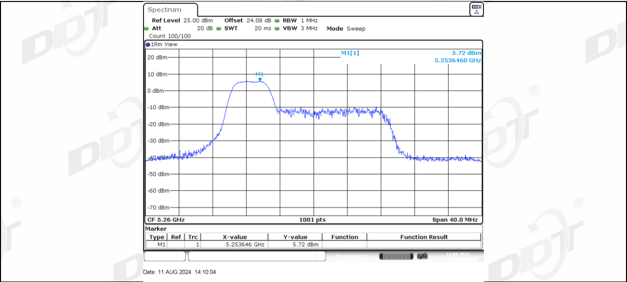
11AX20MIMO_Ant-1_5260_52Tone_RU39
