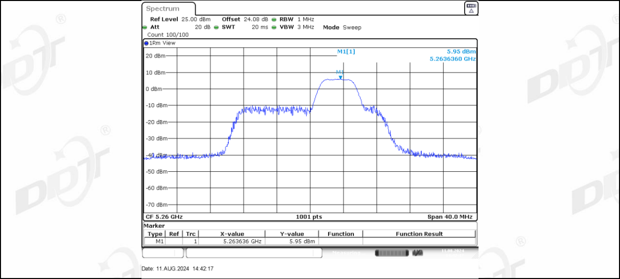
11AX20MIMO_Ant-1_5260_52Tone_RU40
