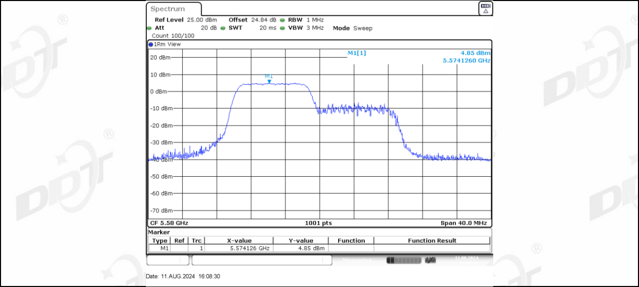
11AX20MIMO Ant-1 5580 106Tone RU54
