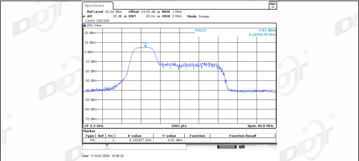
11AX20MIMO_Ant-3_5200_52Tone_RU39
