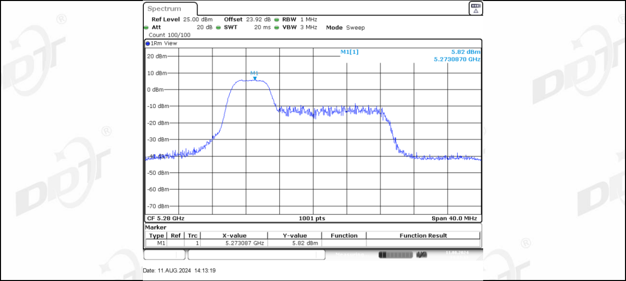
11AX20MIMO_Ant-1_5280_52Tone_RU39
