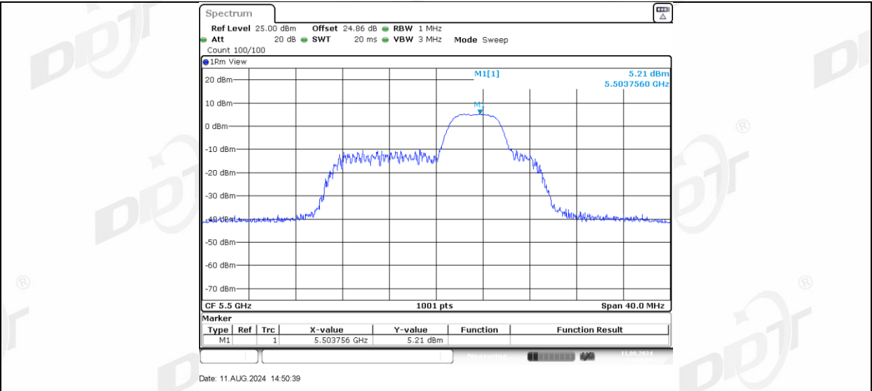
11AX20MIMO_Ant-3_5500_52Tone_RU40
