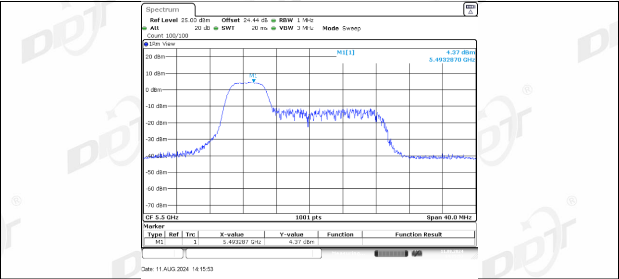
11AX20MIMO_Ant-1_5500_52Tone_RU39
