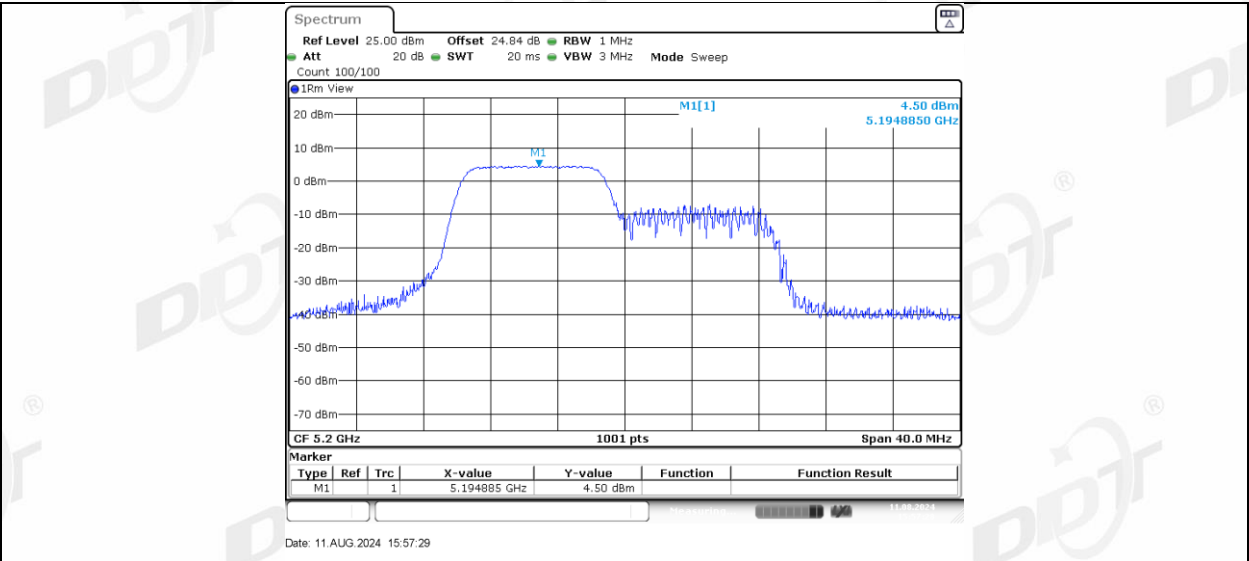
11AX20MIMO Ant-3 5200 106Tone RU54
