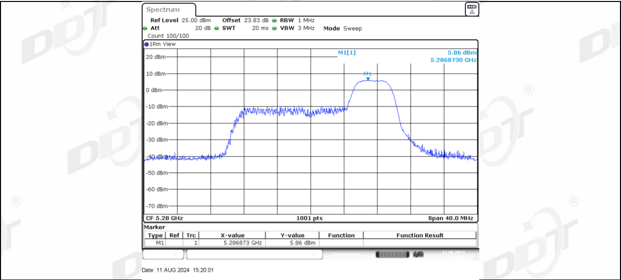
11AX20MIMO Ant-1 5280 106Tone RU53
