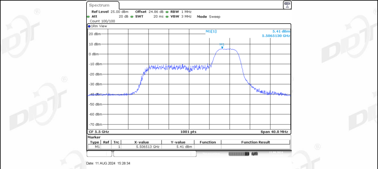
11AX20MIMO_Ant-3_5500_106Tone_RU53
