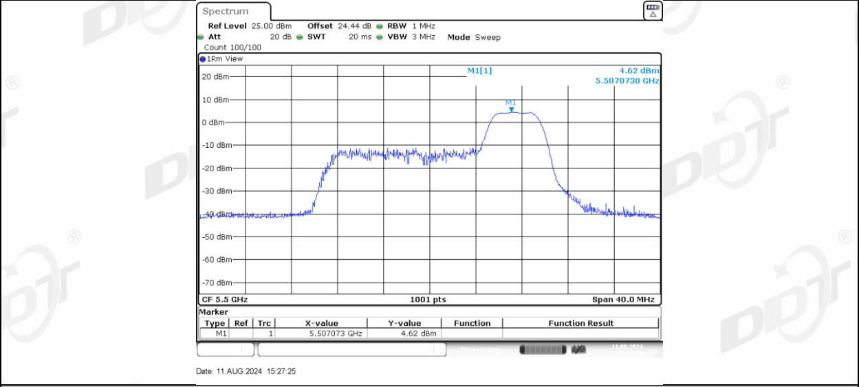
11AX20MIMO_Ant-1_5500_106Tone_RU53
