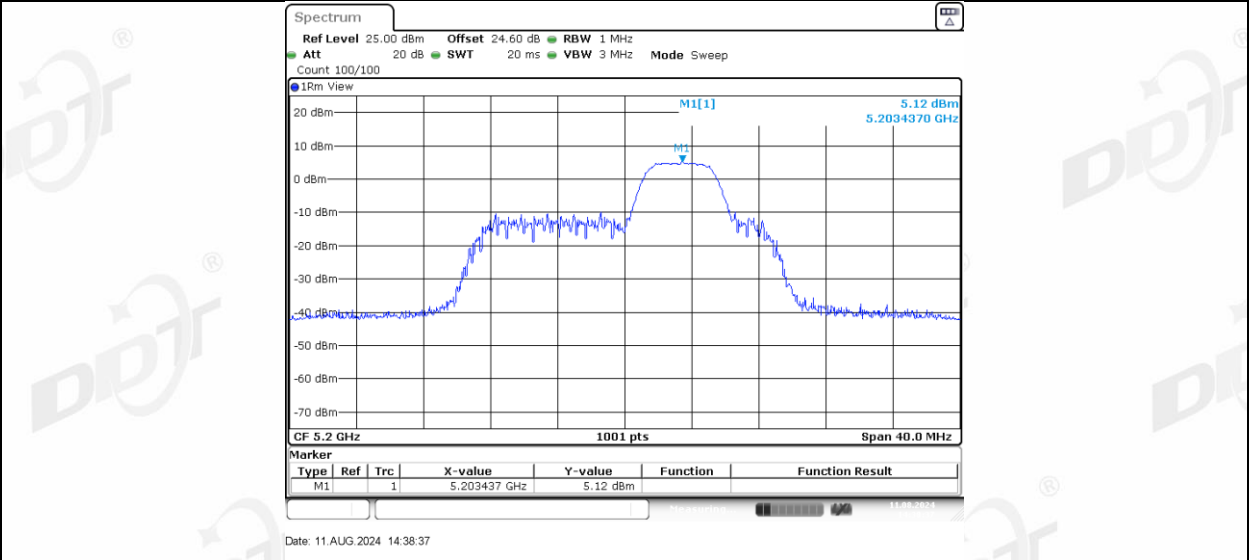
11AX20MIMO_Ant-3_5200_52Tone_RU40
