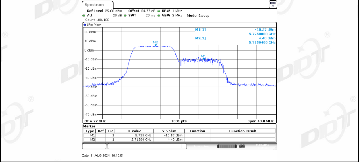
11AX20MIMO_Ant-3_5720_UNII-2C_106Tone_RU54
