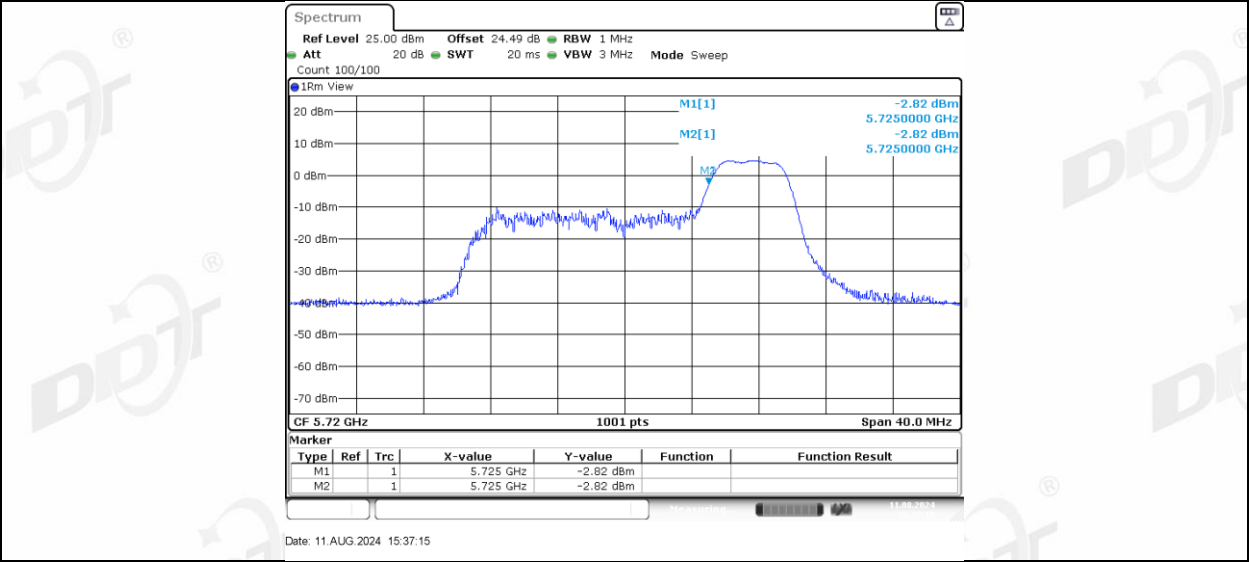
11AX20MIMO_Ant-3_5720_UNII-2C_106Tone_RU53
