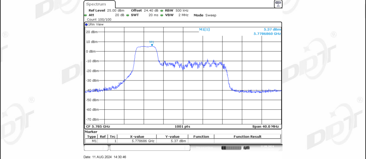
11AX20MIMO_Ant-3_5785_52Tone_RU39
