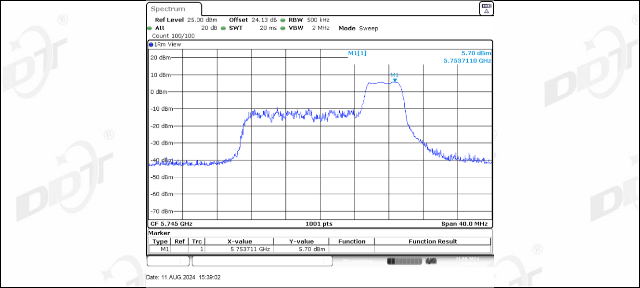
11AX20MIMO_Ant-1_5745_106Tone_RU53
