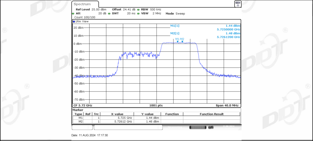
11AX20MIMO_Ant-3_5720_UNII-3_26Tone_RU0
