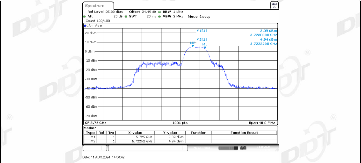
11AX20MIMO_Ant-3_5720_UNII-2C_52Tone_RU40
