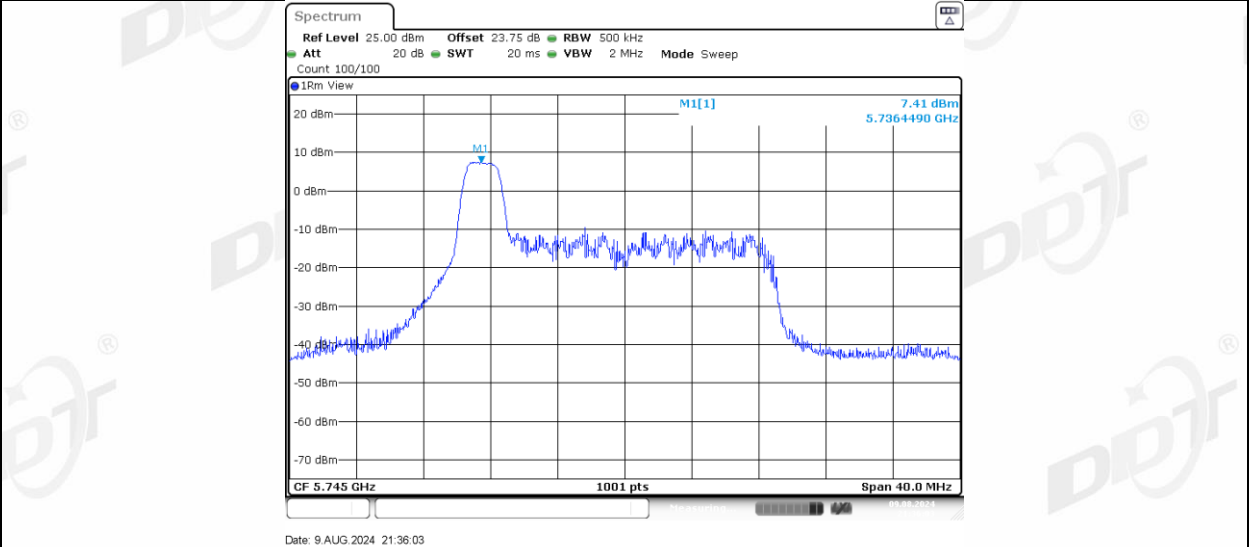
11AX20MIMO_Ant-1_5745_26Tone_RU4
