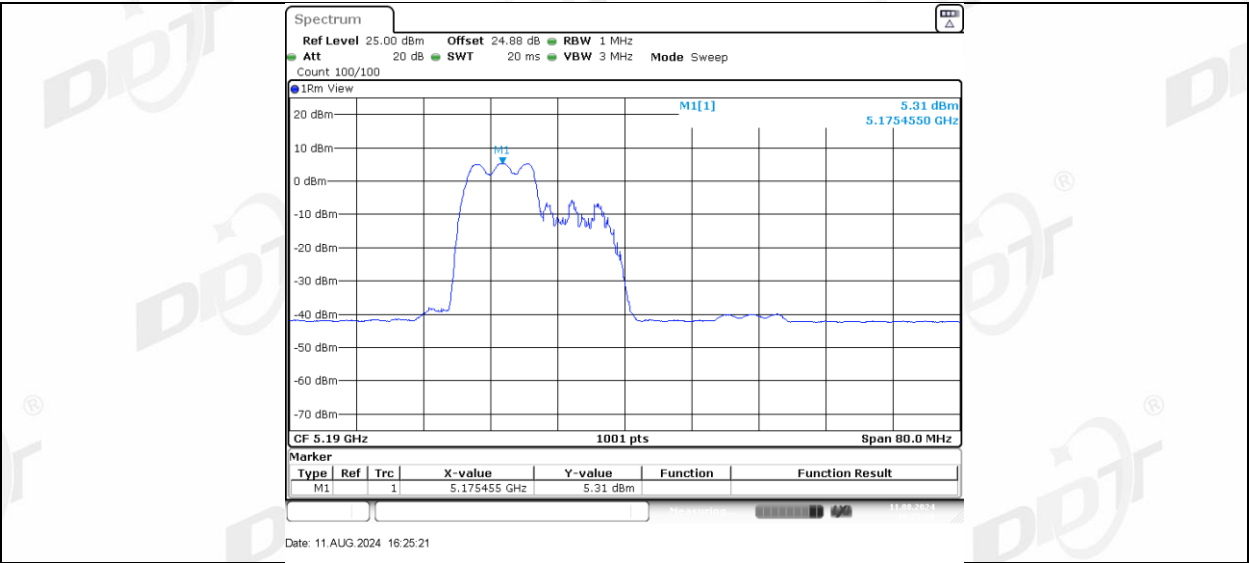
11AX40MIMO_Ant-3_5190_106Tone_RU56
