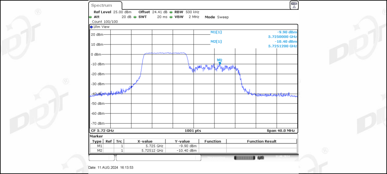
11AX20MIMO_Ant-1_5720_UNII-3_106Tone_RU54
