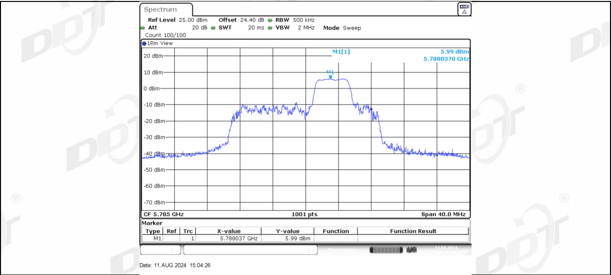
11AX20MIMO_Ant-3_5785_52Tone_RU40
