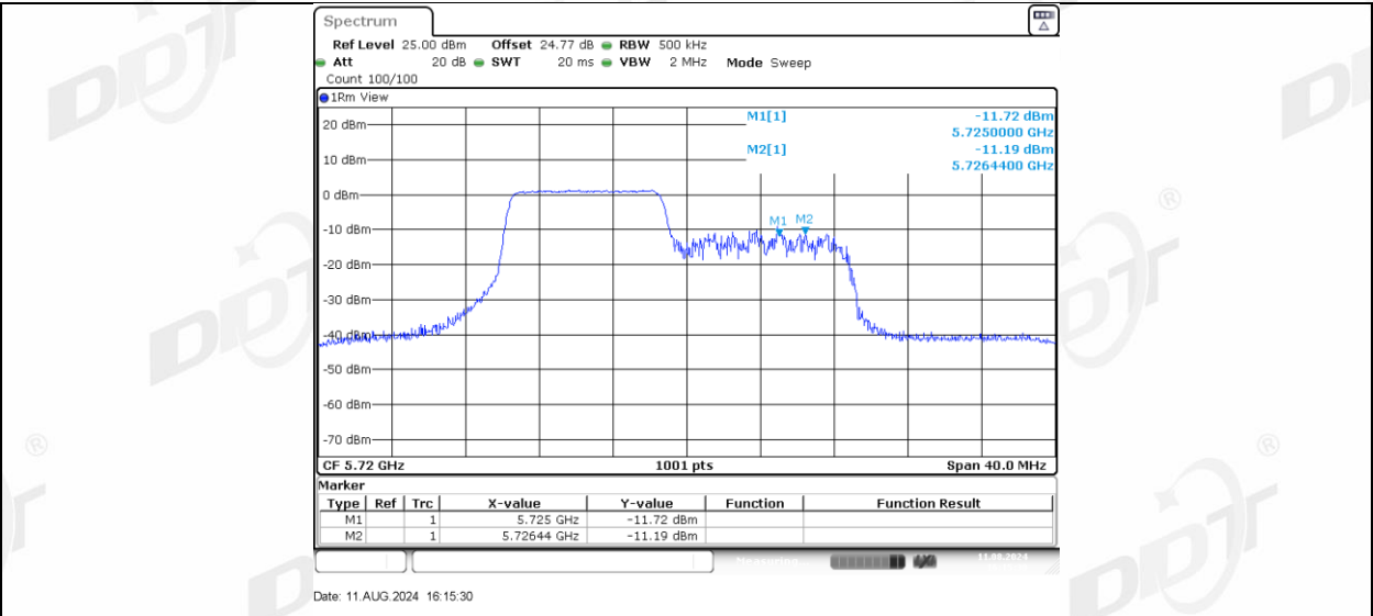
11AX20MIMO_Ant-3_5720_UNII-3_106Tone_RU54
