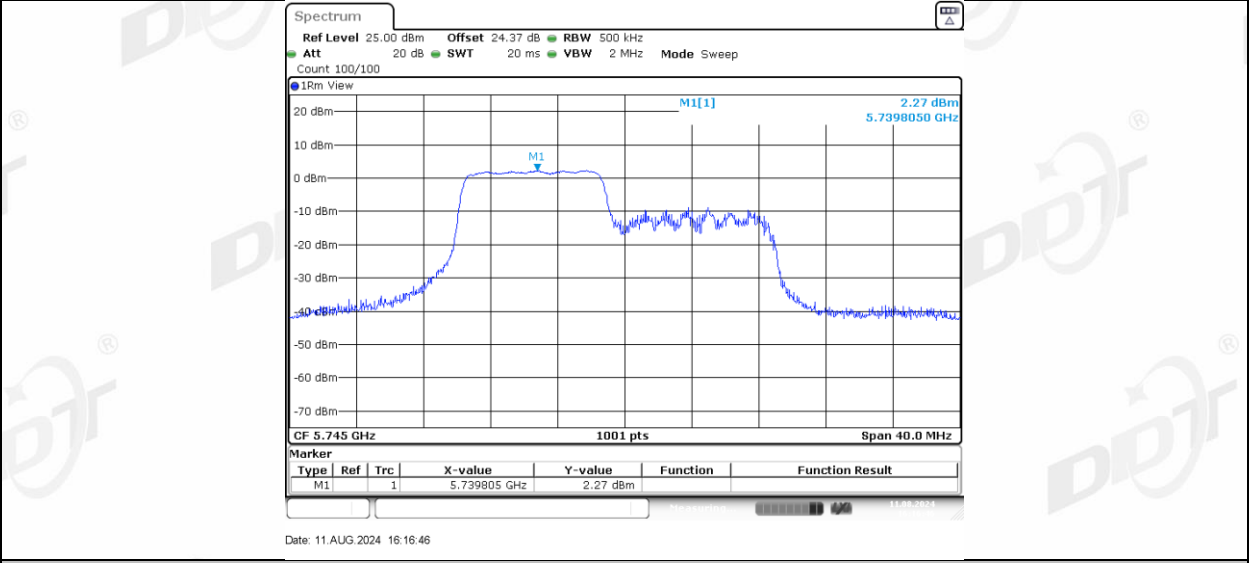
11AX20MIMO_Ant-1_5745_106Tone_RU54
