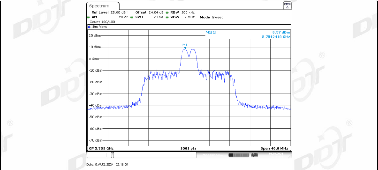
11AX20MIMO_Ant-3_5785_26Tone_RU8
