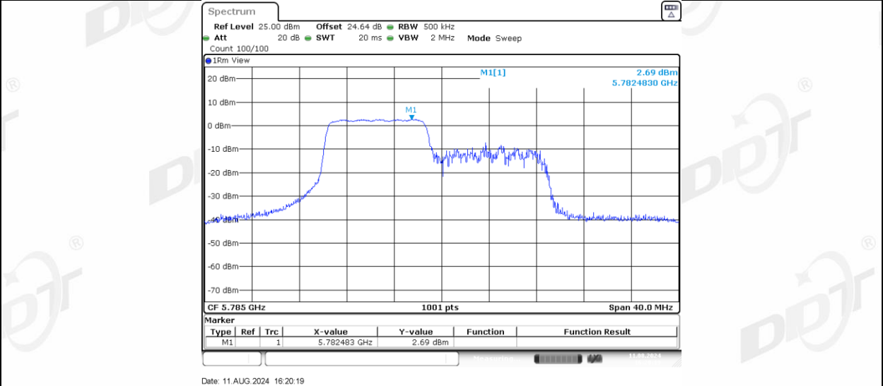
11AX20MIMO_Ant-3_5785_106Tone_RU54
