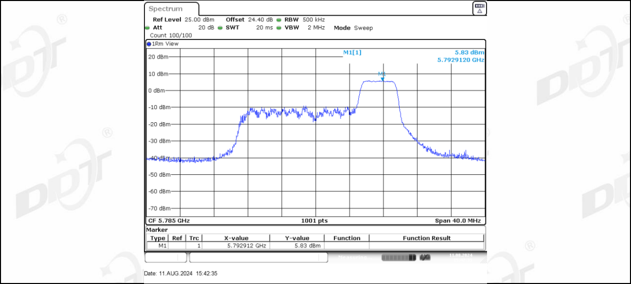
11AX20MIMO_Ant-3_5785_106Tone_RU53
