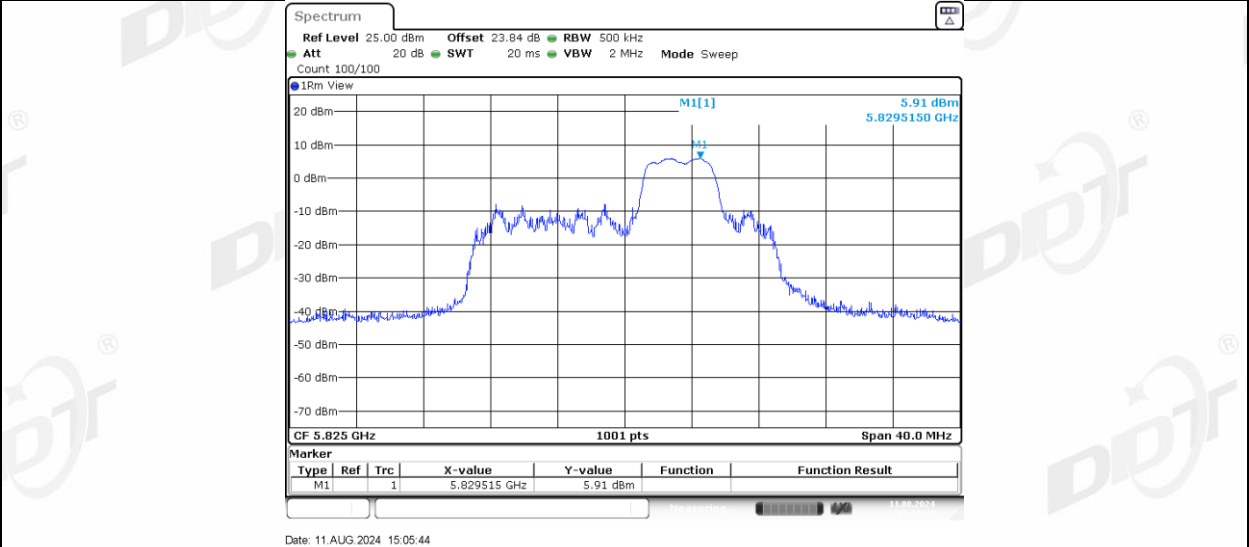
11AX20MIMO_Ant-1_5825_52Tone_RU40
