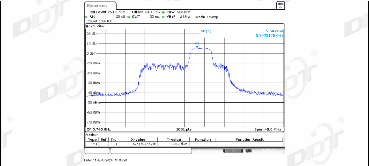
11AX20MIMO_Ant-1_5745_52Tone_RU40
