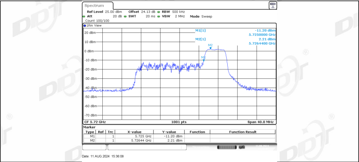
11AX20MIMO_Ant-1_5720_UNII-3_106Tone_RU53
