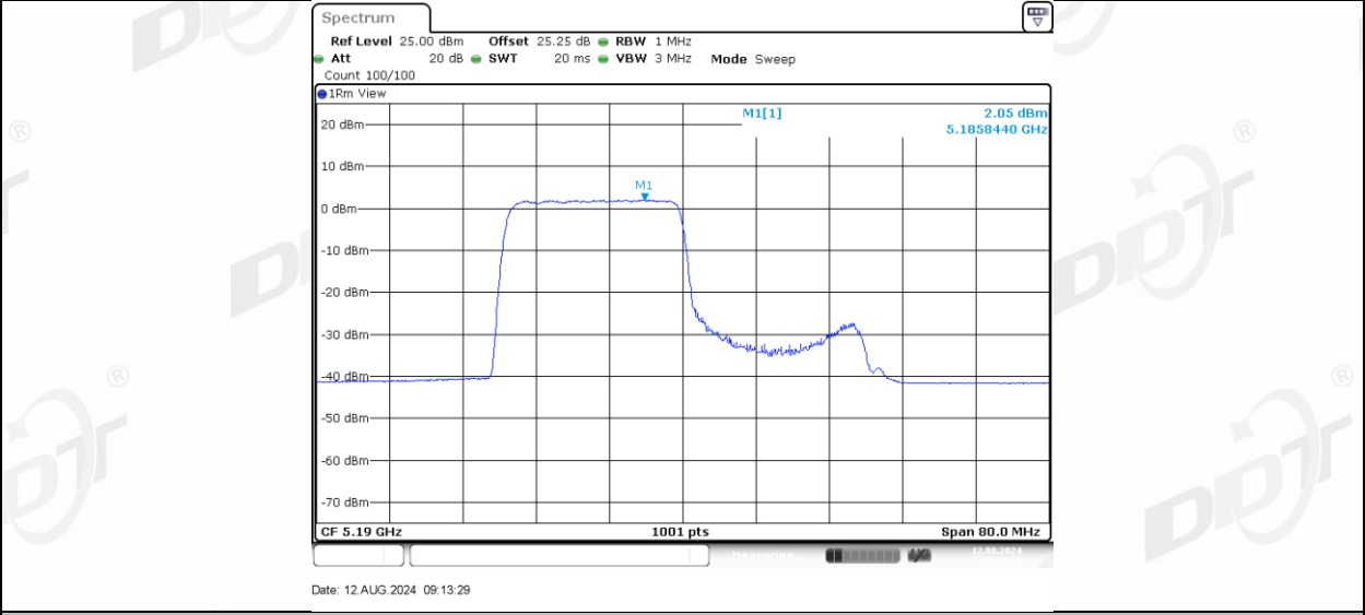
11AX40MIMO_Ant-3_5190_242Tone_RU62
