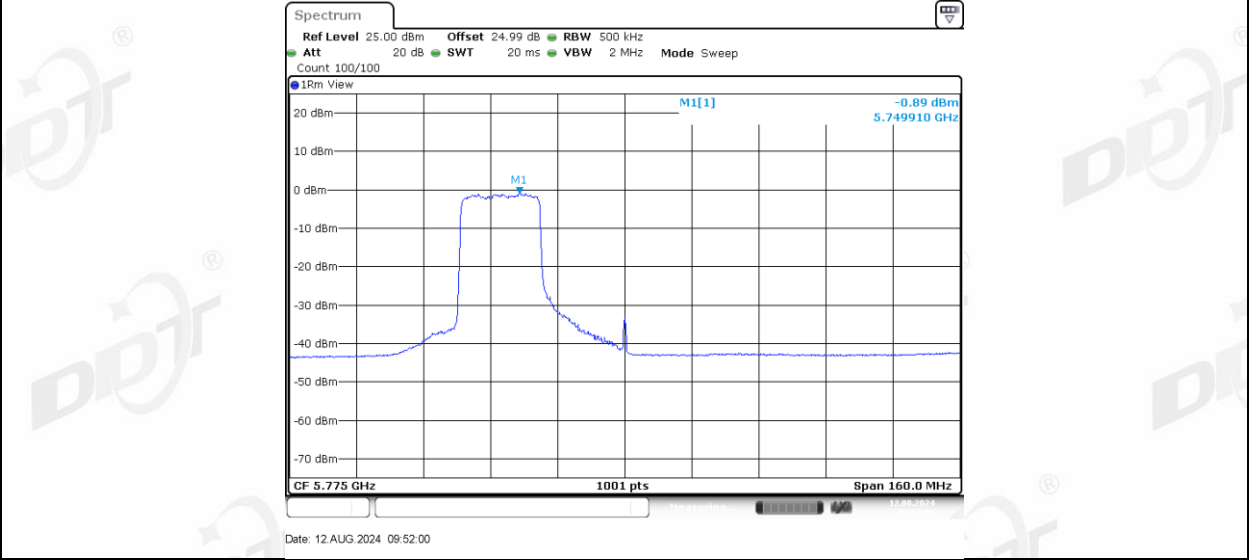
11AX80MIMO_Ant-3_5775_242Tone_RU64
