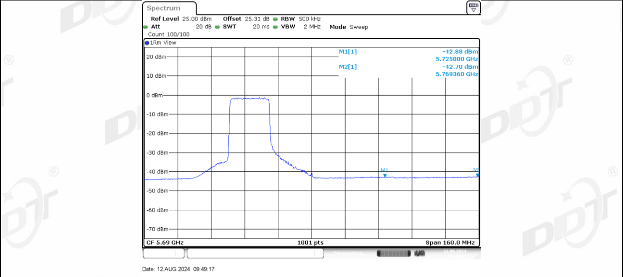
11AX80MIMO_Ant-3_5690_UNII-3_242Tone_RU64
