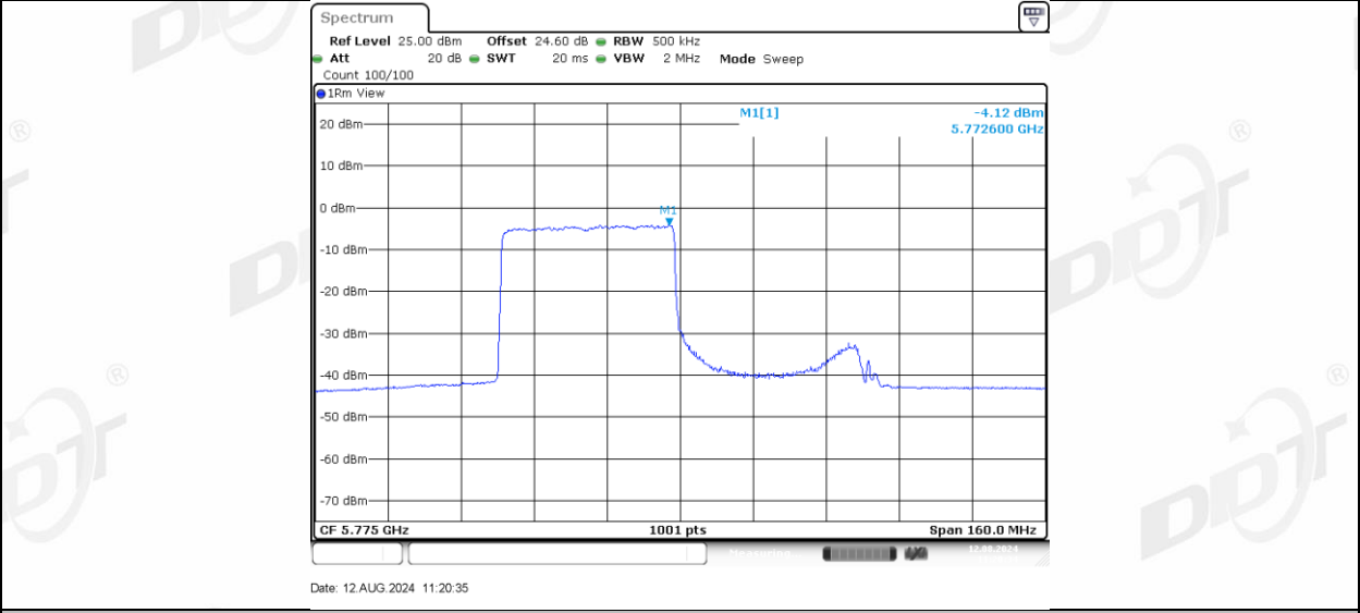
11AX80MIMO_Ant-1_5775_484Tone_RU66
