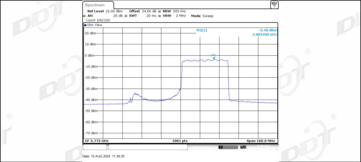
11AX80MIMO_Ant-3_5775_242Tone_RU61
