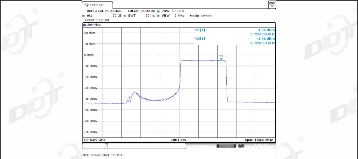
11AX80MIMO_Ant-3_5690_UNII-3_242Tone_RU61
