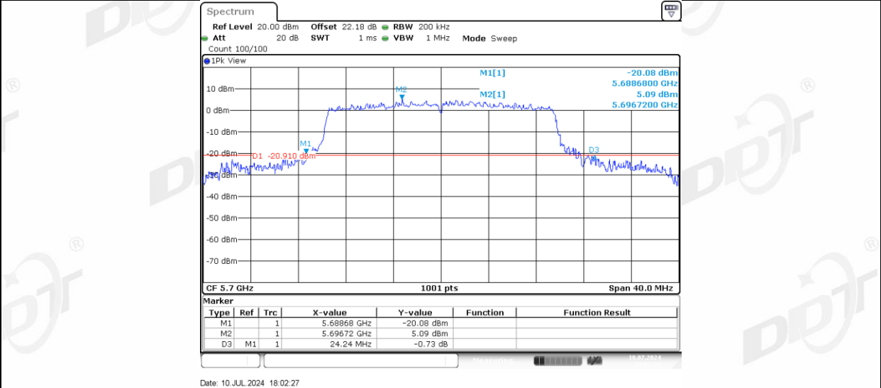
11AX20MIMO_Ant-3_5700
