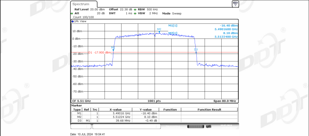
11AX40MIMO_Ant-3_5510
