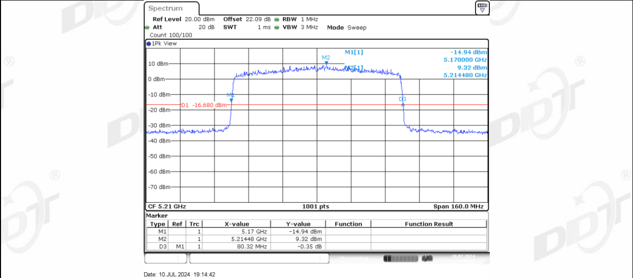
11AX80MIMO_Ant-3_5210
