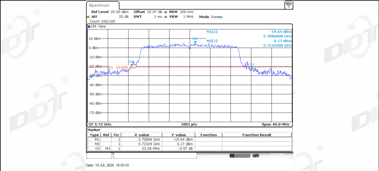
11AX20MIMO_Ant-3_5720
