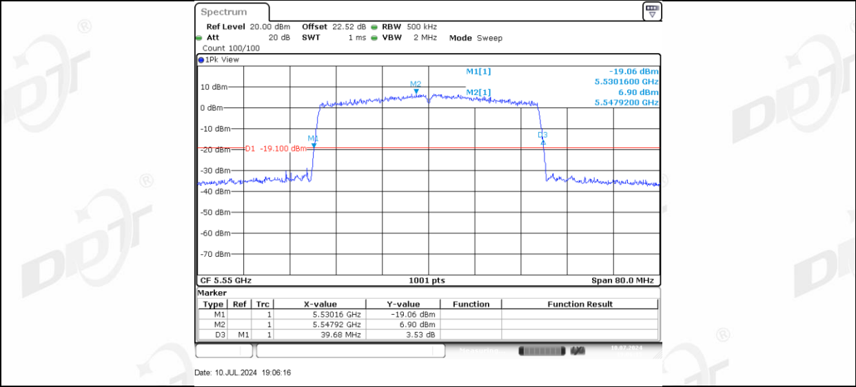
11AX40MIMO_Ant-3_5550
