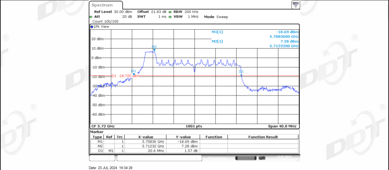
11AX20MIMO Ant-3 5720 26Tone_RU4
