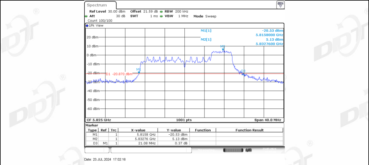
11AX20MIMO_Ant-3_5825_106Tone_RU53
