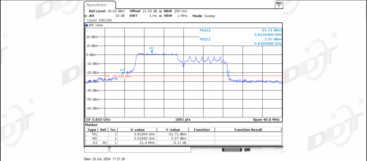
11AX20MIMO_Ant-3_5825_106Tone_RU54
