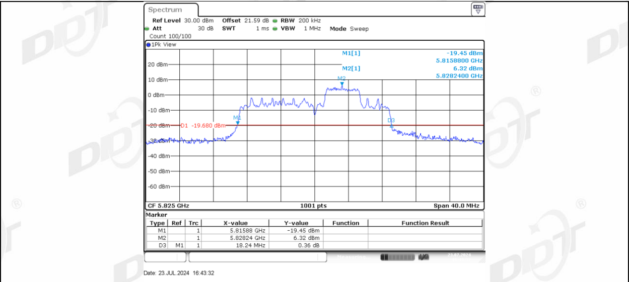
11AX20MIMO_Ant-3_5825_52Tone_RU40
