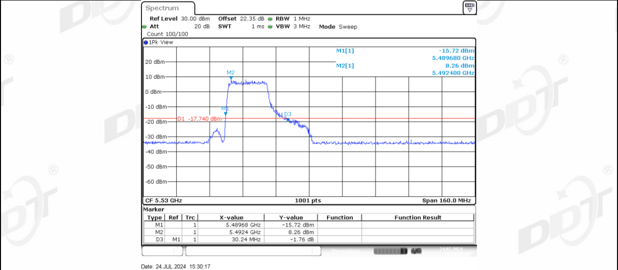
11AX80MIMO_Ant-3_5530_242Tone_RU64
