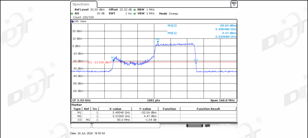
11AX80MIMO_Ant-3_5530_242Tone_RU61
