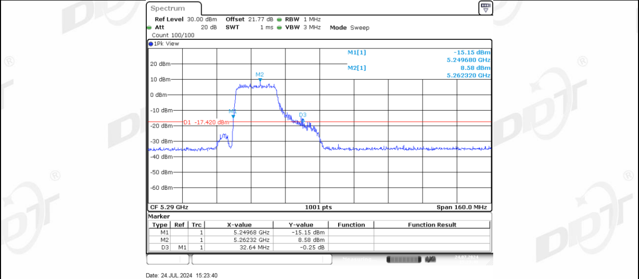
11AX80MIMO_Ant-1_5290_242Tone_RU64
