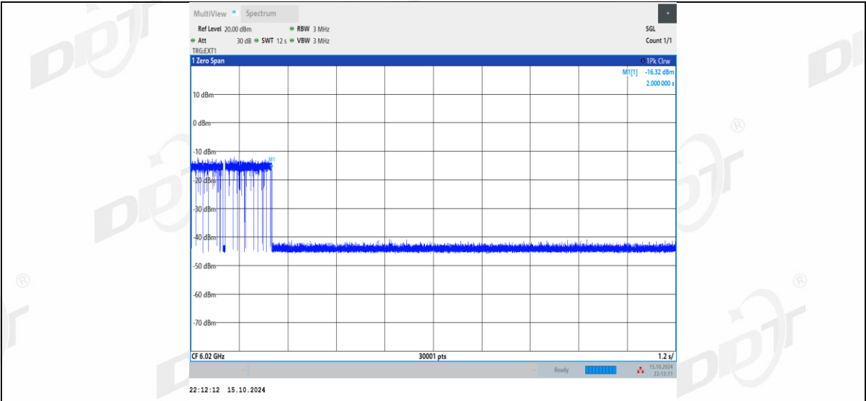
11AX80MIMO_Ant1_6465_Low_6430_OFF
