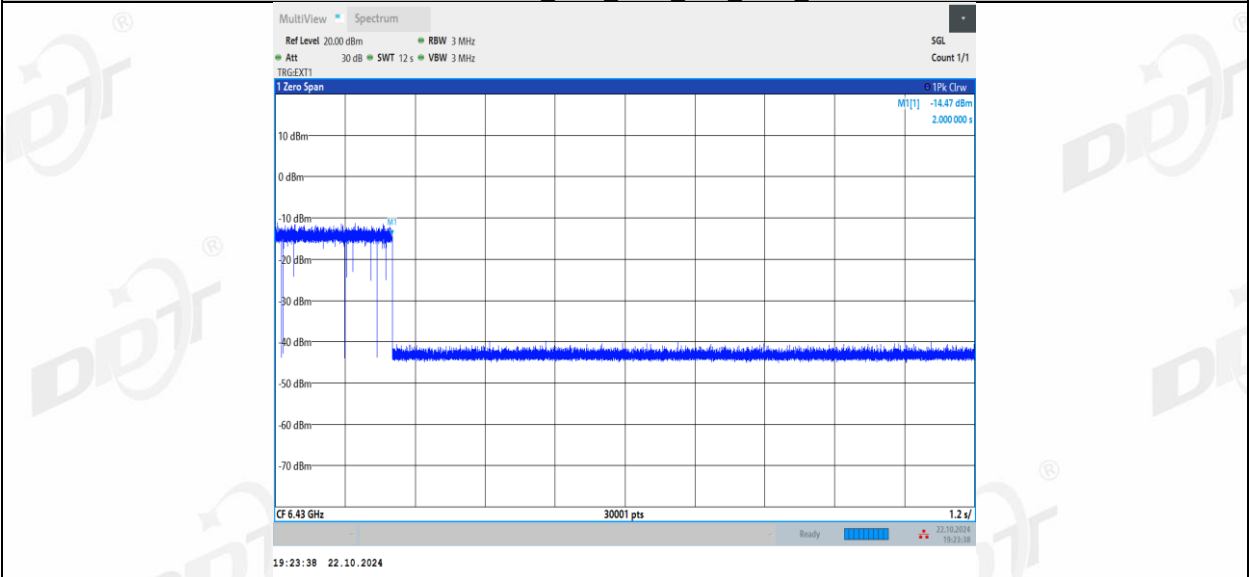
11AX80MIMO_Ant1_6465_Low_6430_Minimal
