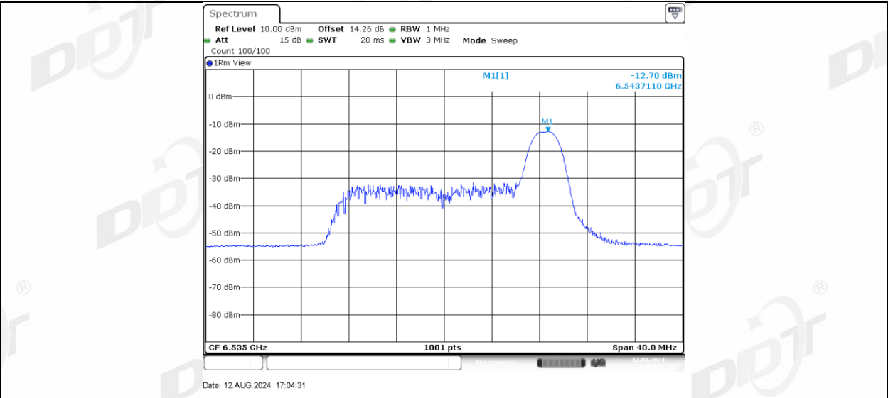
11AX20MIMO_Ant-1_6535_52Tone_RU37
