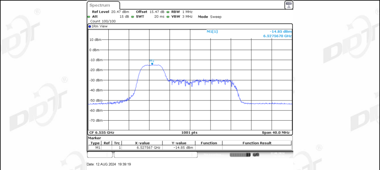
11AX20MIMO_Ant-1_6535_52Tone_RU39
