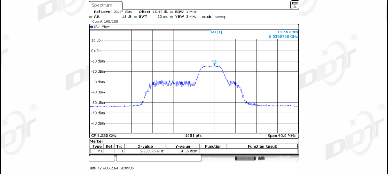
11AX20MIMO_Ant-1_6535_52Tone_RU40
