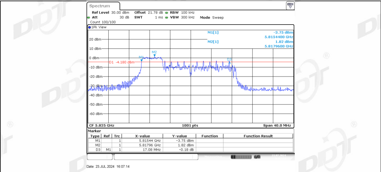
11AX20MIMO_Ant-1_5825_52Tone_RU39
