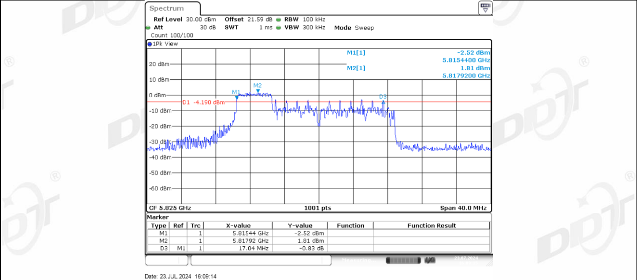
11AX20MIMO_Ant-3_5825_52Tone_RU39
