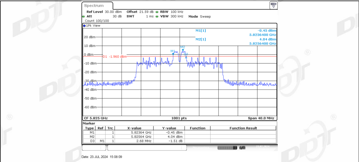
11AX20MIMO_Ant-3_5825_26Tone_RU8
