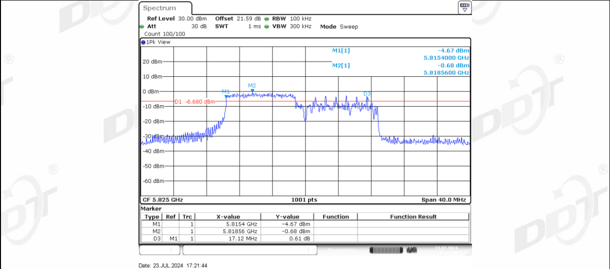
11AX20MIMO_Ant-3_5825_106Tone_RU54
