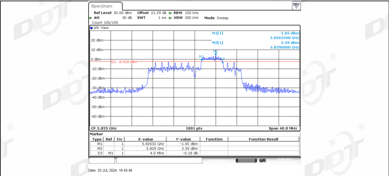
11AX20MIMO_Ant-3_5825_52Tone_RU40
