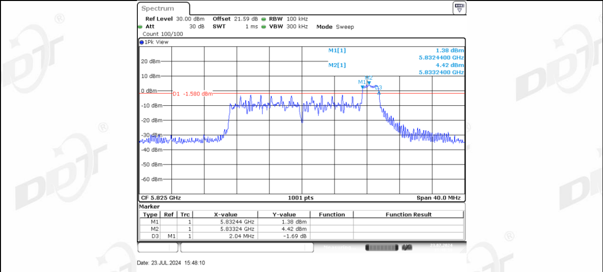
11AX20MIMO_Ant-3_5825_52Tone_RU37
