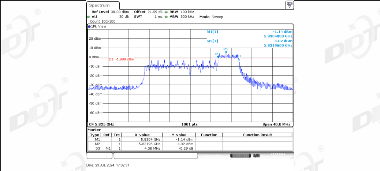
11AX20MIMO_Ant-3_5825_106Tone_RU53
