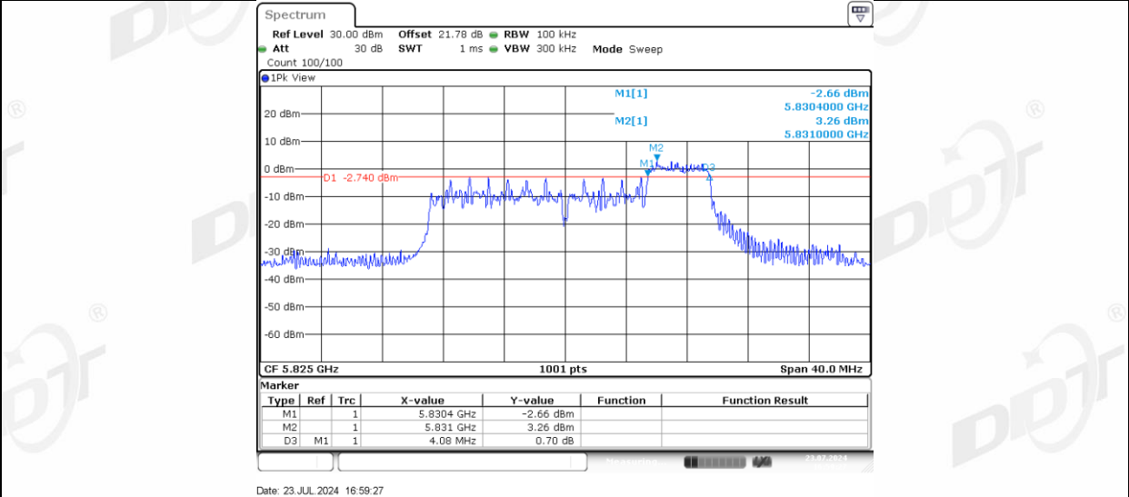
11AX20MIMO_Ant-1_5825_106Tone_RU53
