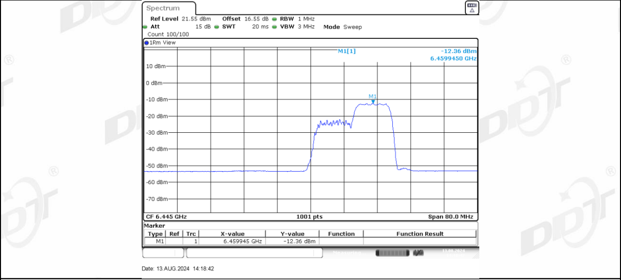
11AX40MIMO_Ant-3_6445_242Tone_RU61
