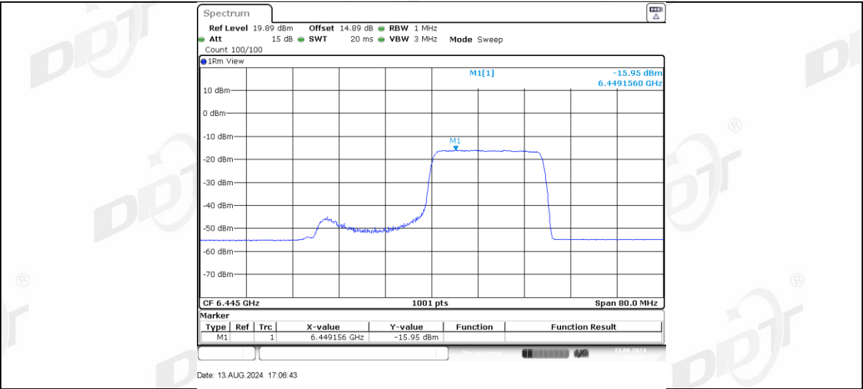
11AX40MIMO_Ant-3_6445_106Tone_RU53
