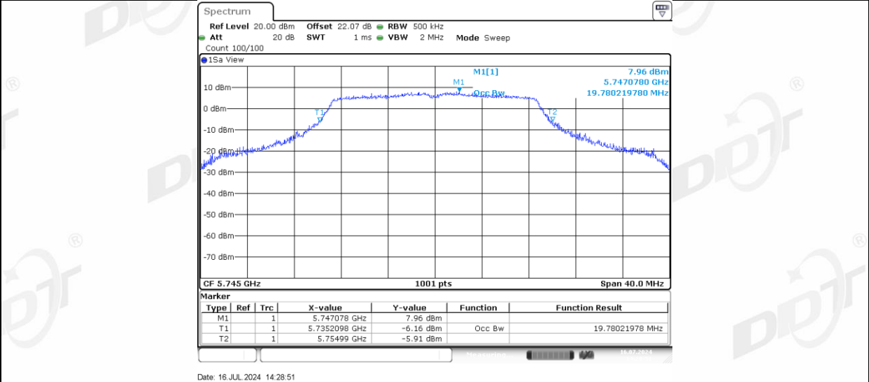
11AC20MIMO_Ant-3_5745
