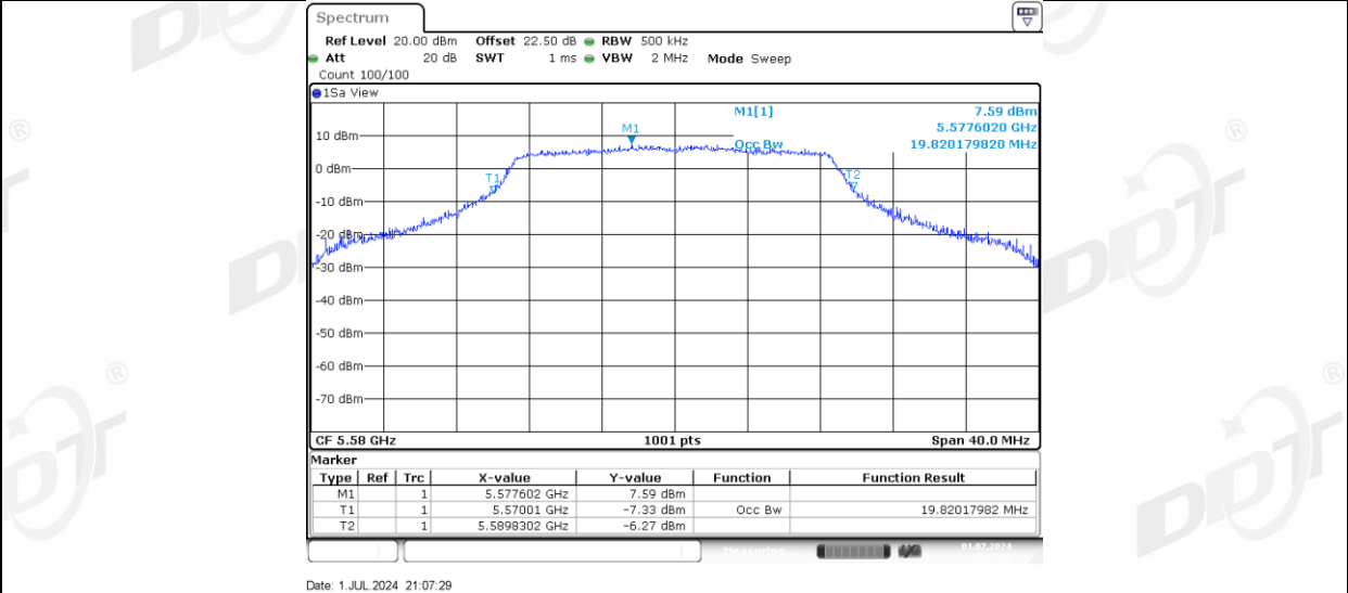
11AC20MIMO_Ant-3_5580
