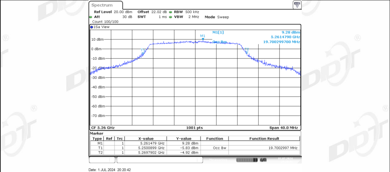
11N20MIMO_Ant-3_5260
