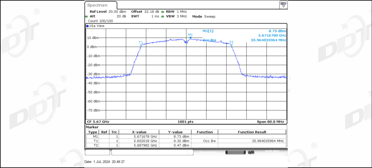
11N40MIMO_Ant-3_5670
