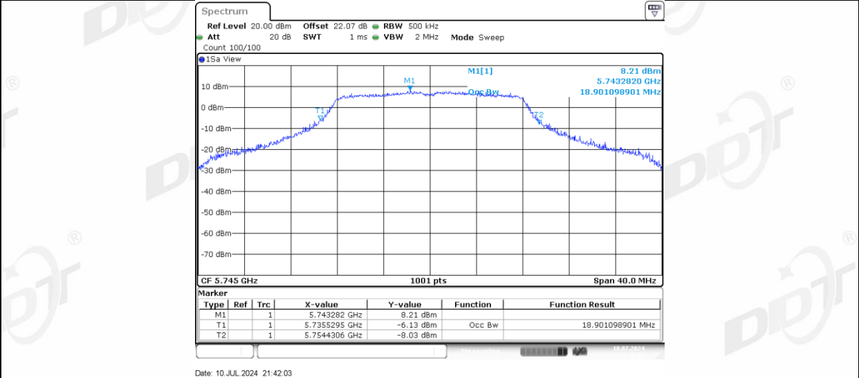
11A-CDD_Ant-3_5745
