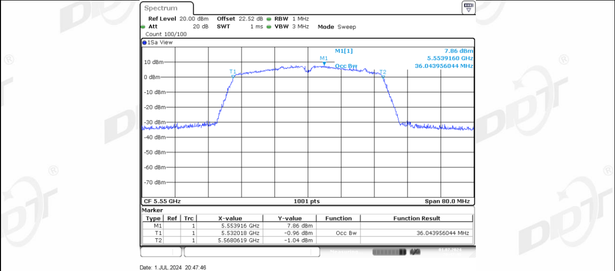
11N40MIMO_Ant-3_5550
