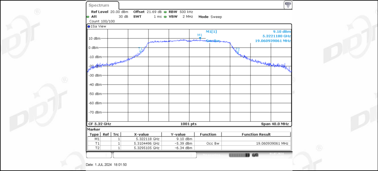
11A-CDD_Ant-3_5320
