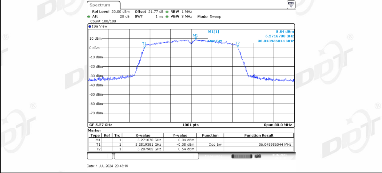
11N40MIMO_Ant-3_5270
