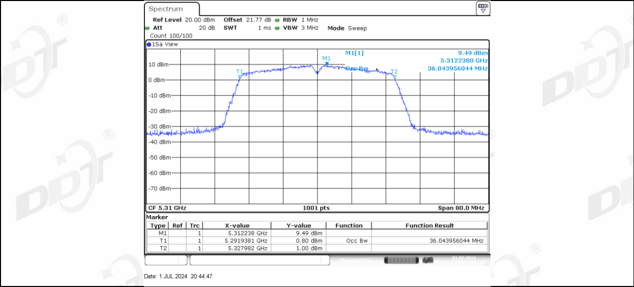
11N40MIMO_Ant-3_5310
