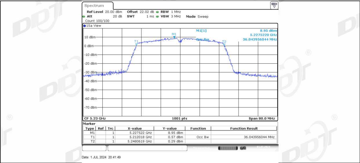
11N40MIMO_Ant-3_5230
