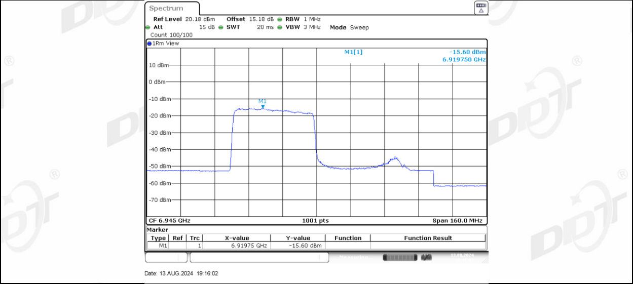
11AX80MIMO_Ant-3_6945_484Tone_RU66
