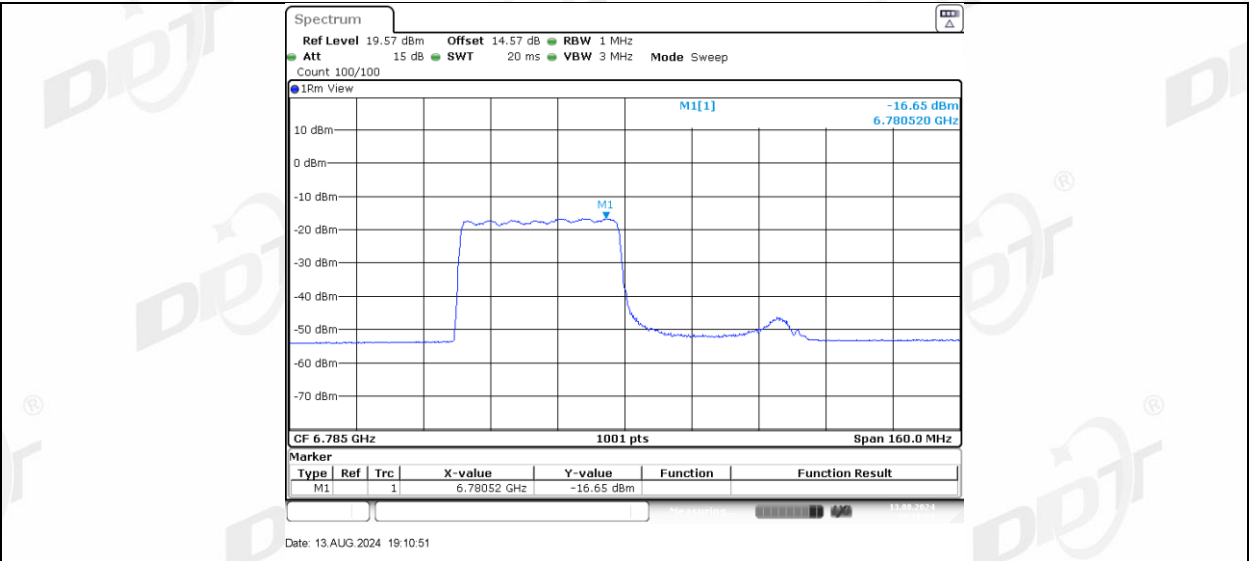
11AX80MIMO_Ant-1_6785_484Tone_RU66
