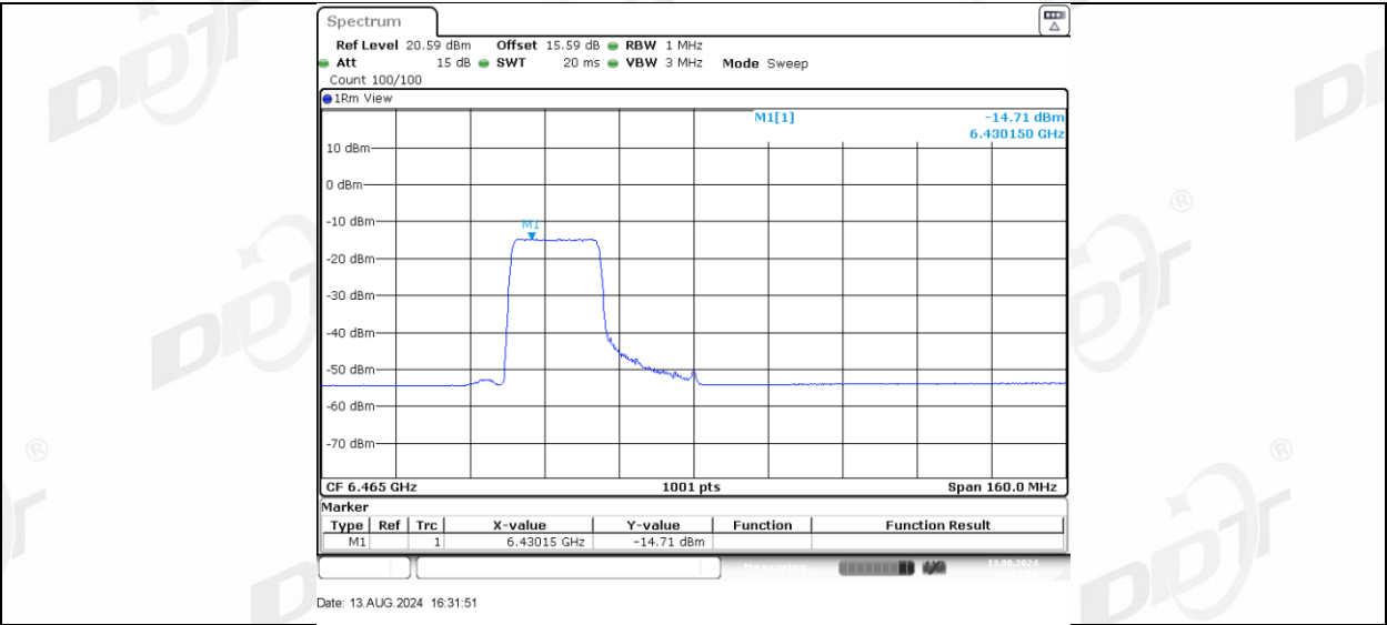
11AX80MIMO_Ant-3_6465_242Tone_RU64
