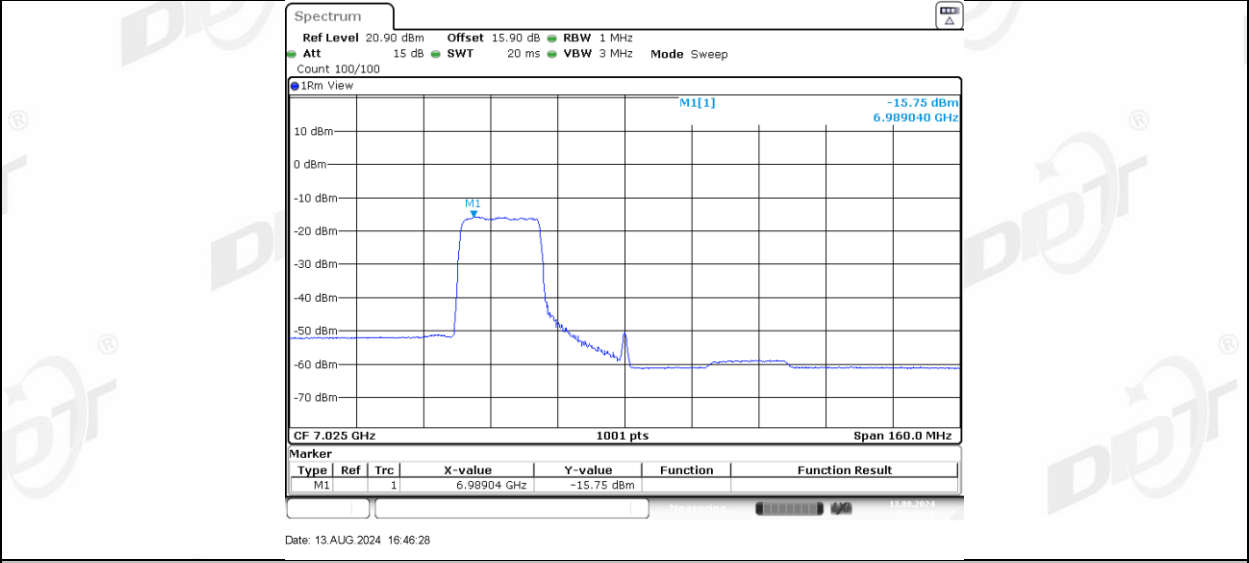
11AX80MIMO_Ant-3_7025_242Tone_RU64
