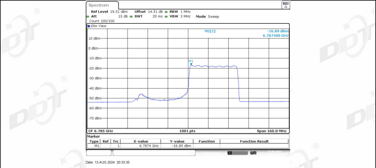
11AX80MIMO_Ant-3_6785_242Tone_RU61
