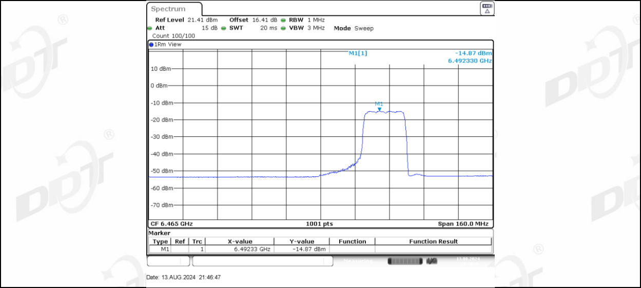
11AX80MIMO_Ant-3_6465_484Tone_RU65
