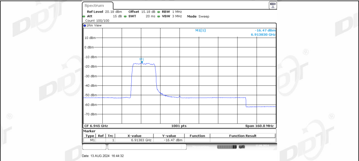
11AX80MIMO_Ant-3_6945_242Tone_RU64
