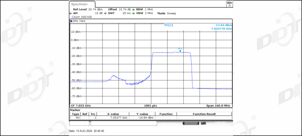
11AX80MIMO_Ant-3_7025_242Tone_RU61
