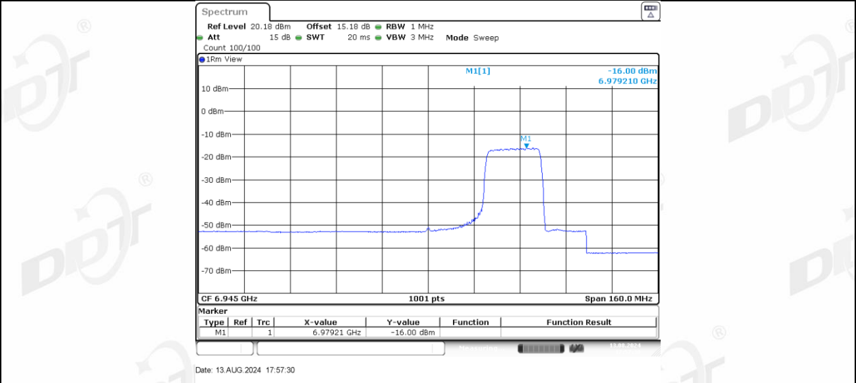
11AX80MIMO_Ant-3_6945_484Tone_RU65
