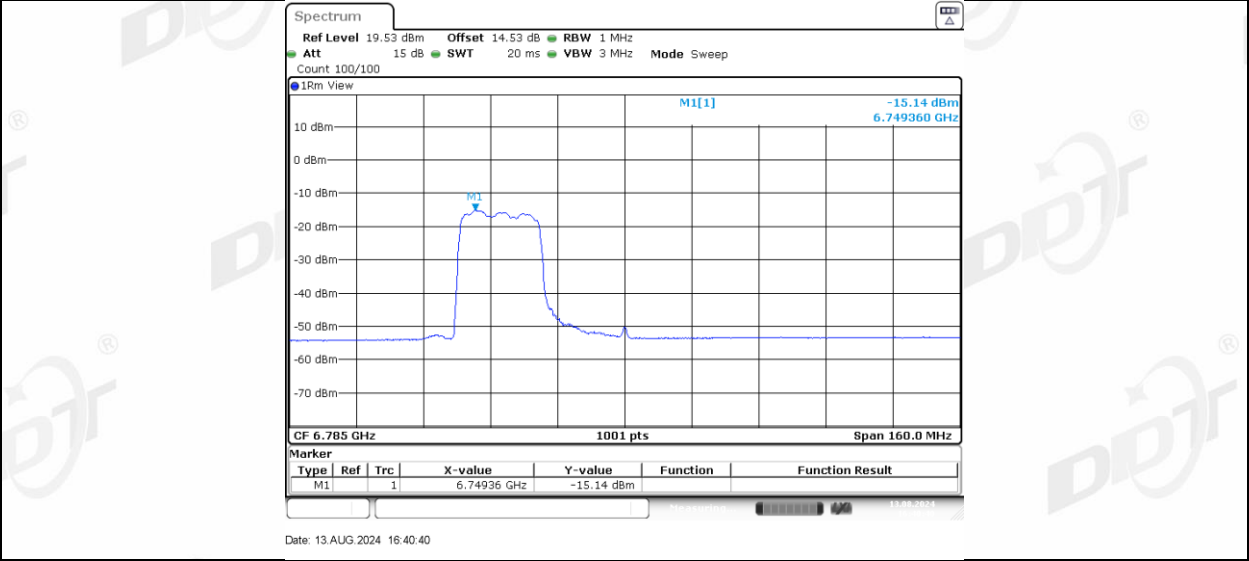
11AX80MIMO_Ant-3_6785_242Tone_RU64
