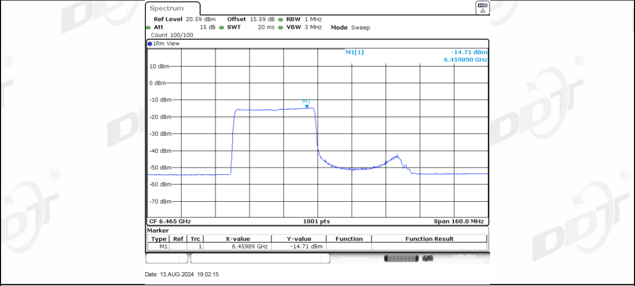
11AX80MIMO_Ant-3_6465_484Tone_RU66
