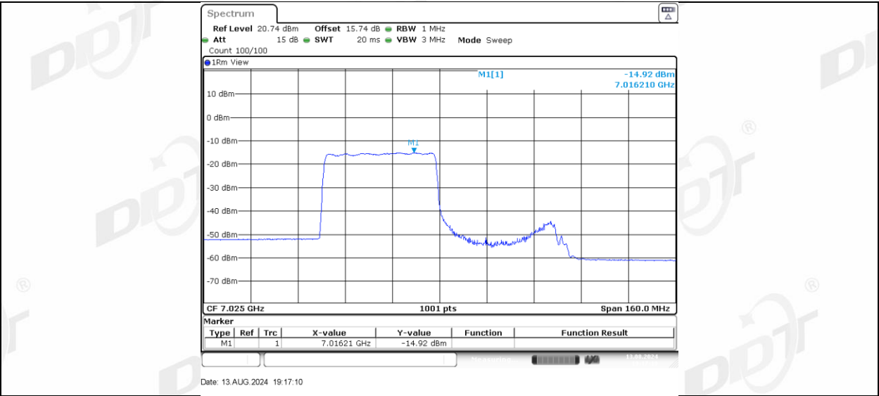
11AX80MIMO_Ant-1_7025_484Tone_RU66
