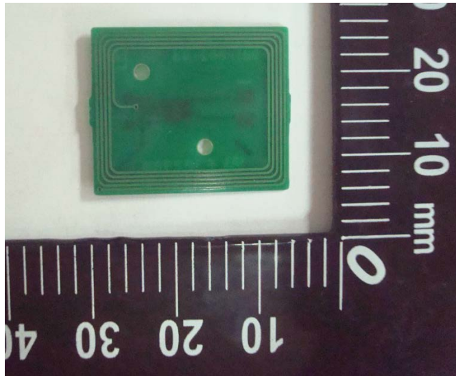
NFC (Back)
