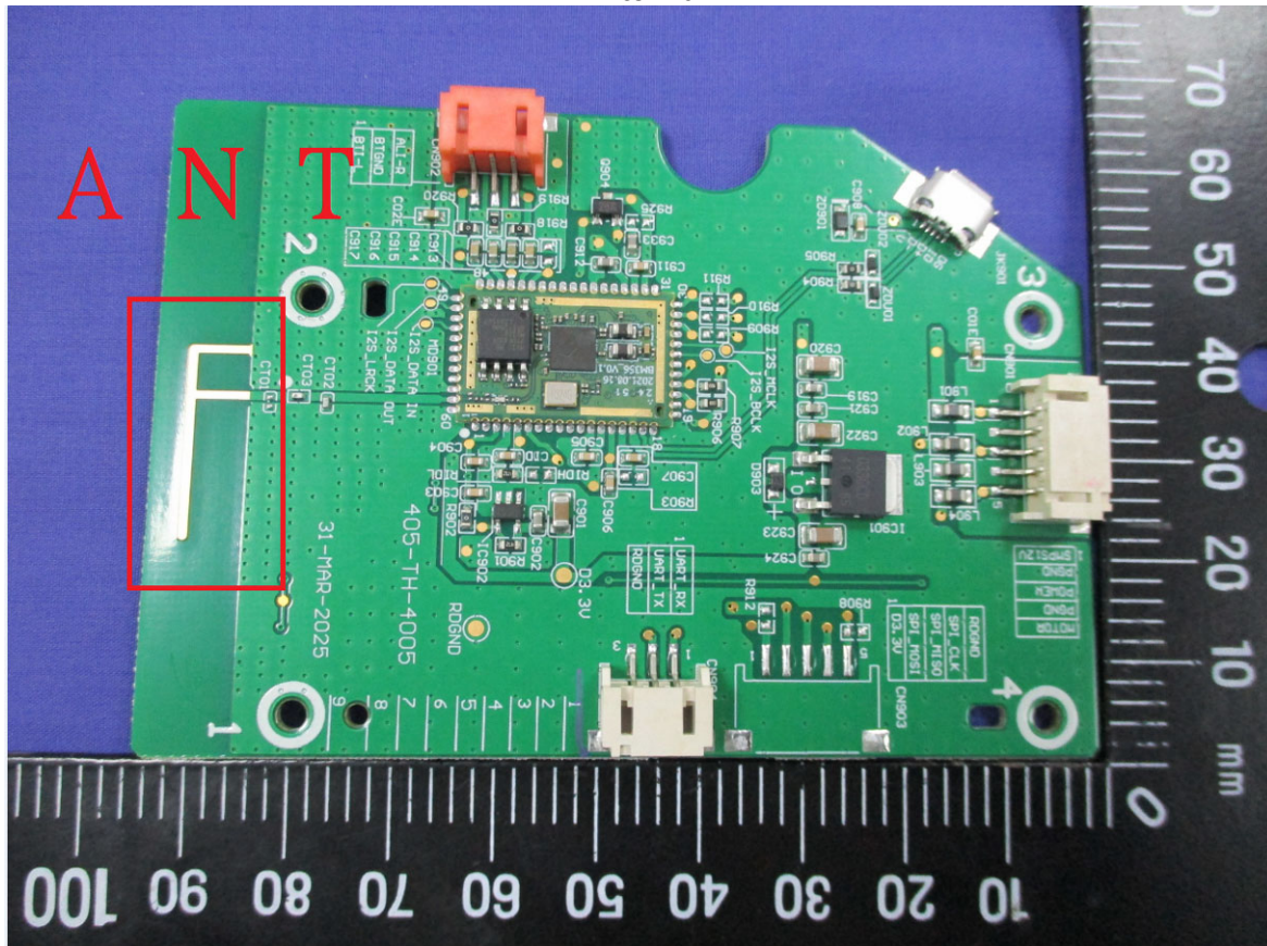
Antenna
