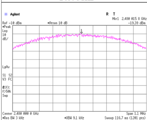
2480 MHz
