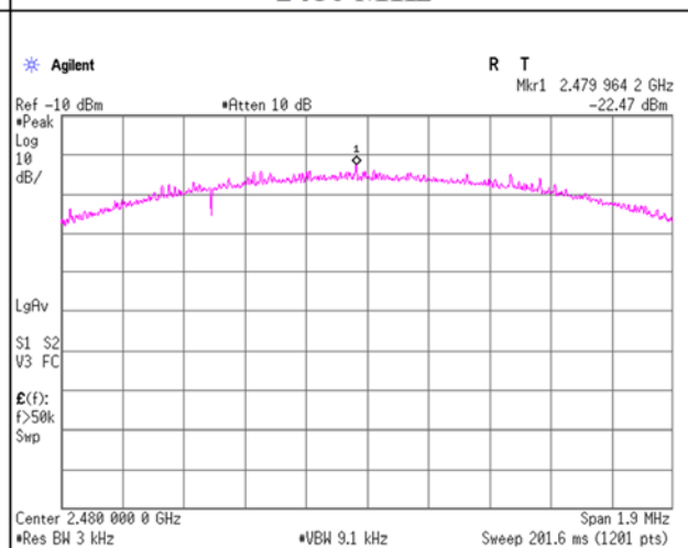
2480 MHz
