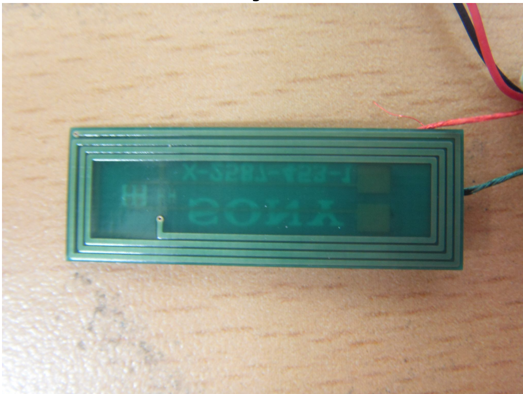
NFC Tag Antenna
