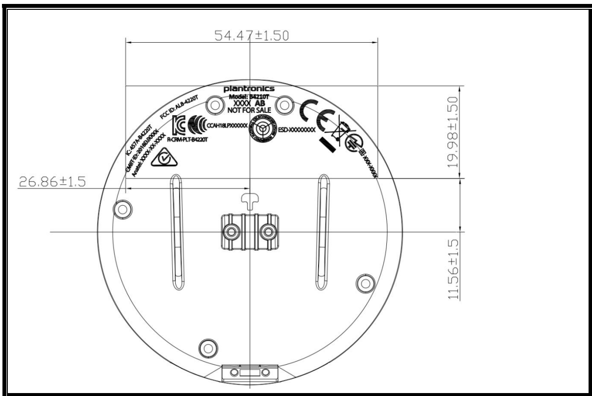
铭牌（标贴）
