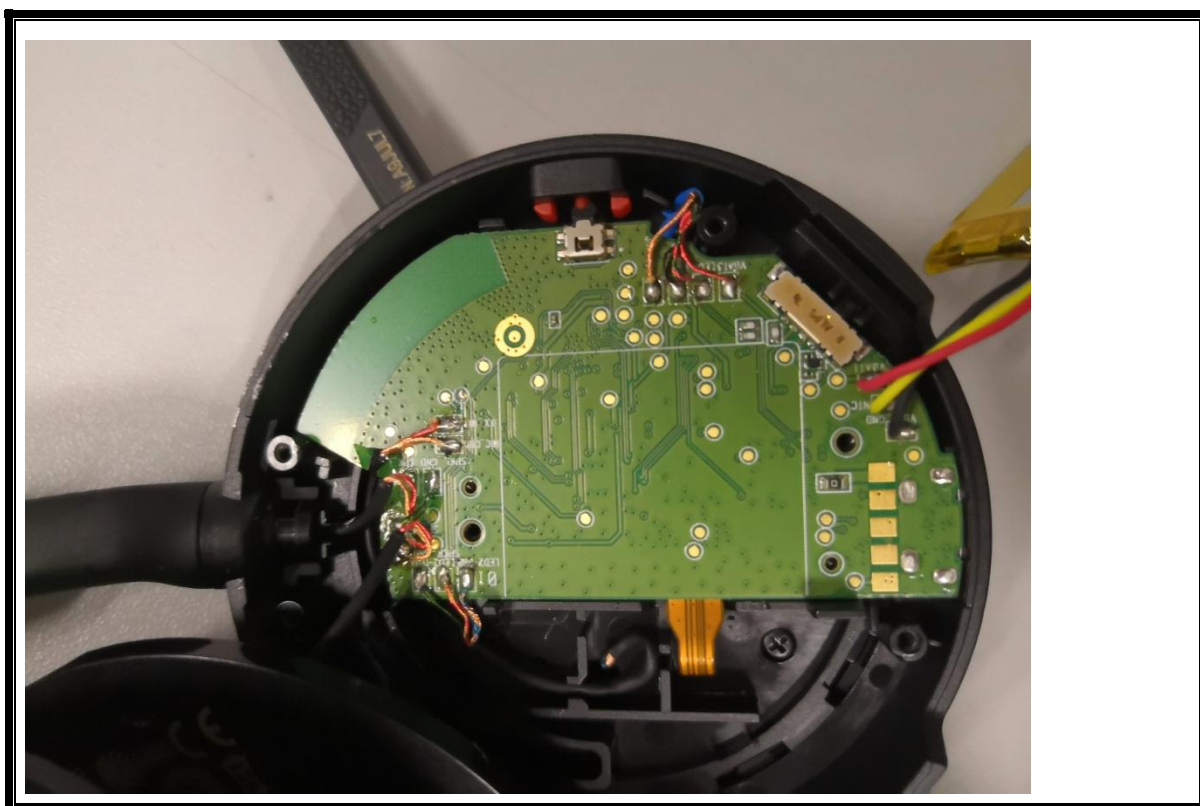
内部主板反面照片（去掉屏蔽罩放在旁边）
