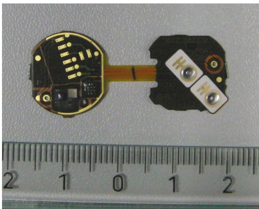
Left PCBA Top
