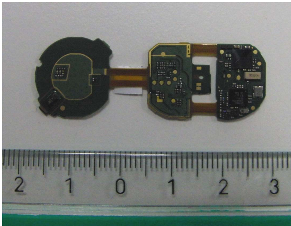
Right PCBA Bottom
