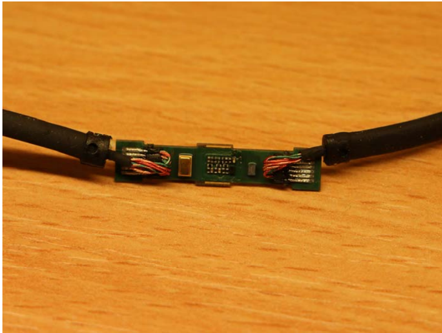
Inline PCBA Bottom
