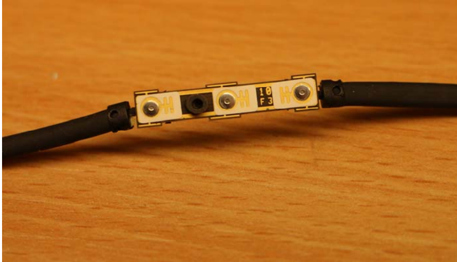
Inline PCBA Top
