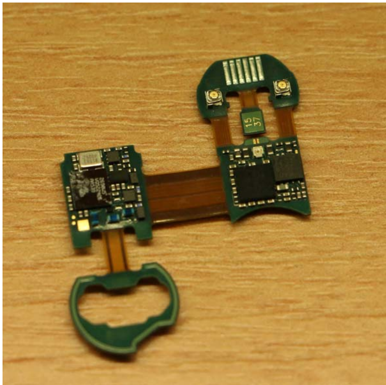
Right PCBA Bottom
