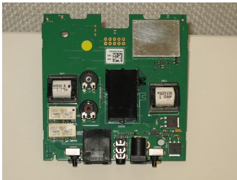
PCBA Bottom
