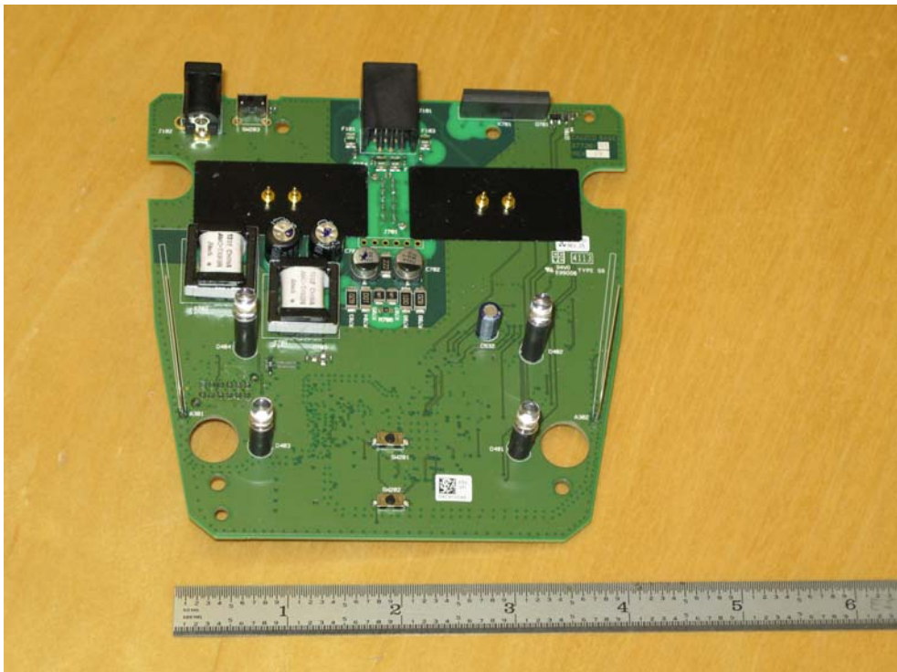
PCB Top
