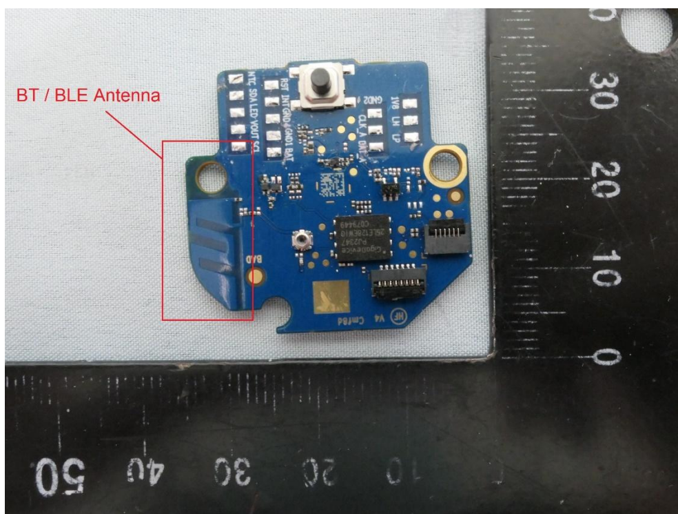
(18) EUT Photo (PBF620)
