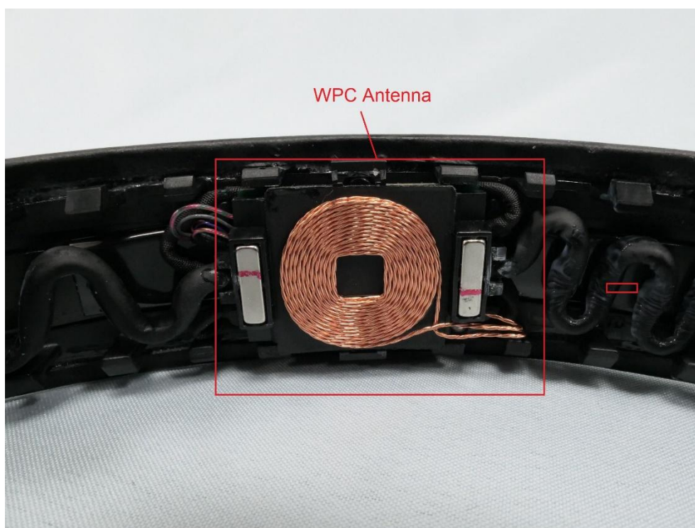
(16) EUT Photo (PBF620)
