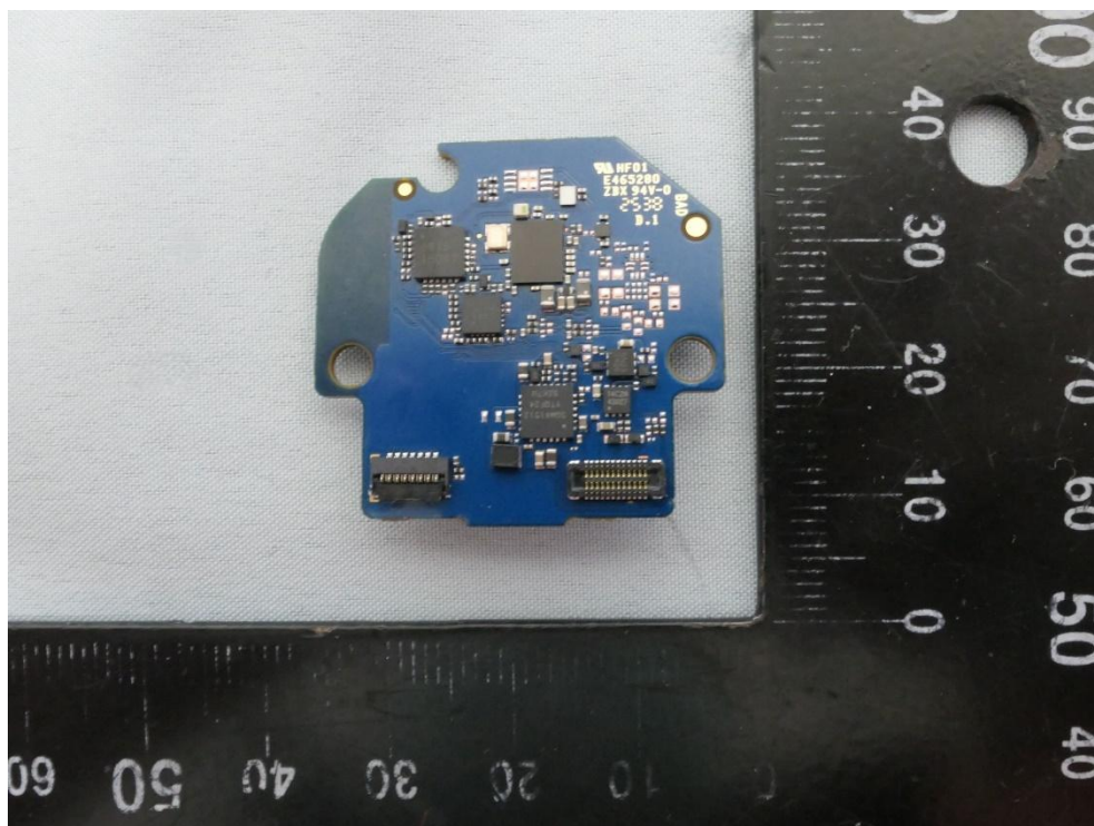
(20) EUT Photo (PBF620)
