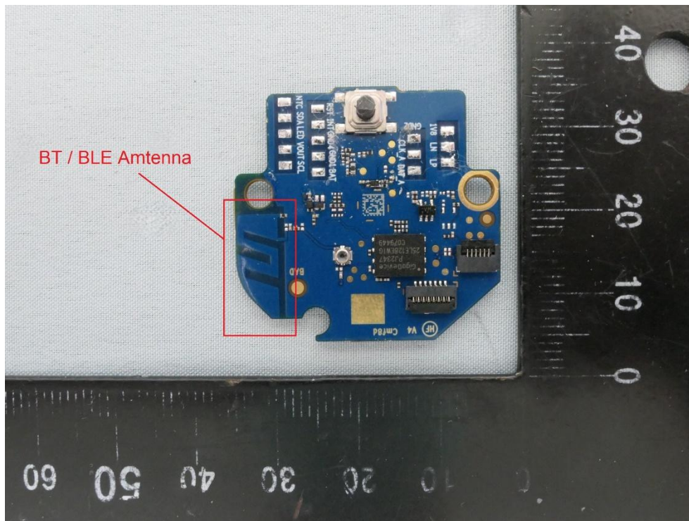
(8) EUT Photo (PBF620F)
