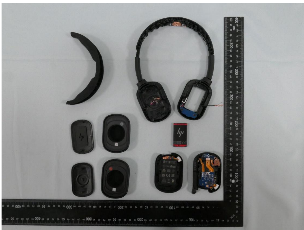
(12) EUT Photo (PBF620)
