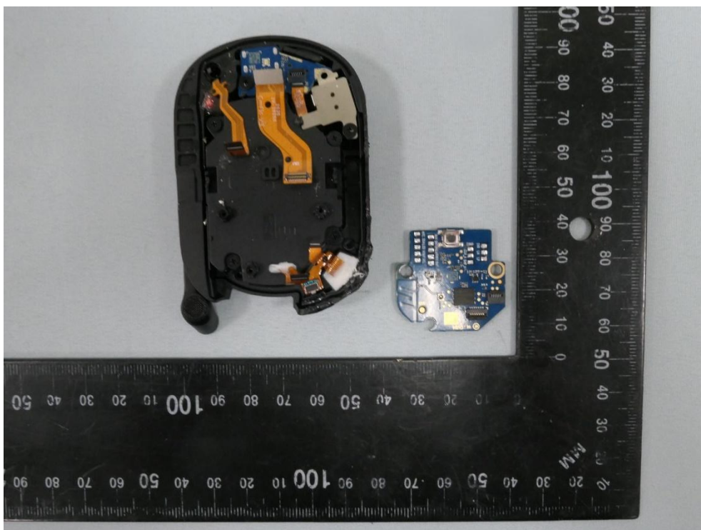
(6) EUT Photo (PBF620F)
