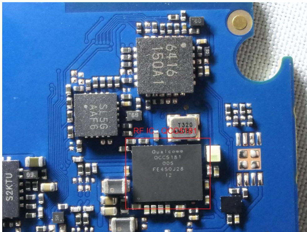
(22) EUT Photo (PBF620)
