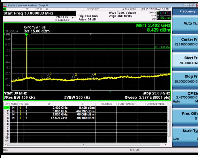
Mode 2 CH00(2402MHz)
