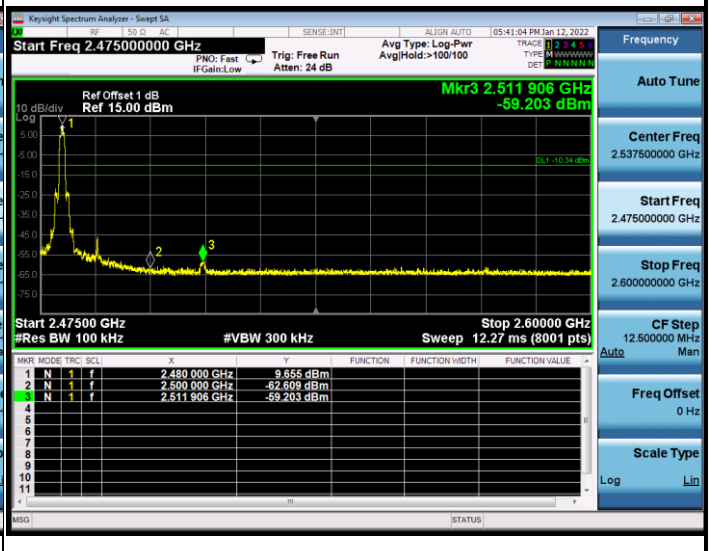
Mode 3 CH78(2480MHz)
