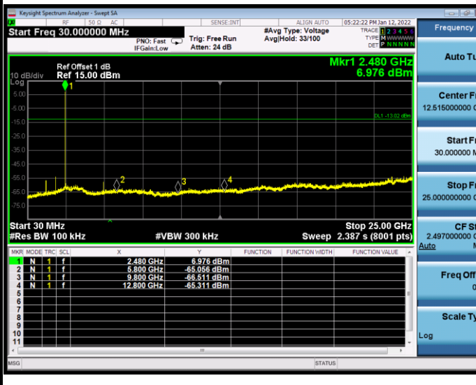
Mode 3 CH78(2480MHz)
