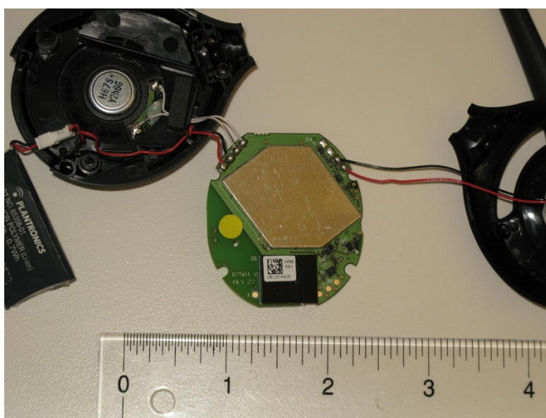
PCBA Bottom
