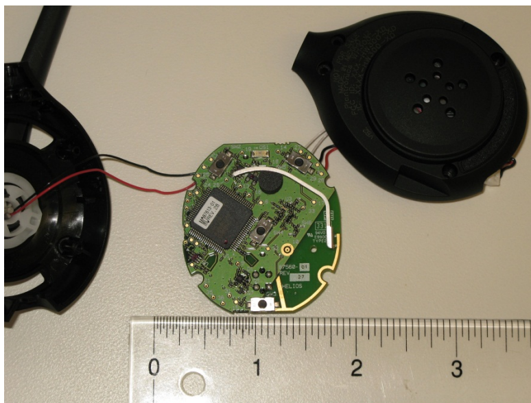
PCBA Top
