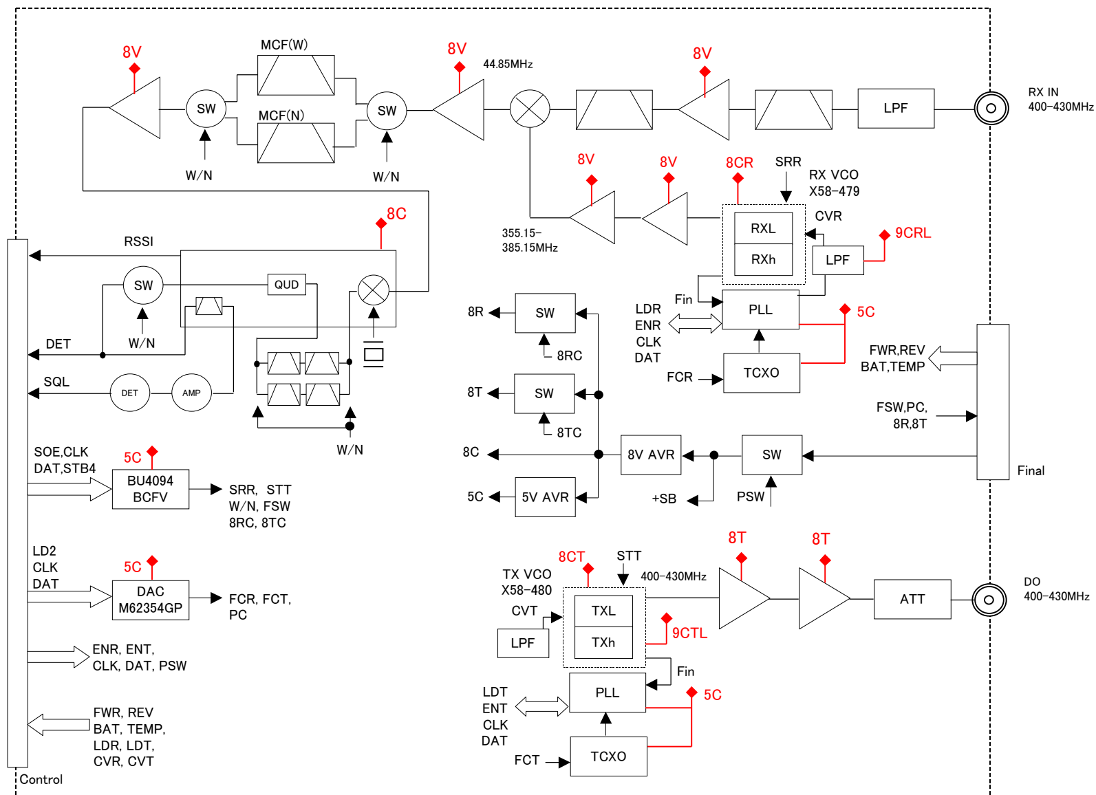
TKR-850K3 TX-RX unit (X57-6270-11): TX-RX
