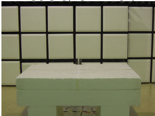
FCC_15_247_SRD_System_RC-P10DX-TUHH_Setup
