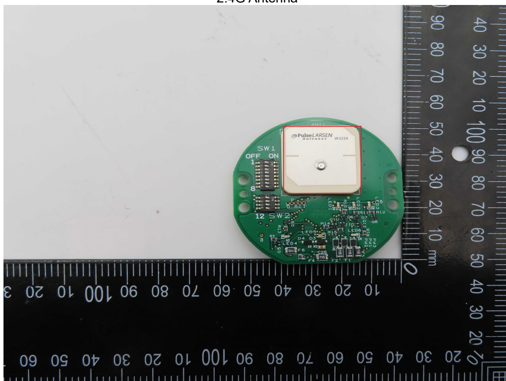
2.4G Antenna
