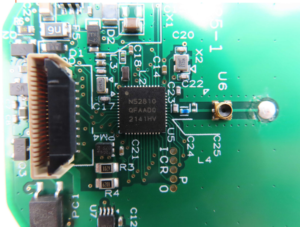
2.4G Antenna
