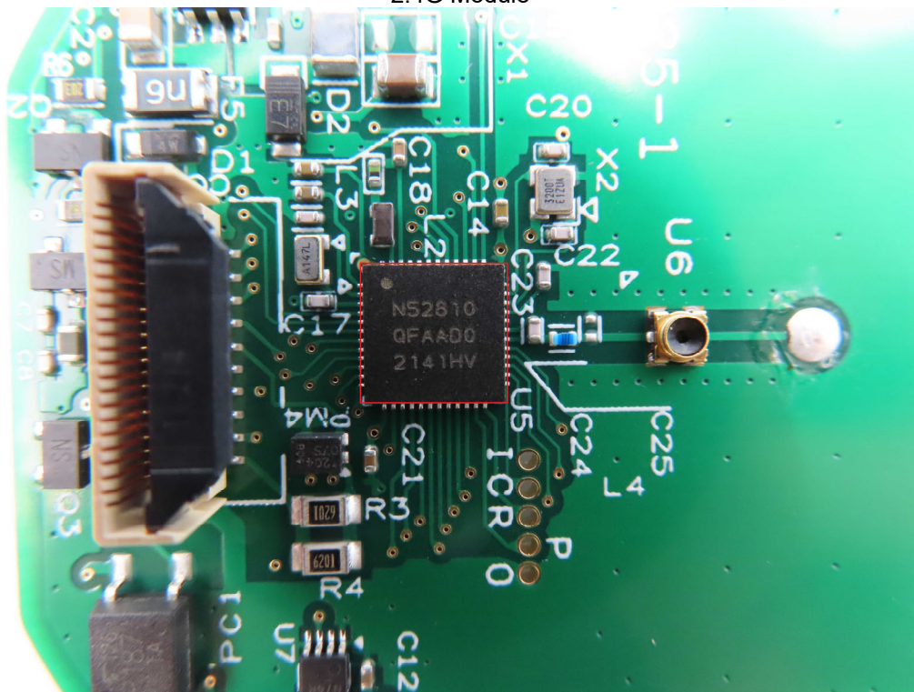
2.4G Module
