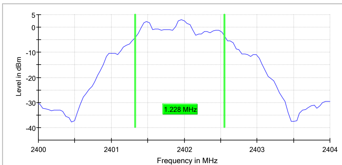
BLE_2M_Ant1_2402
