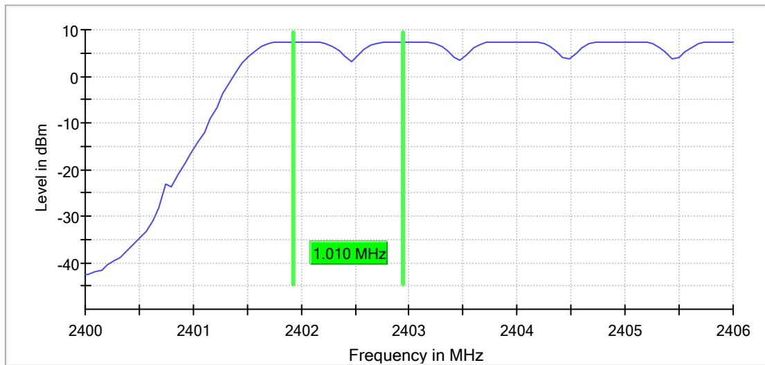
3DH5_Ant1_Hop
