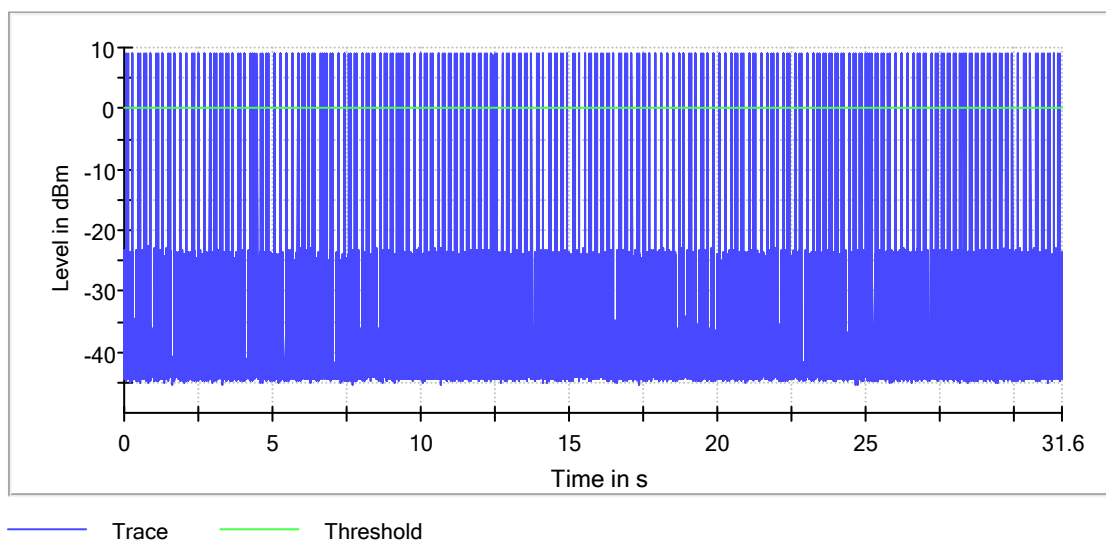
DH1_Ant1_Hop
