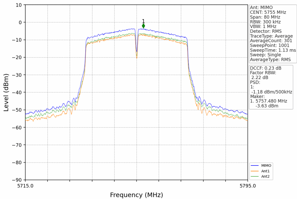
802.11ac(VHT40)_LCH_5755MHz_MIMO_NTNV
