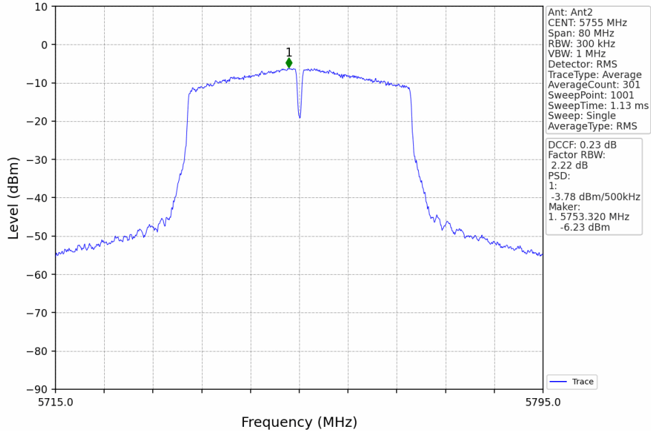
802.11ac(VHT40)_LCH_5755MHz_MIMO_NTNV
