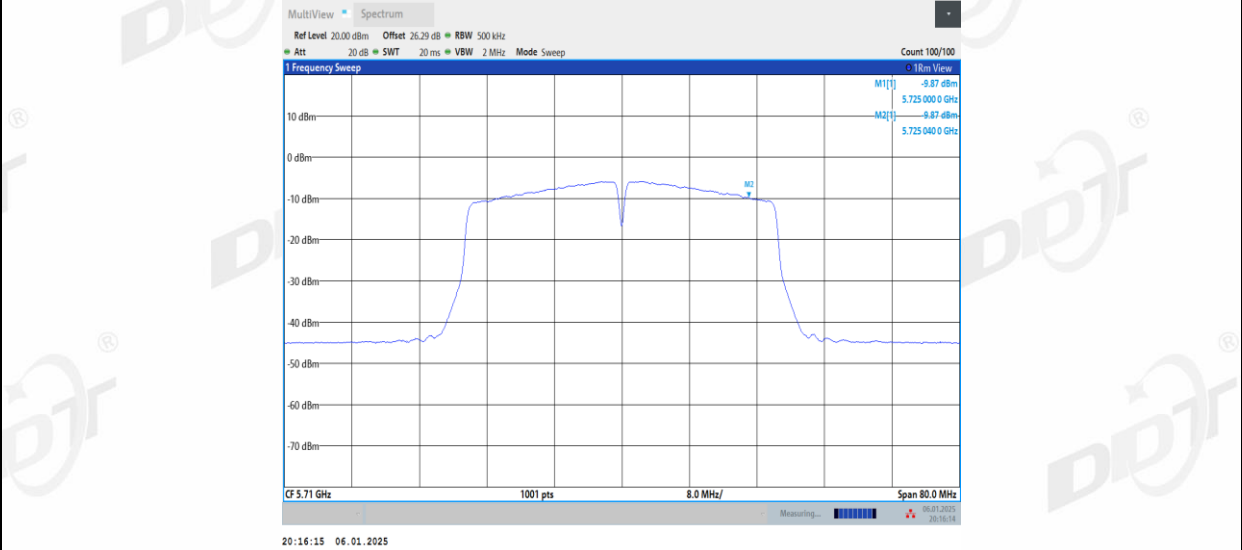
11AC40MIMO_Ant2_5710_UNII-3
