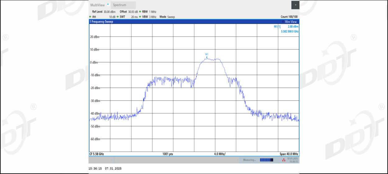
11AX20MIMO_Ant1_5580_52Tone_RU40
