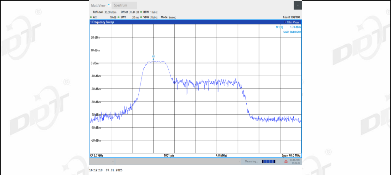
11AX20MIMO_Ant2_5700_52Tone_RU39
