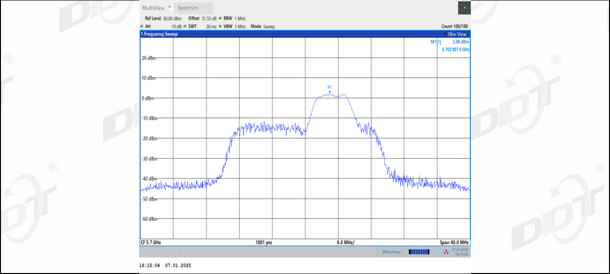
11AX20MIMO_Ant2_5700_52Tone_RU40
