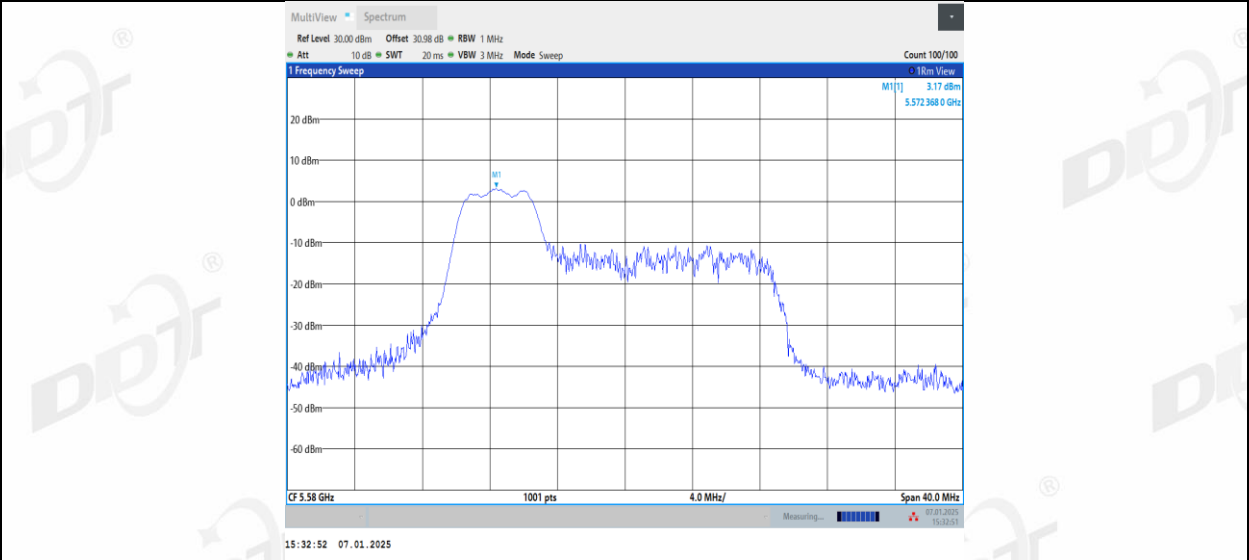
11AX20MIMO_Ant1_5580_52Tone_RU39
