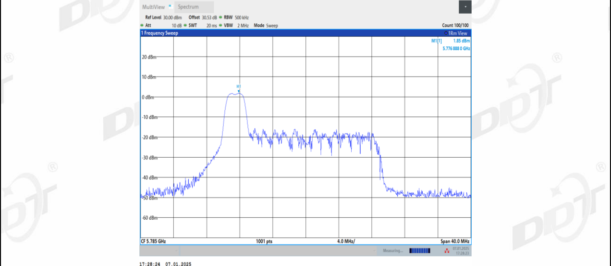
11AX20MIMO_Ant2_5785_26Tone_RU4
