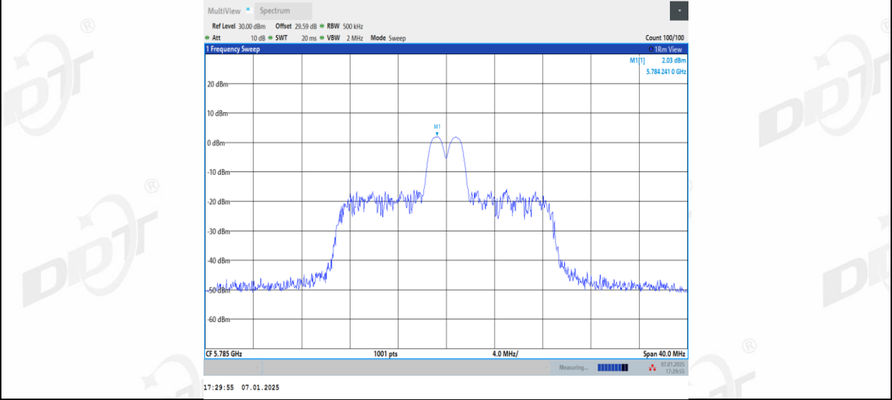
11AX20MIMO_Ant1_5785_26Tone_RU5
