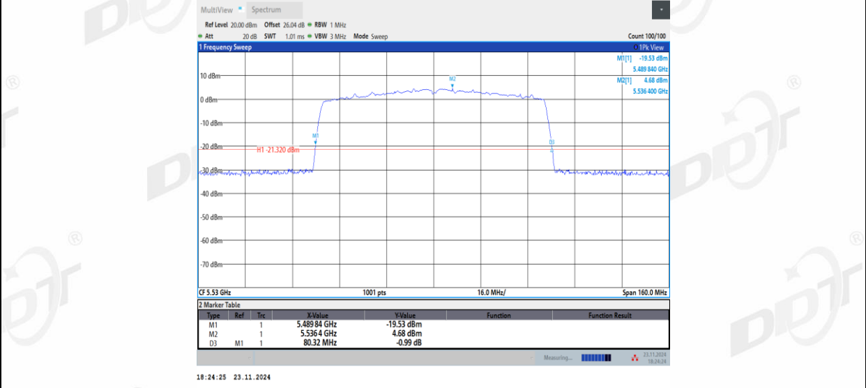
11AC80MIMO_Ant2_5530
