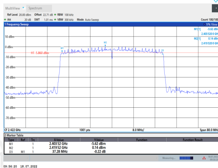
11AX40MIMO_Ant2_2422
