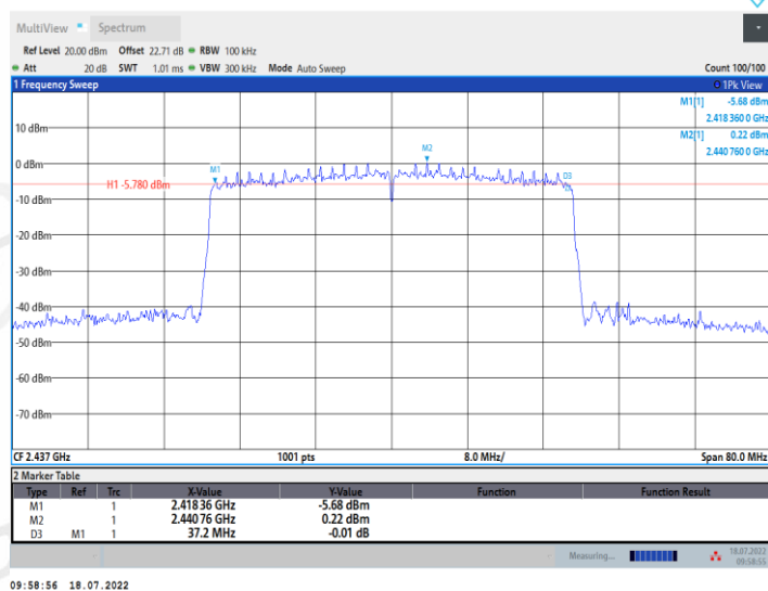
11AX40MIMO_Ant2_2437
