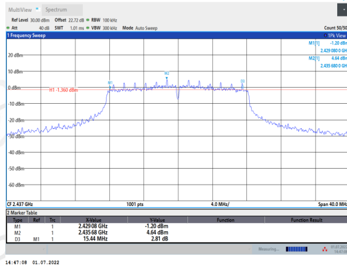
11G_Ant2_2437
