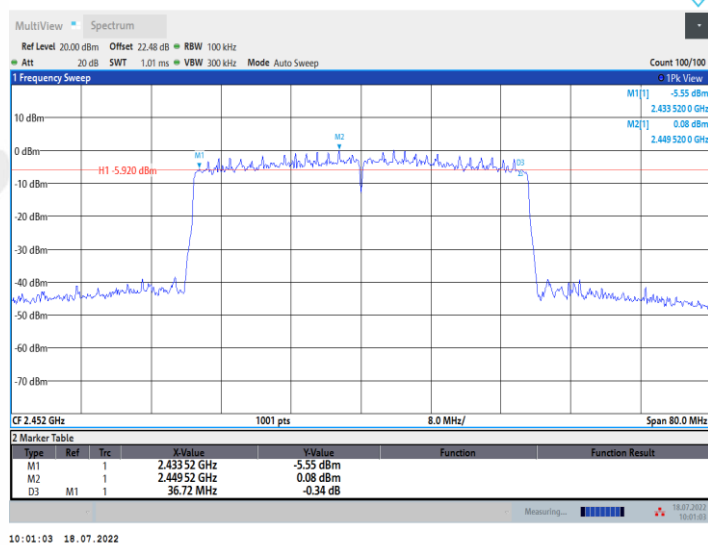
11AX40MIMO_Ant2_2452
