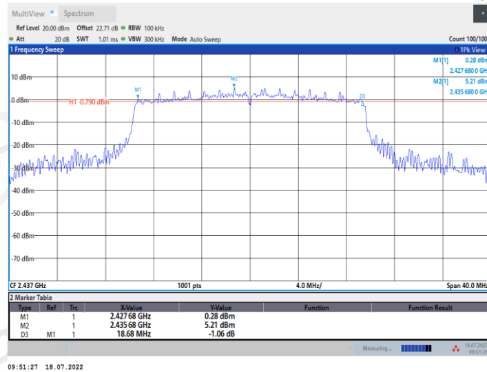
11AX20MIMO_Ant2_2437
