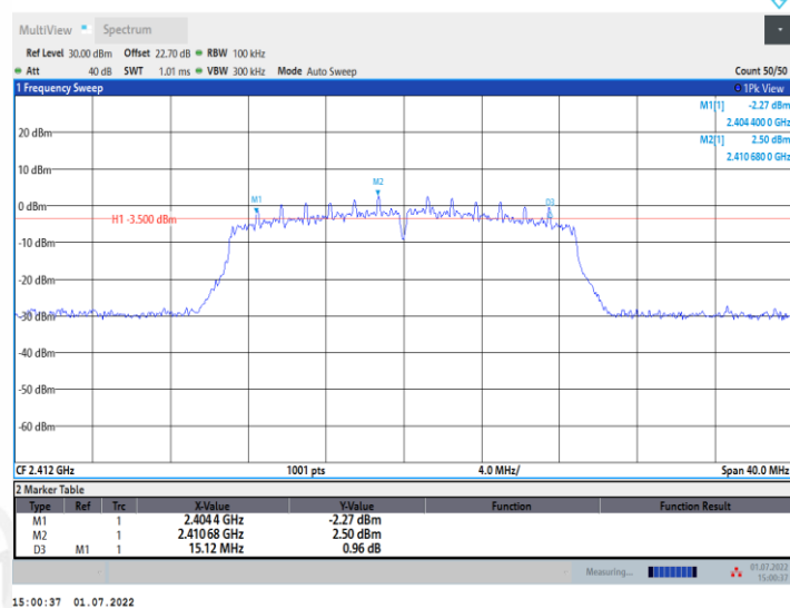
11N20MIMO_Ant2_2412
