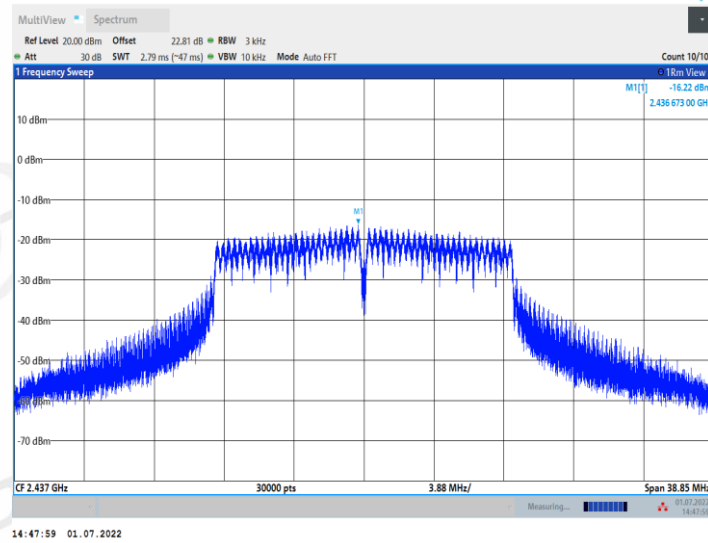
11G_Ant2_2437
