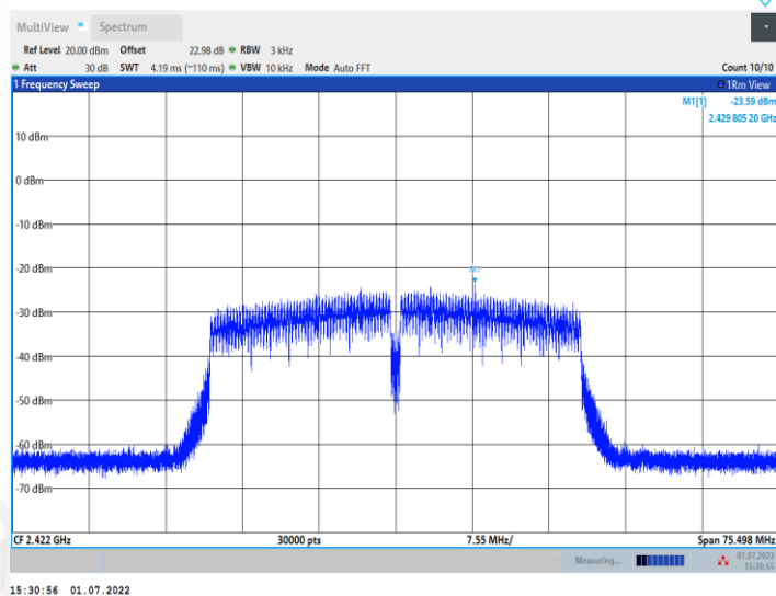
11N40MIMO_Ant2_2422
