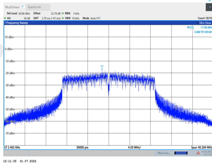
11N20MIMO_Ant2_2462
