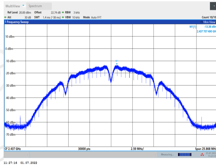
11B_Ant2_2437
