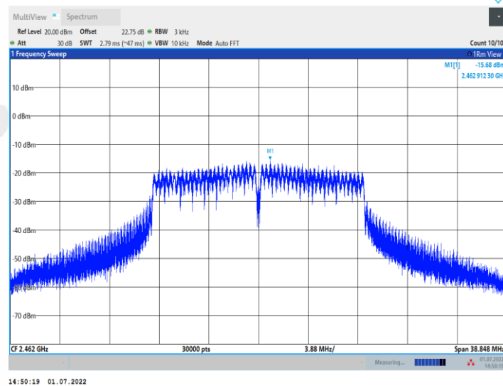
11G_Ant2_2462
