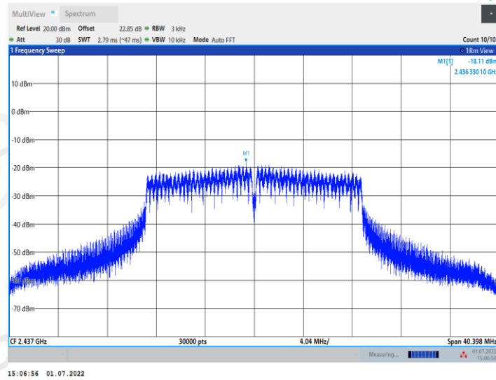
11N20MIMO_Ant2_2437
