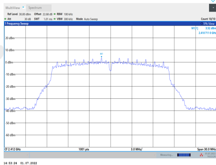
11G_Ant2_2412_30~1000
