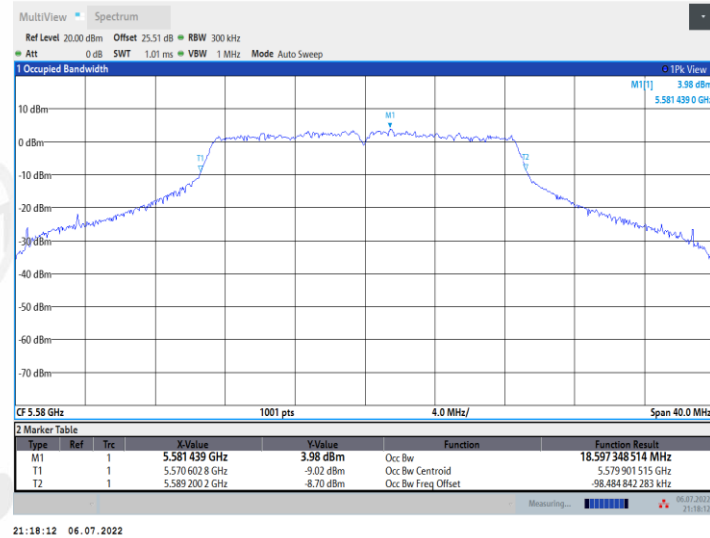
11N20MIMO Ant2 5580
