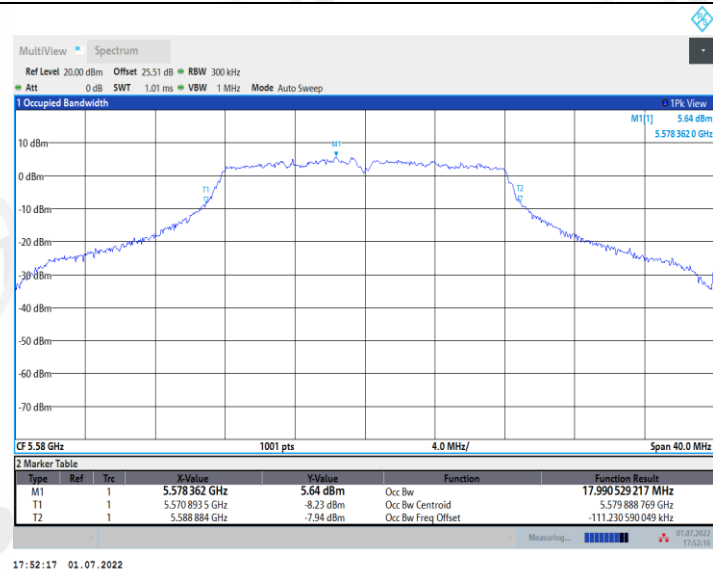
11A_Ant2_5580
