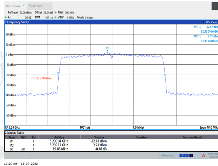
11AX20MIMO_Ant2_5240
