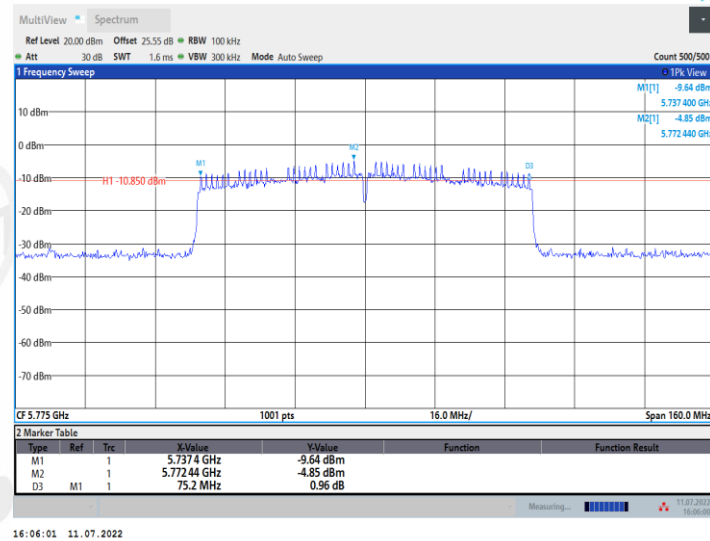
11AC80MIMO_Ant2_5775
