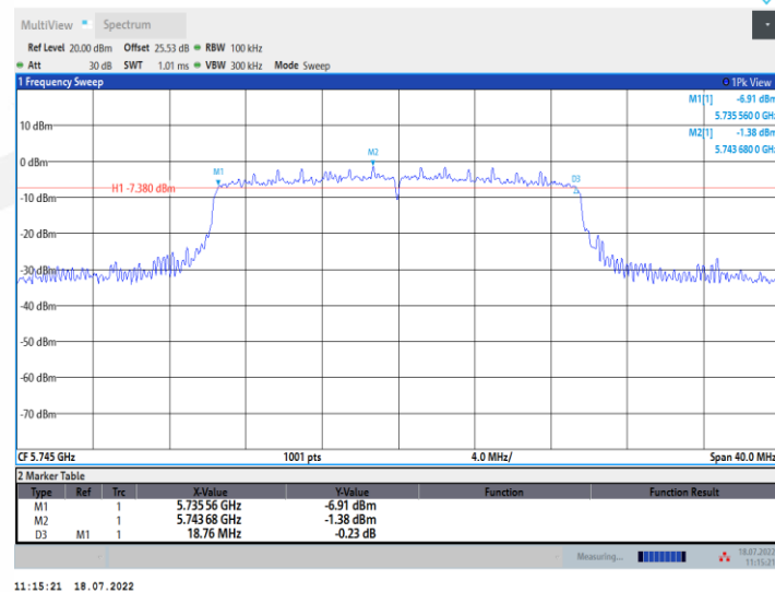
11AX20MIMO_Ant2_5745
