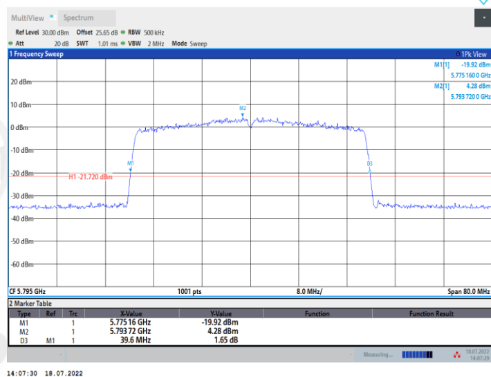
11AX40MIMO_Ant2_5795
