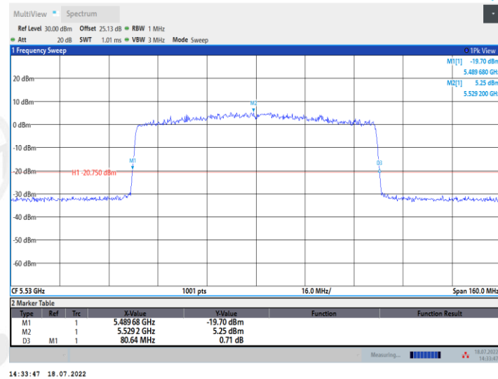
11AX80MIMO_Ant2_5530
