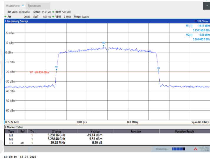
11AX40MIMO_Ant2_5270
