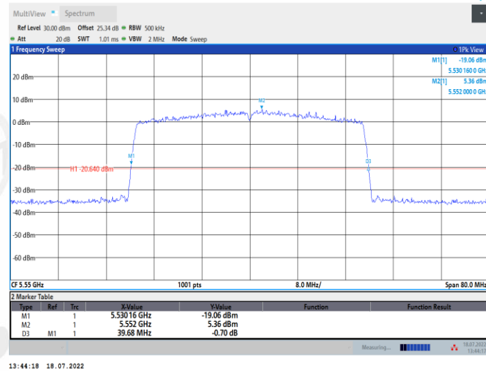
11AX40MIMO_Ant2_5550
