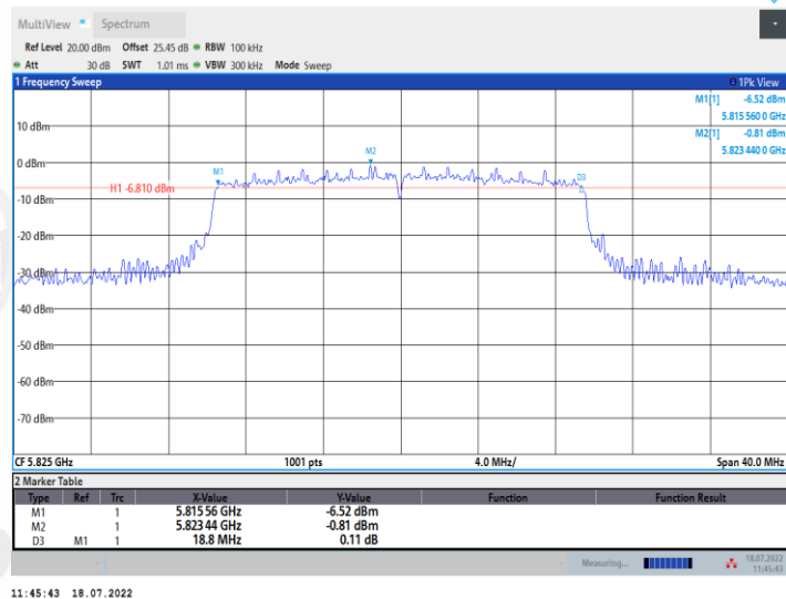
11AX20MIMO_Ant2_5825
